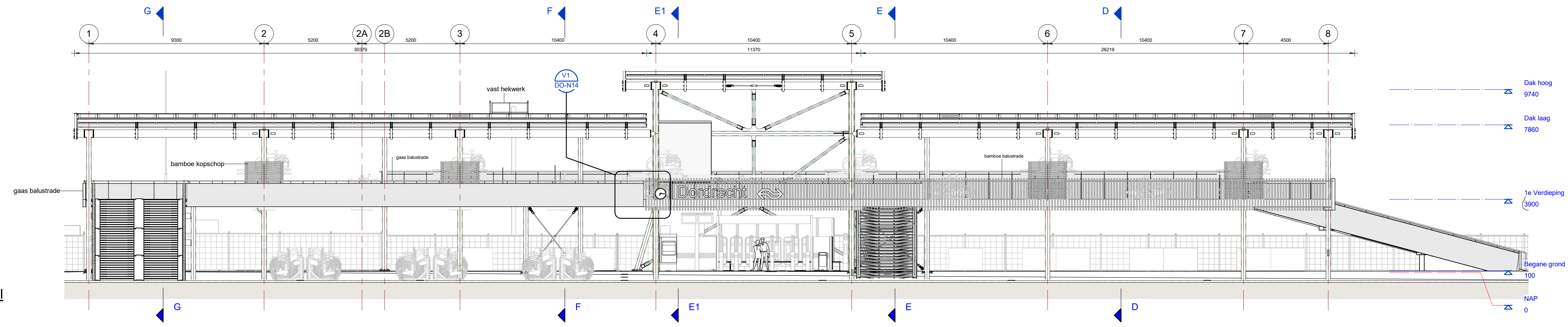
Zuid gevel schaal: 1 : 100
