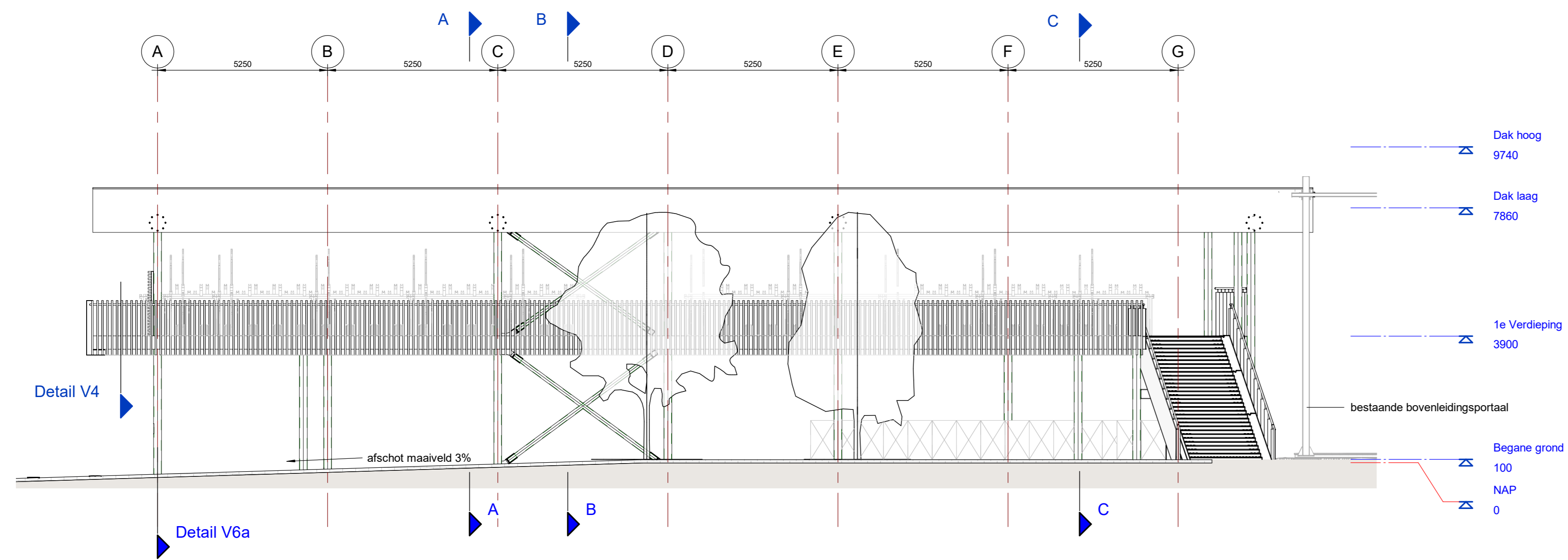
Oost gevel schaal: 1 : 100
