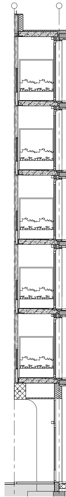
verticaal fragment parkgevel
