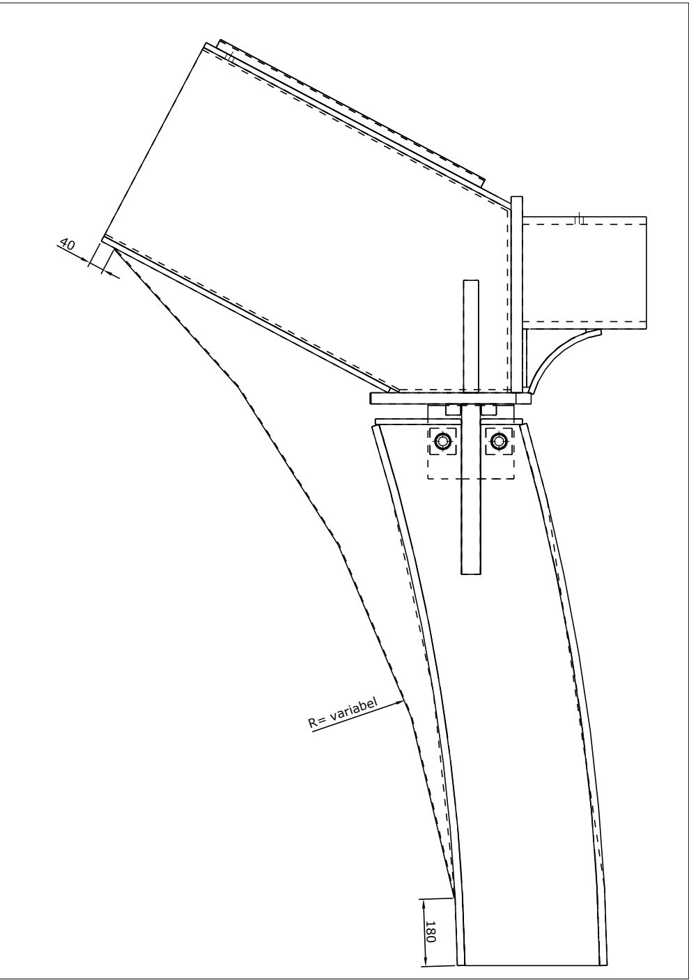
Detail beplating tpv overgang kolommen naar liggers
