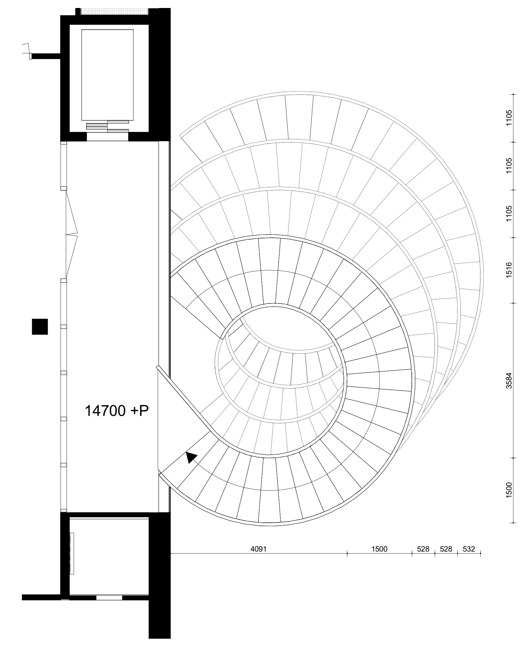
vierde verdieping
