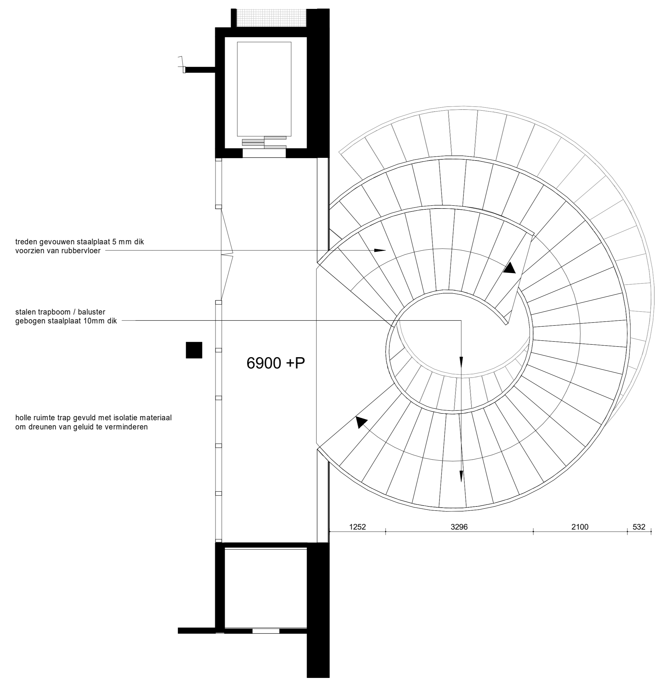
tweede verdieping
