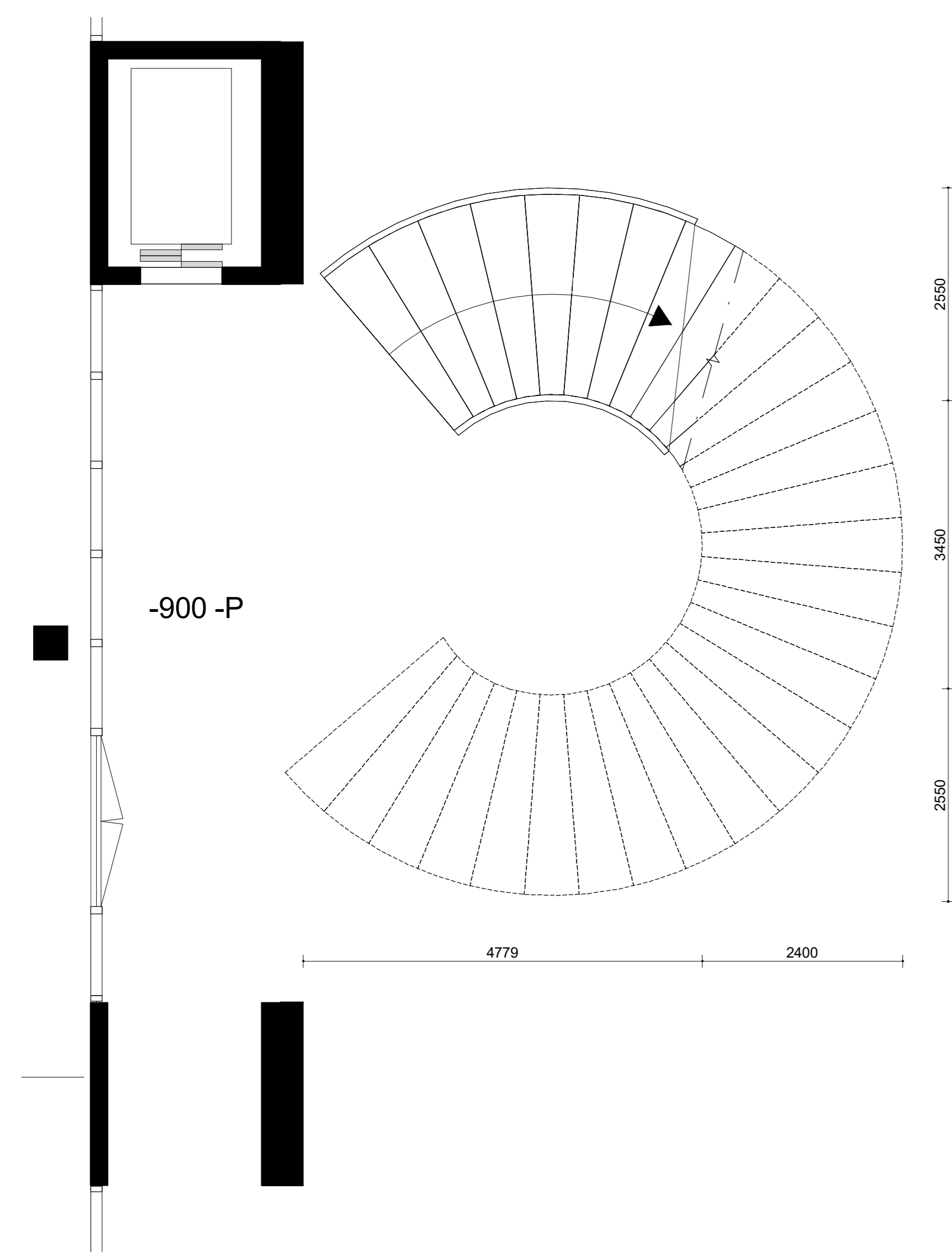
begane grond
