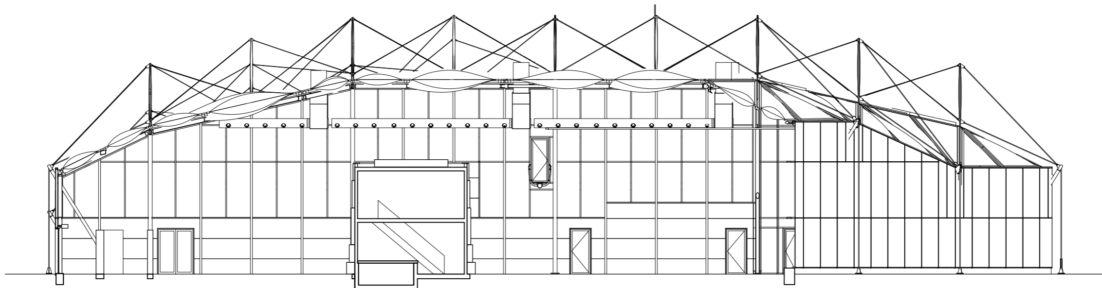
doorsnede A-A'
