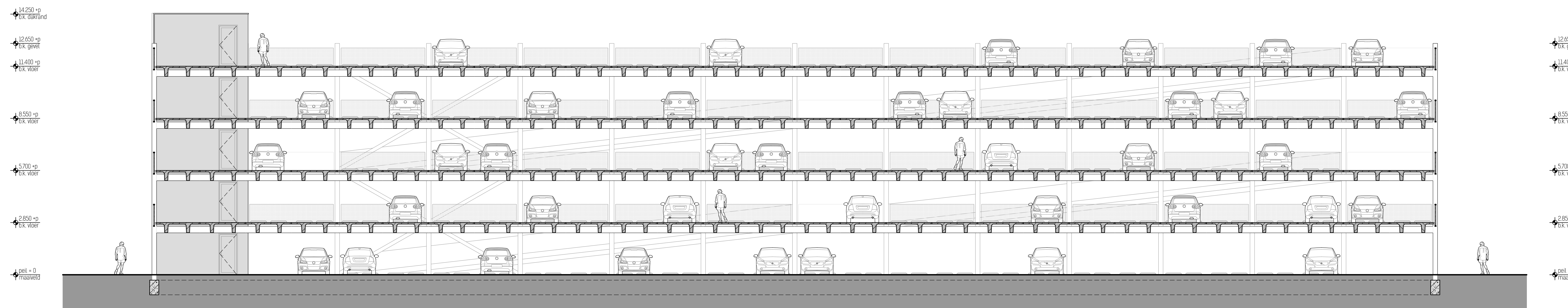
DOORSNEDE | LANGSDOORSNEDE A-A'
