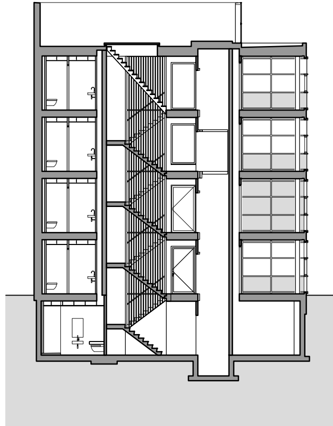
Langsdoorsnede kern
