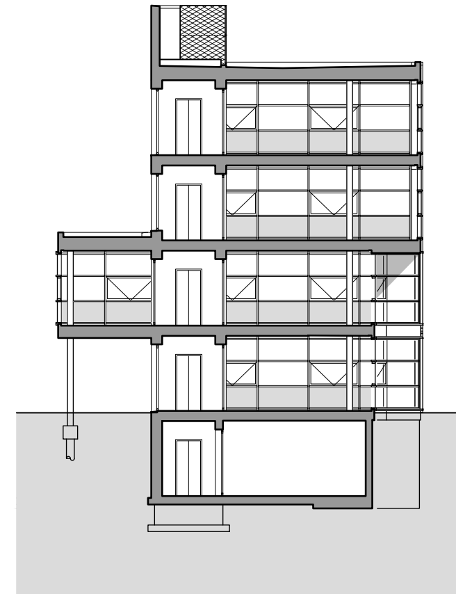
Dwarsdoorsnede entree / hal
