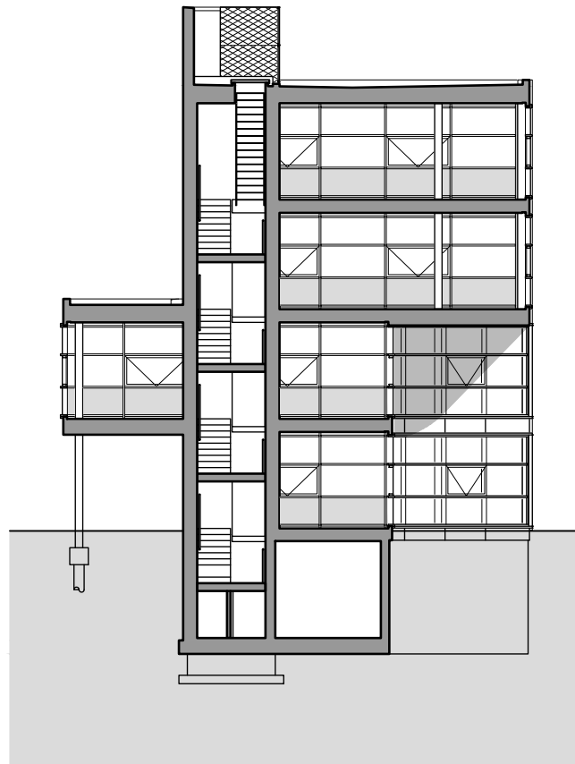
Dwarsdoorsnede trappenhuis
