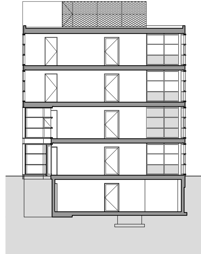
Langsdoorsnede verdieping
