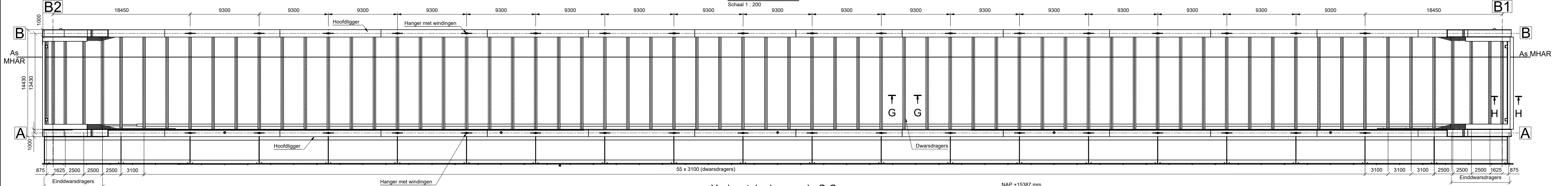
Horizontale doorsnede C-C Schaal 1 : 200
