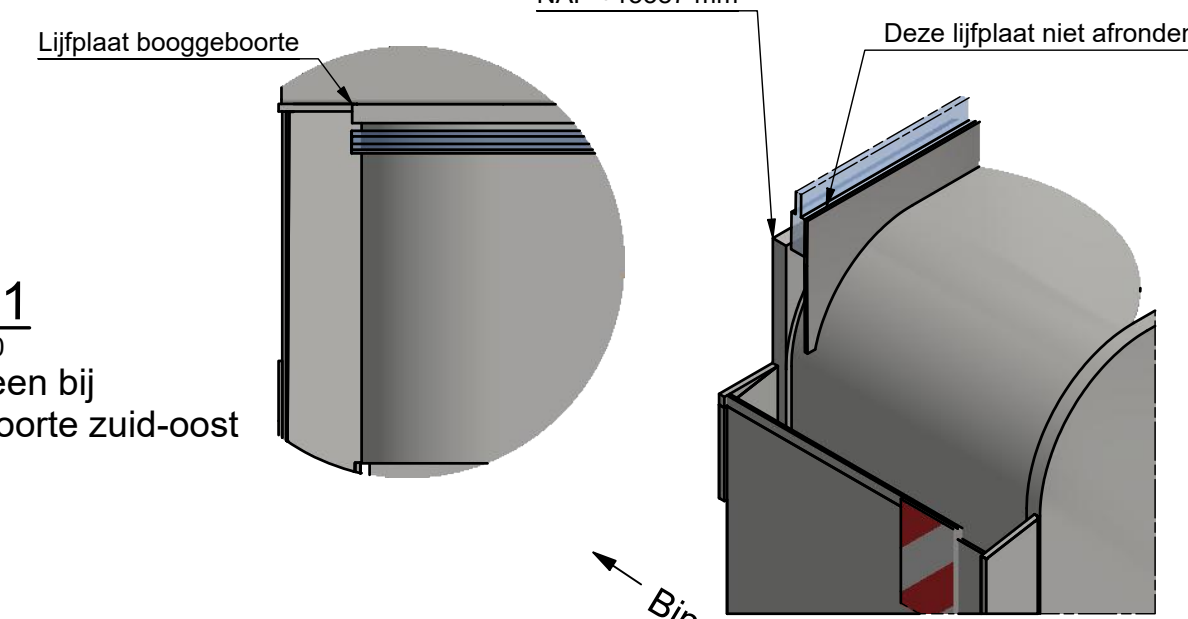
Isometrisch aanzicht Schaal 1 : 20
