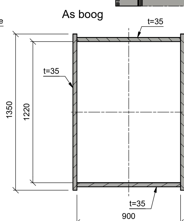
Doorsnede F-F Schaal 1 : 20
