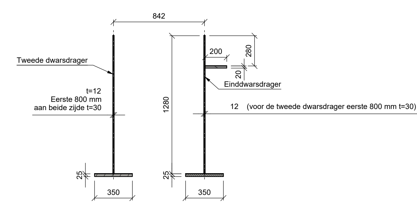
Doorsnede H-H Schaal 1 : 20
