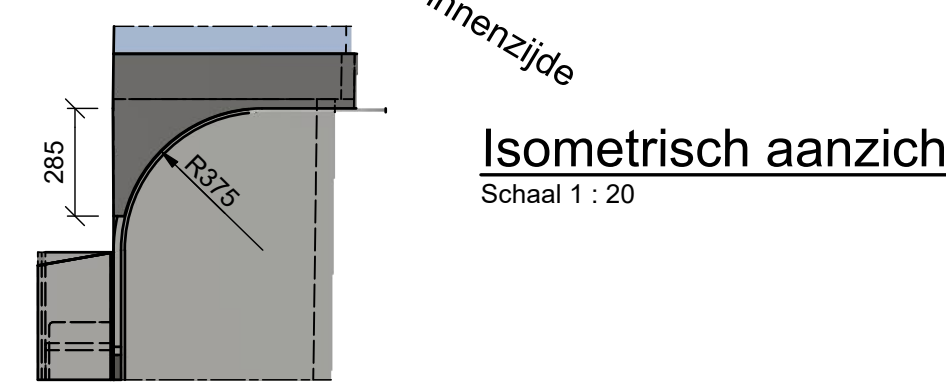
Zijaanzicht Schaal 1 : 20
