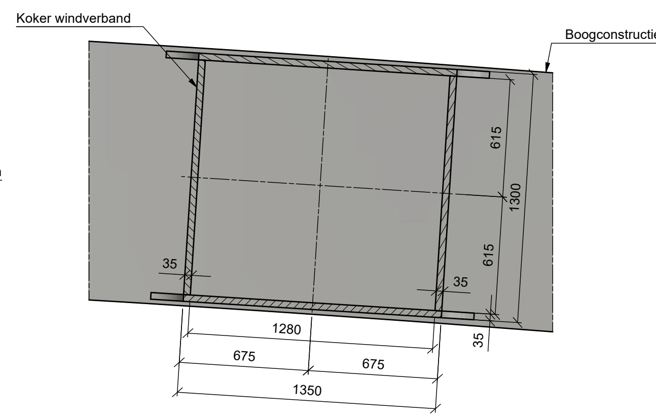
Doorsnede E-E Schaal 1 : 20
