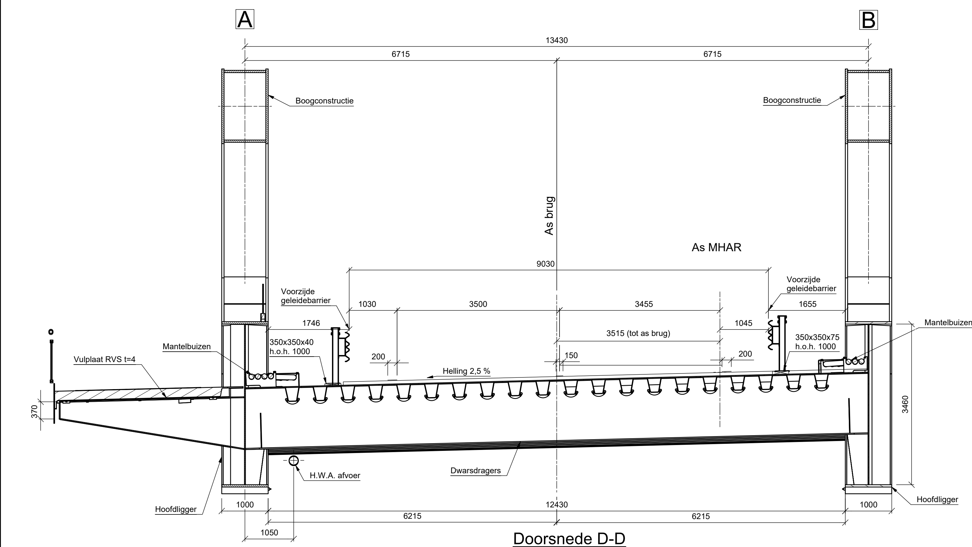
Doorsnede D-D Schaal 1 : 50
