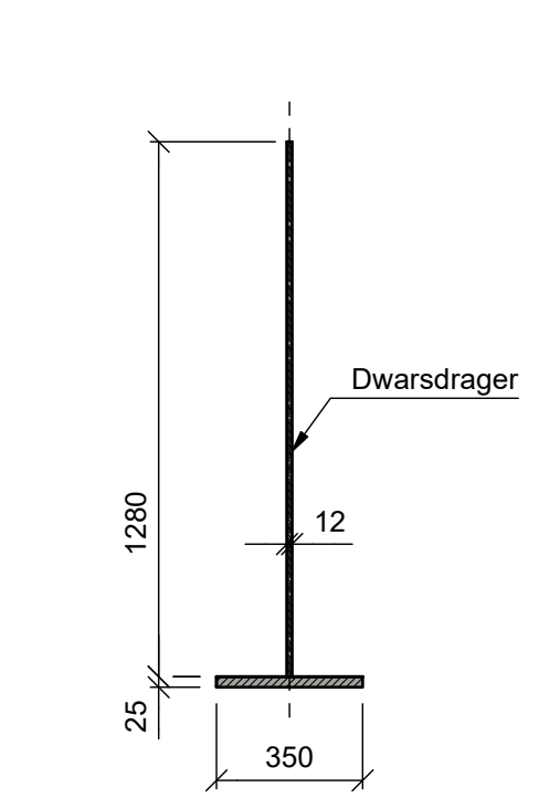
Doorsnede G-G Schaal 1 : 20
