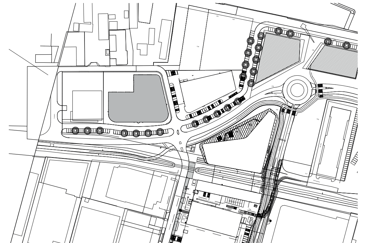
Situatietekening
