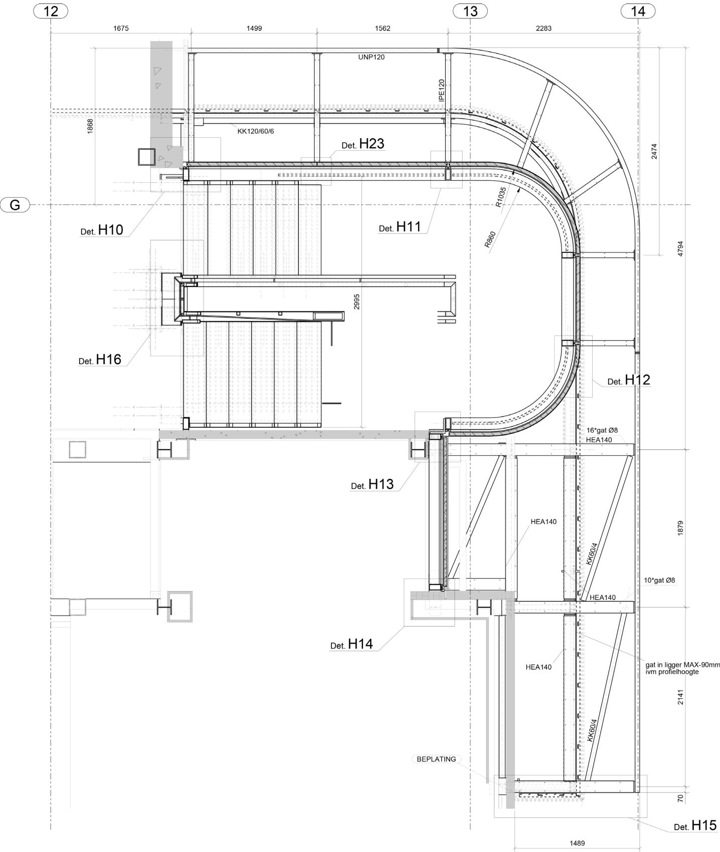
Plattegrond trappenhuis
