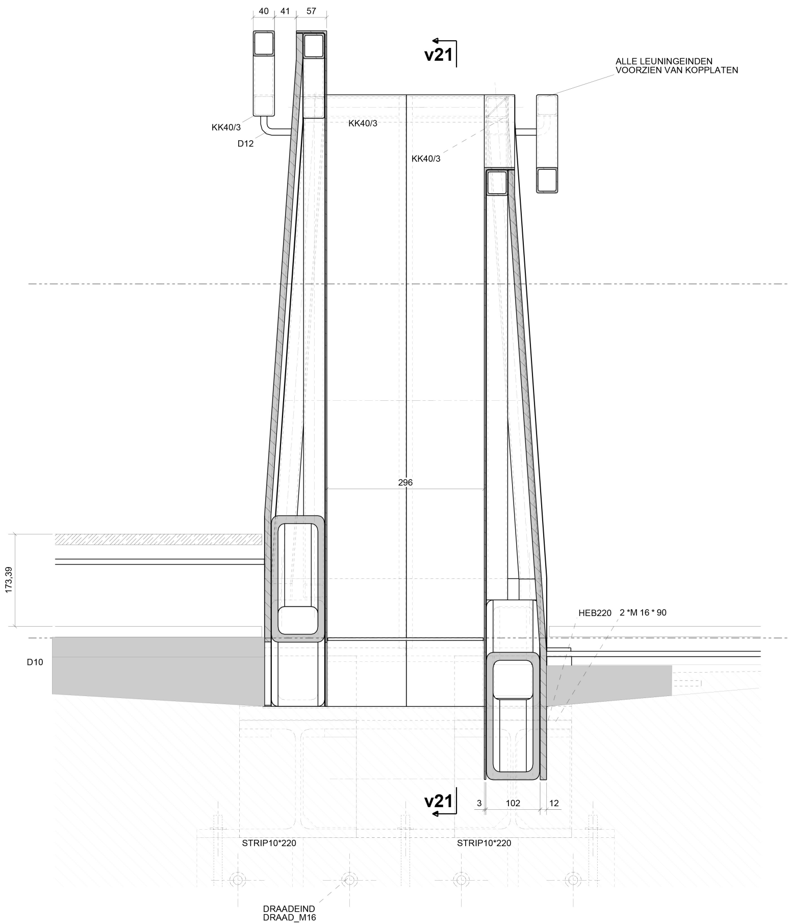
Detail dragende trapboom met uitkragende treden
