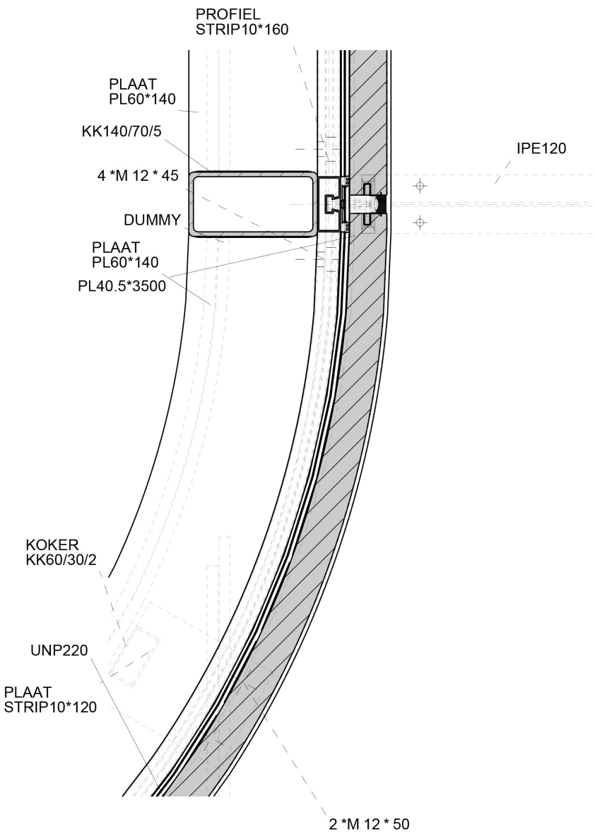
Detail structurele glas gevel met 'on steel' montage
