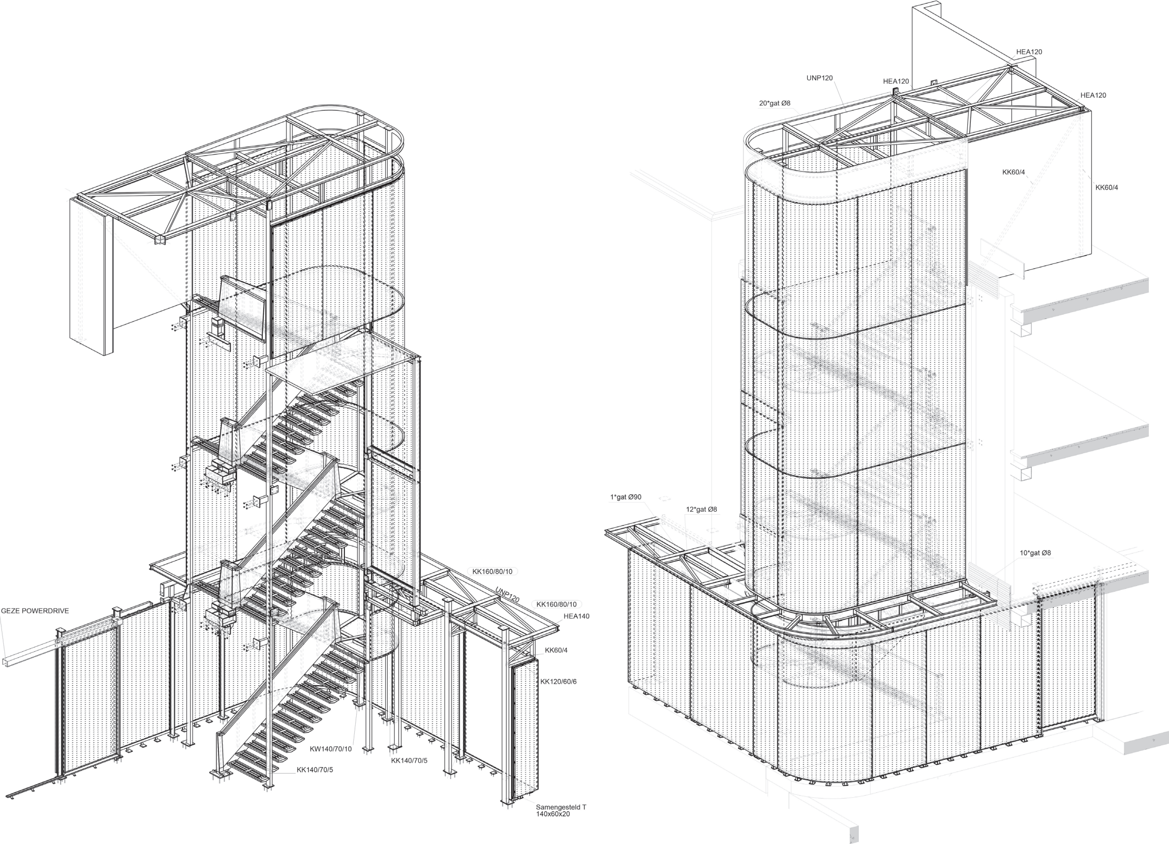
3D staalconstructie
