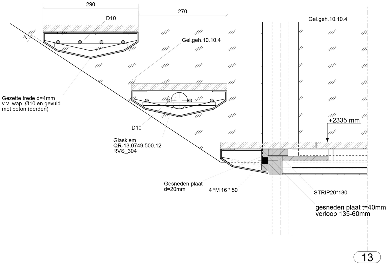
Detail doorsnede traptrede
