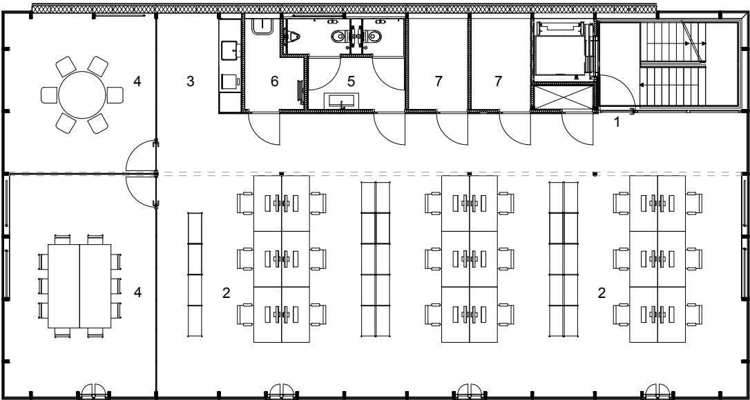
2e verdieping
