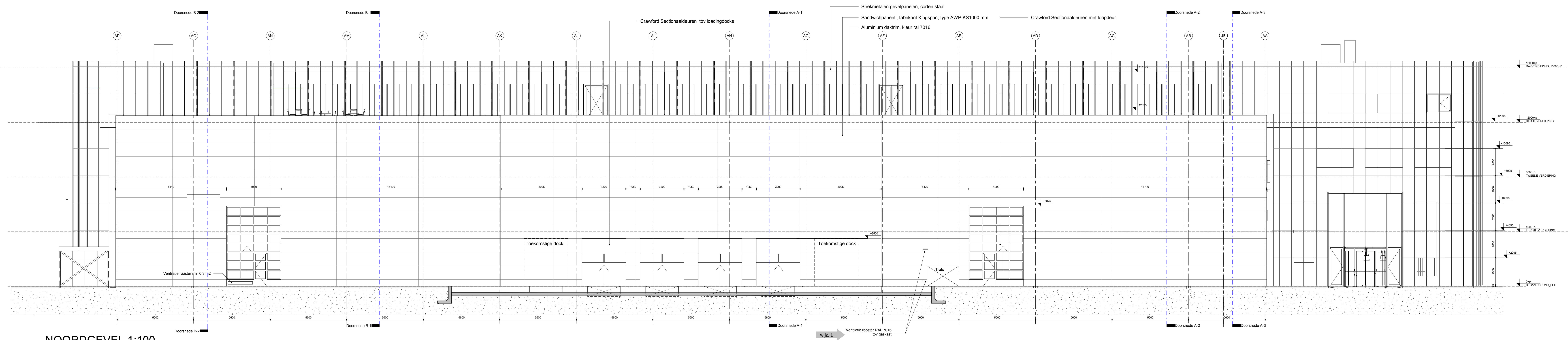
NOORDGEVEL 1:100
