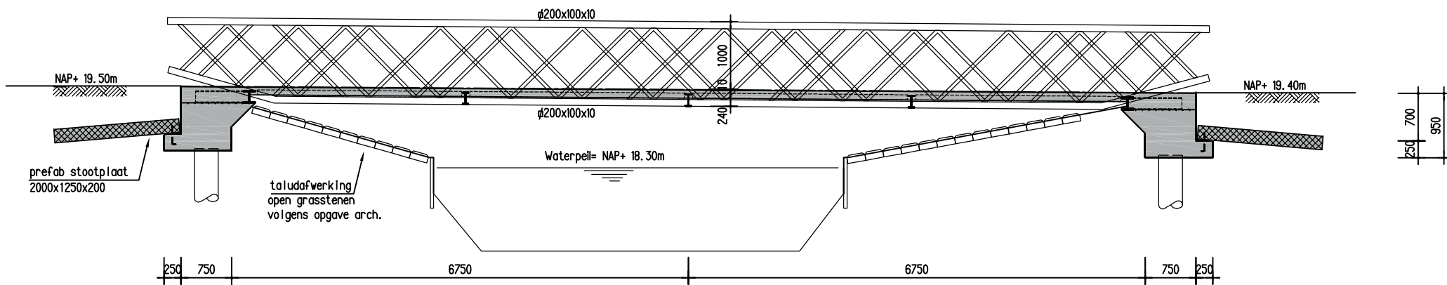
Doorsnede
