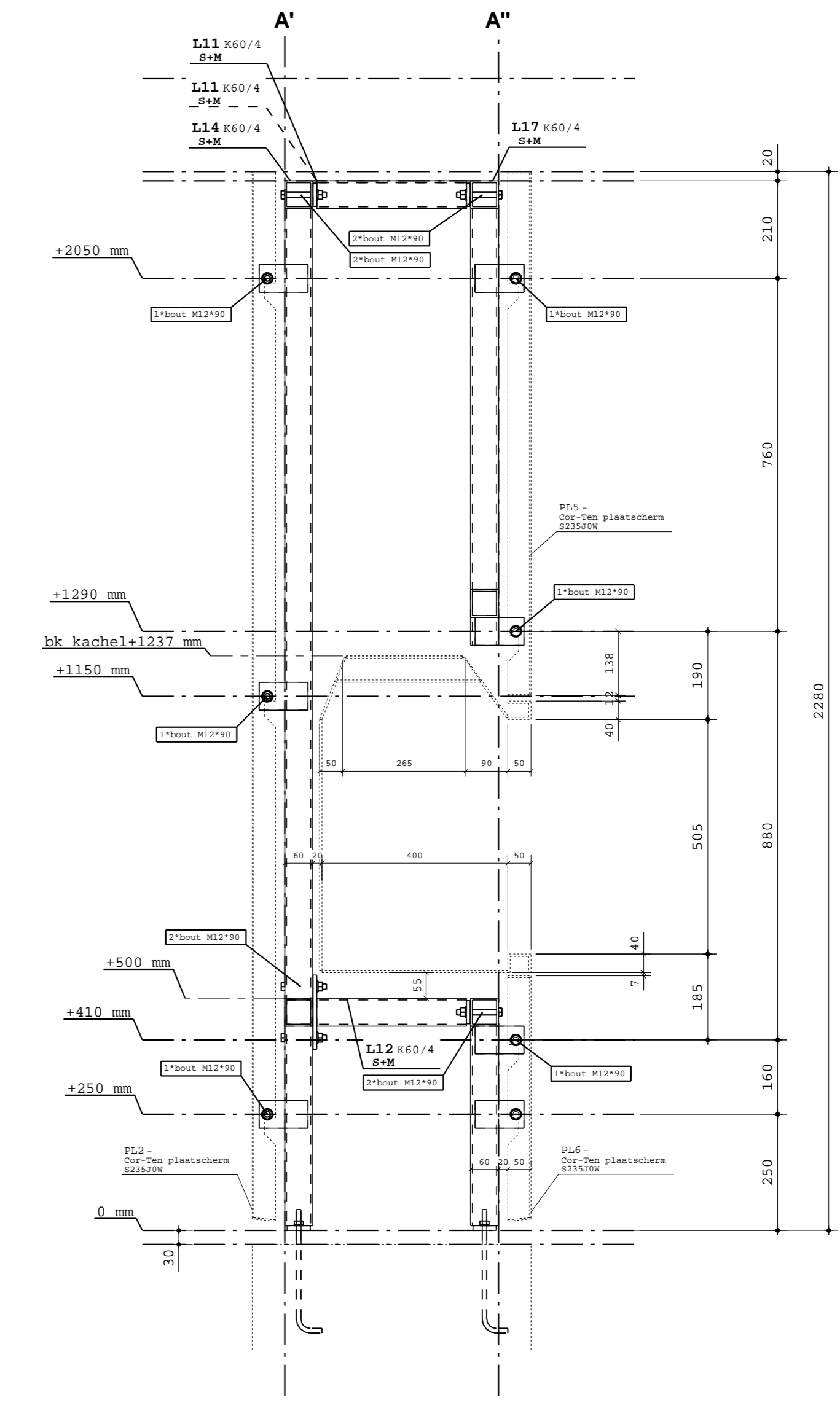
dsn D - D, 1:10
