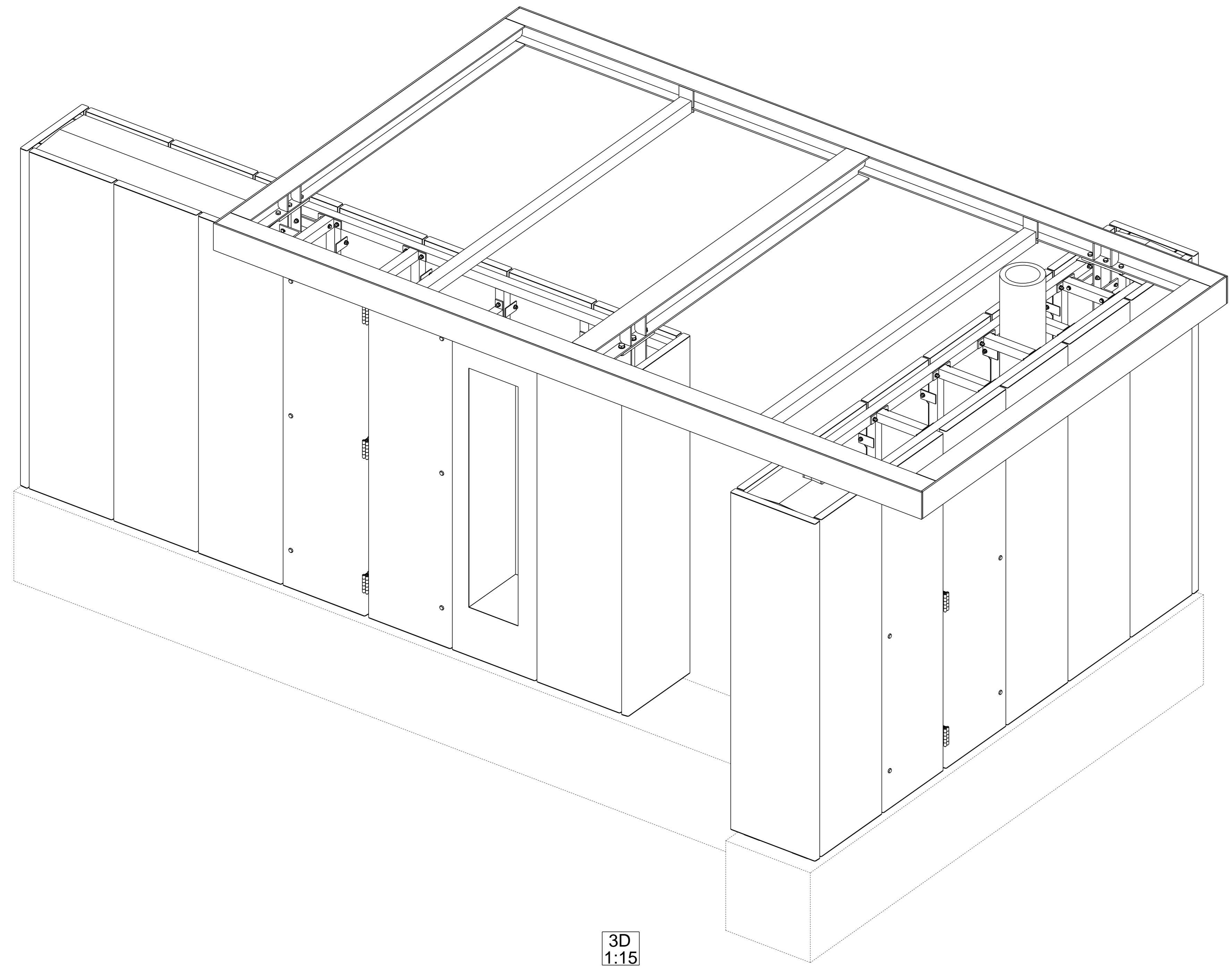
3D (zonder panelen) 1:15
