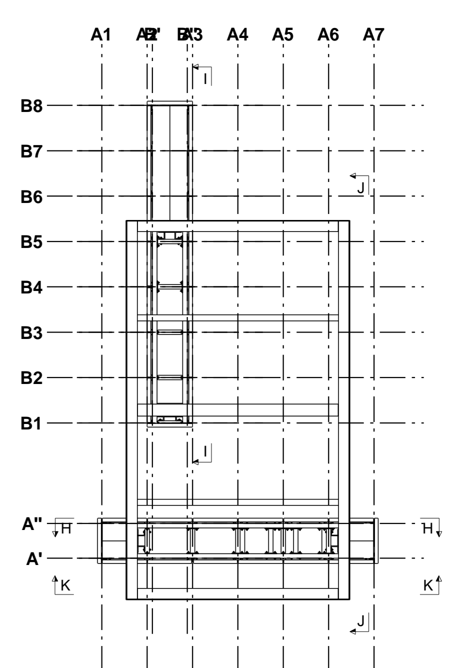
Bovenaanzicht op 2480+ 1:50
