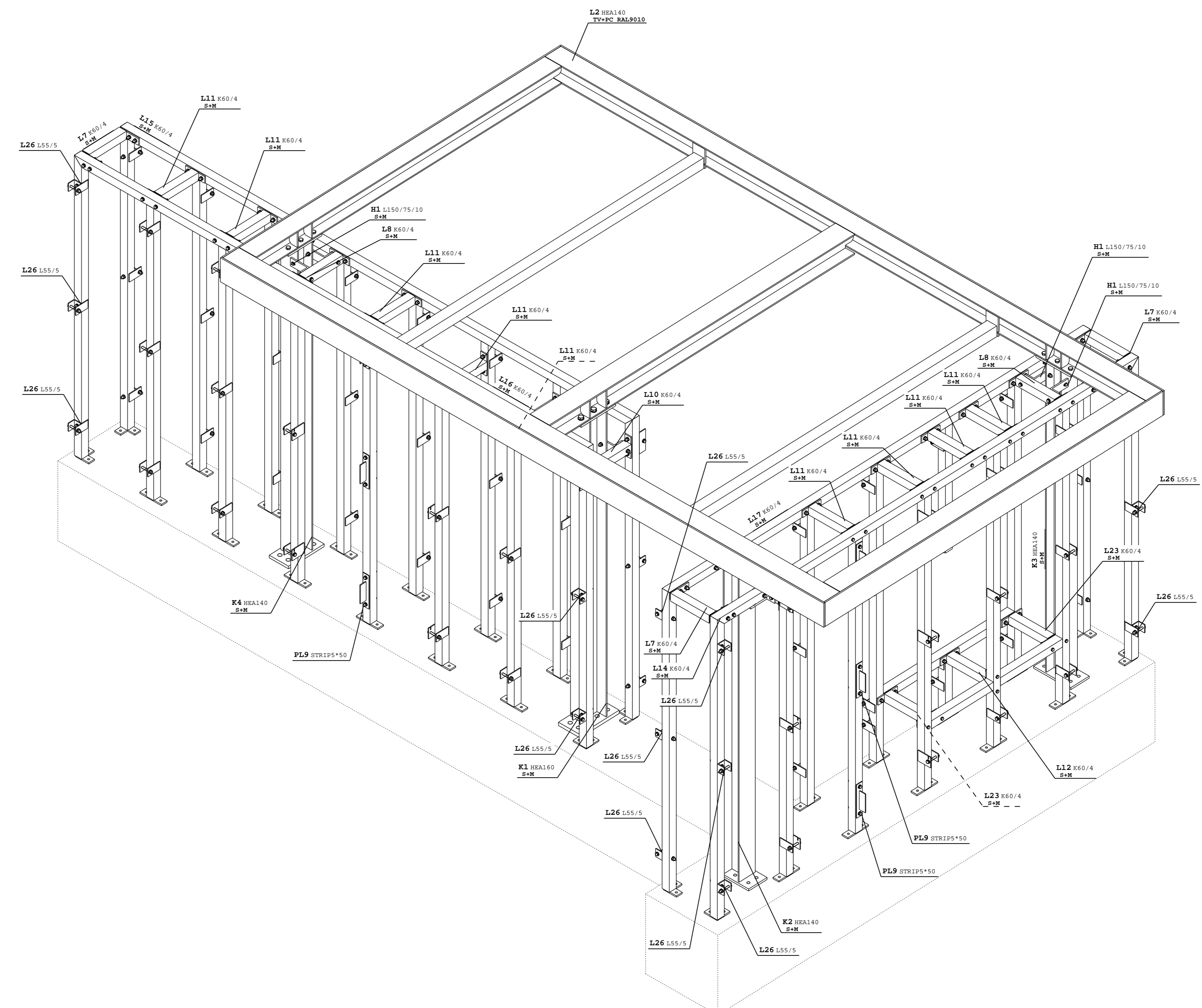
3D (zonder panelen) 1:15
