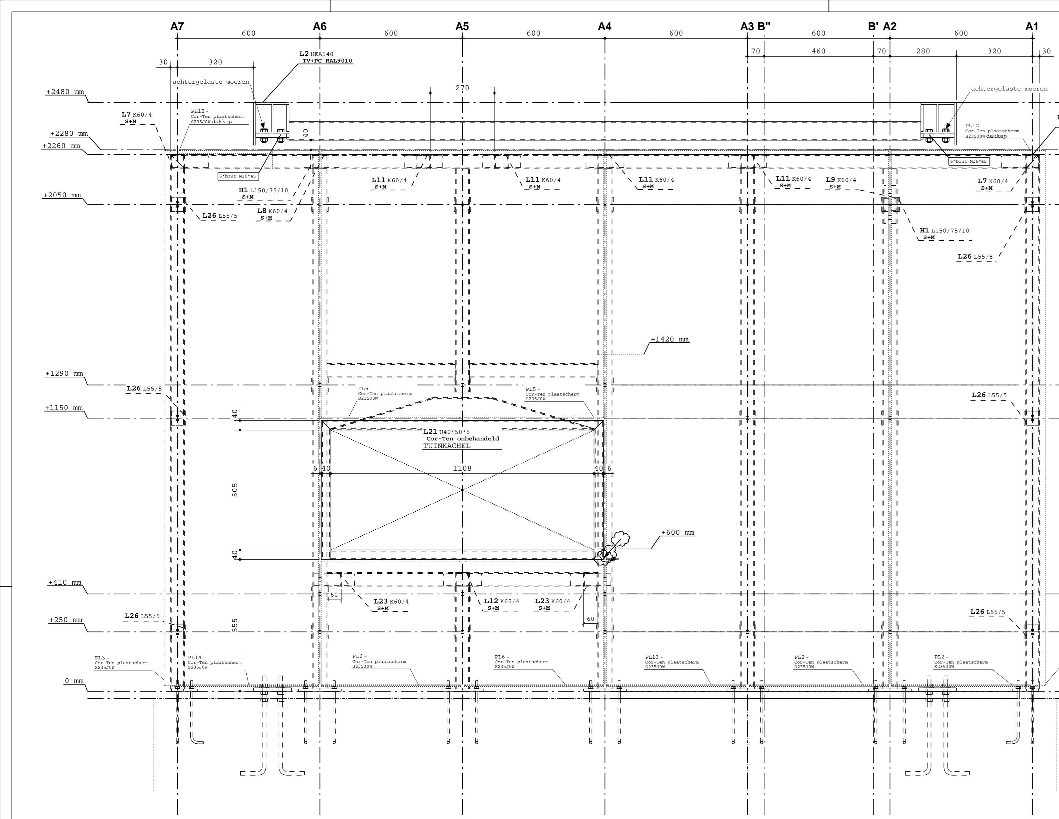
dsn H-H, 1:10
