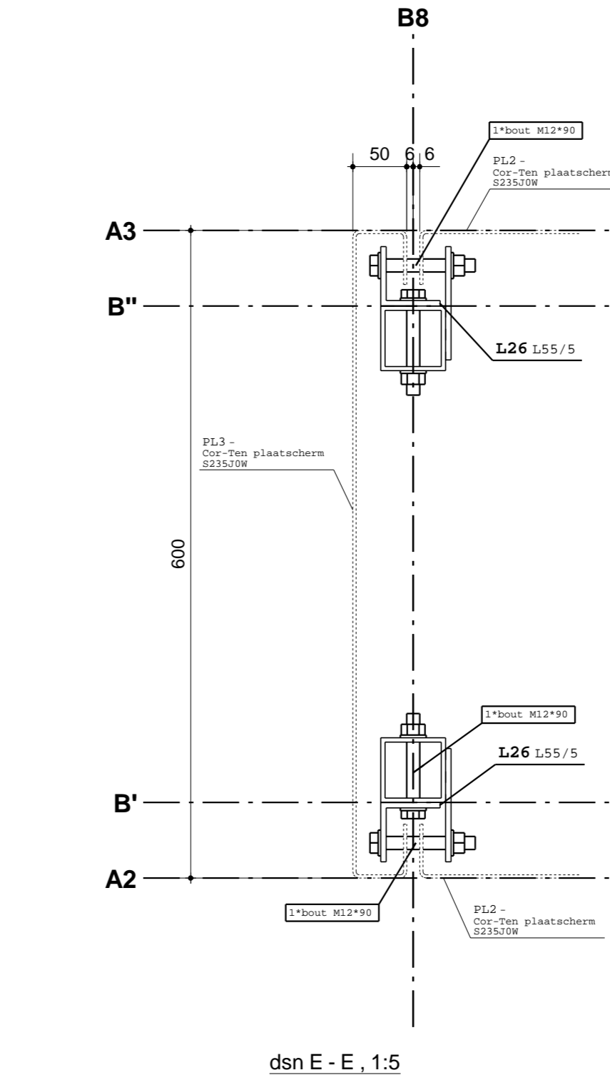
dsn E - E, 1:5
