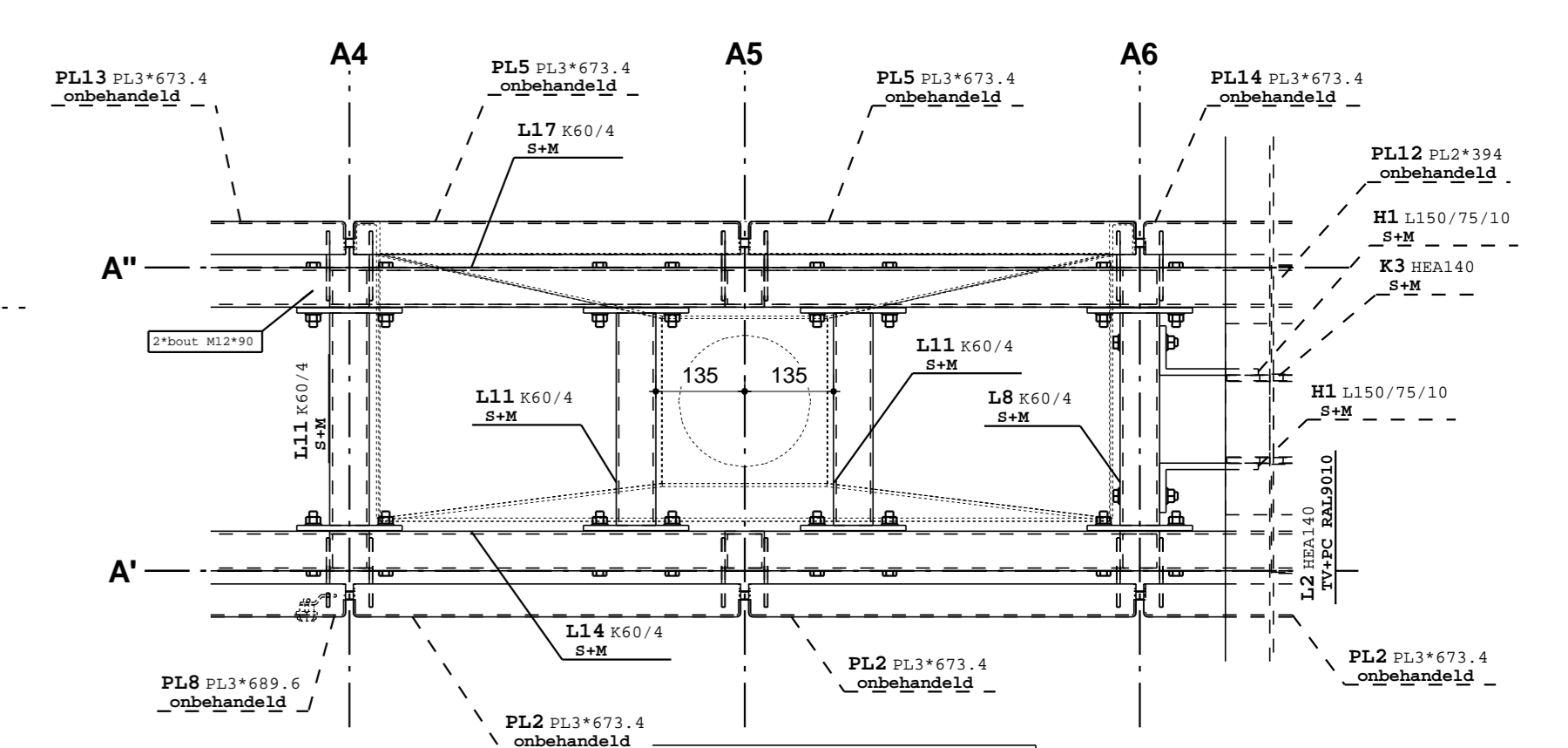
Bovenaanzicht op 1150+ 1:10
