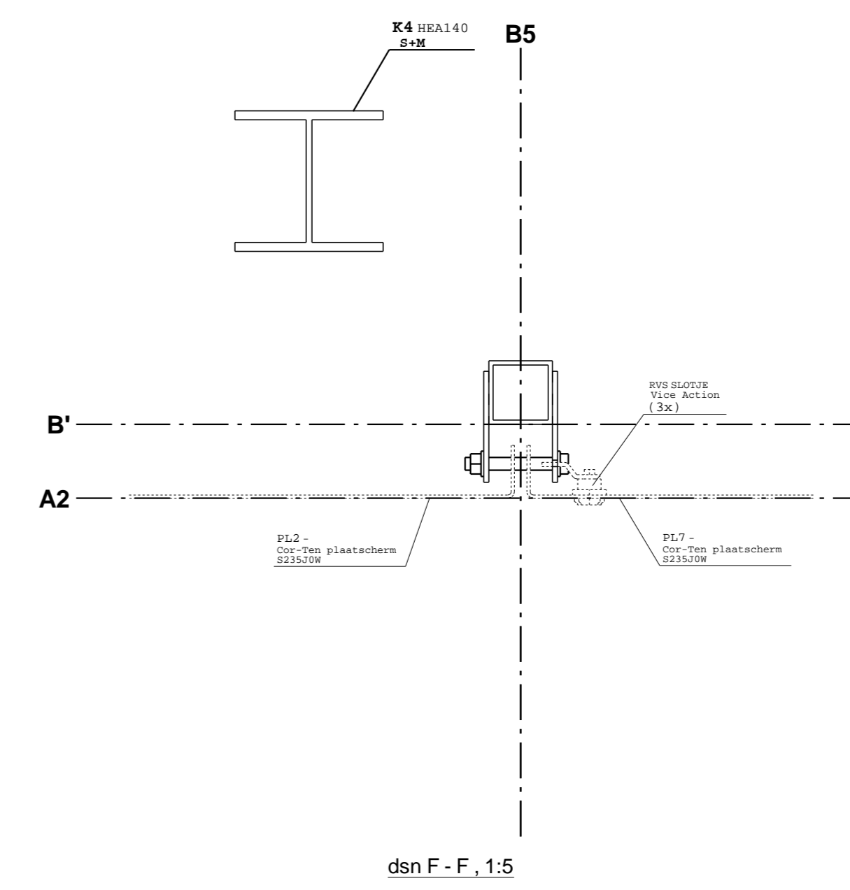
dsn F - F, 1:5
