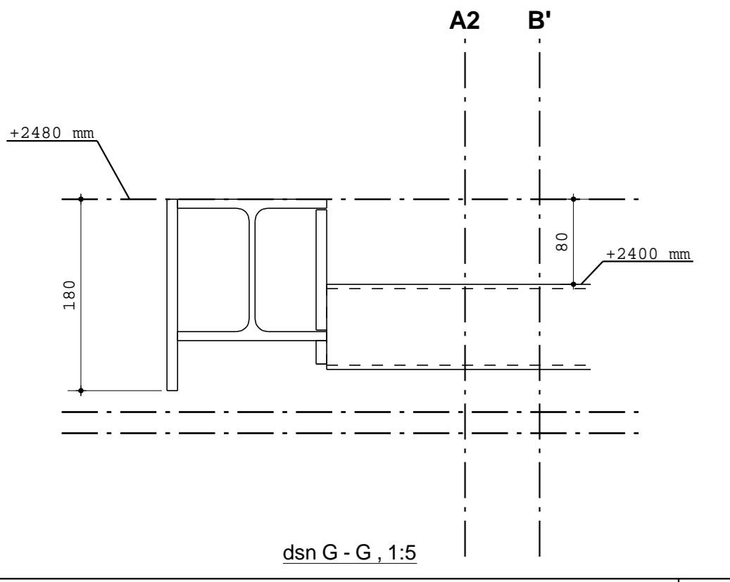
dsn G - G, 1:5
