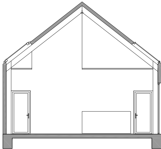
DOORSNEDE A-A
