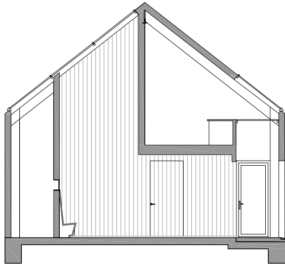
DOORSNEDE B-B
