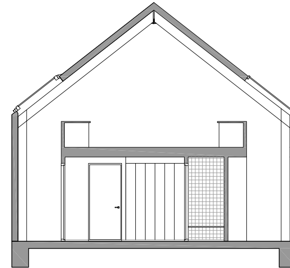
DOORSNEDE C-C
