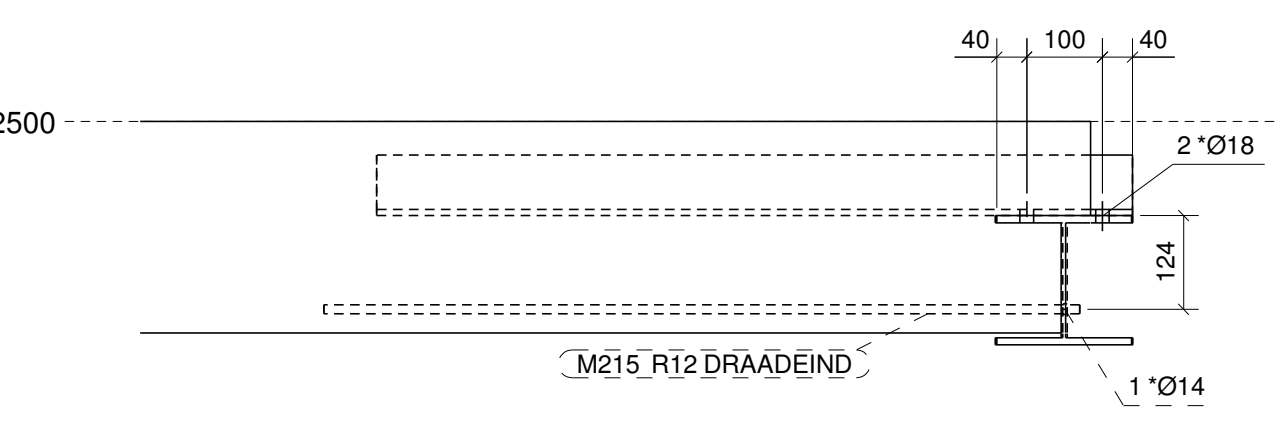
dsn K - K, 1:10
