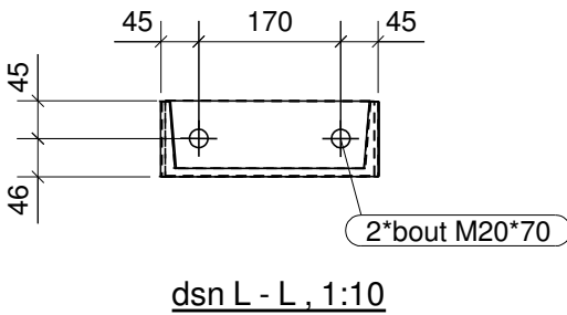
dsn L - L, 1:10
