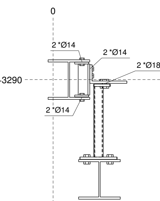
dsn I - I, 1:10
