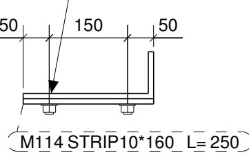
dsn F - F, 1:10
