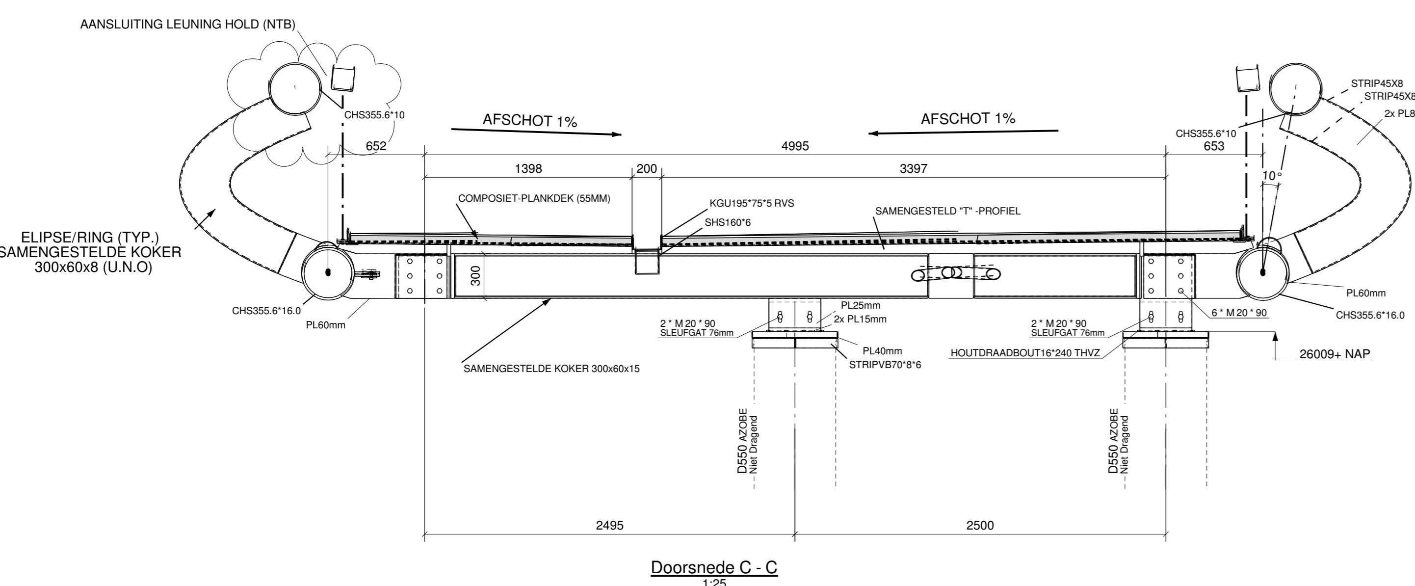
Doorsnede C - C 1:25
