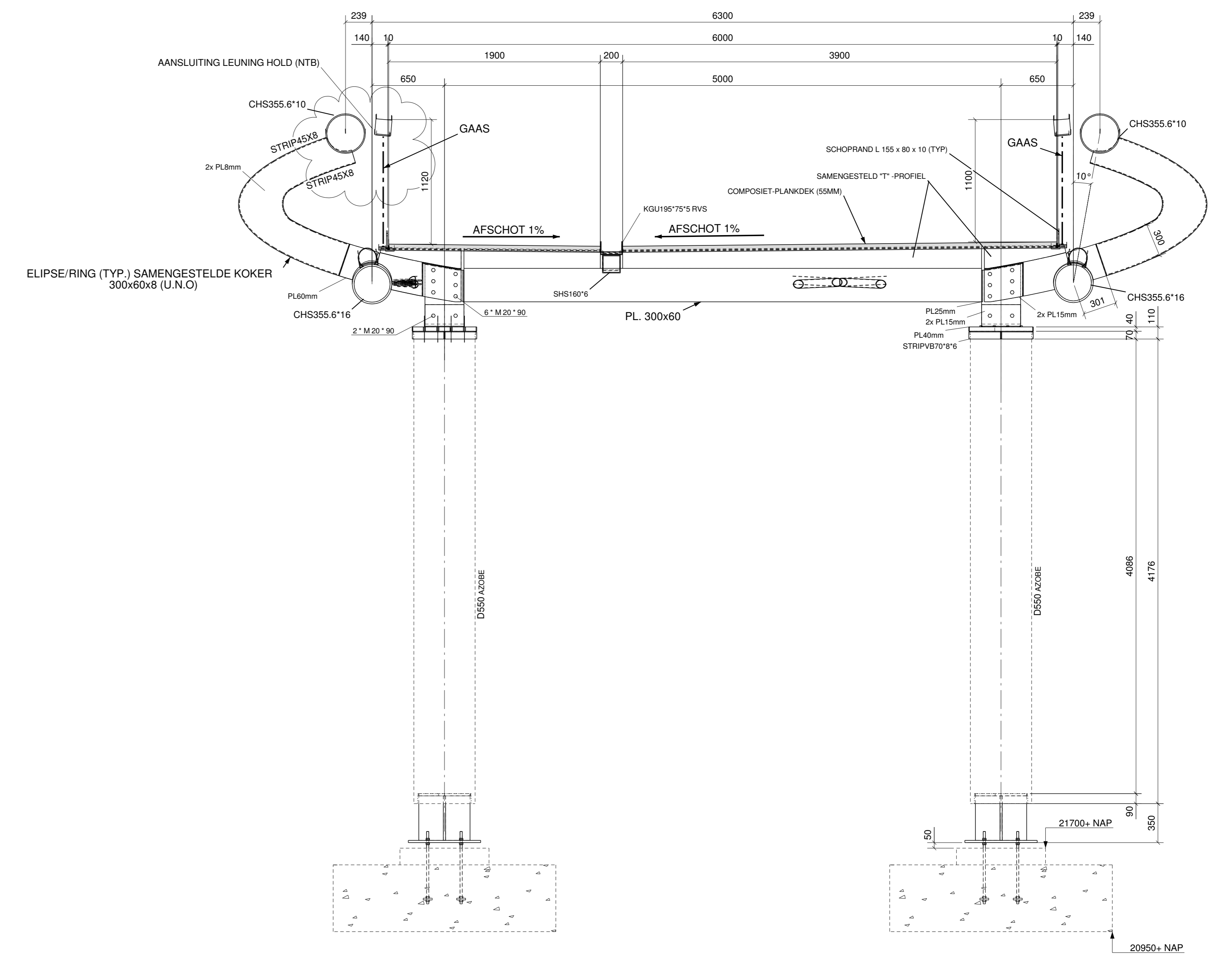
Doorsnede A - A 1:25
