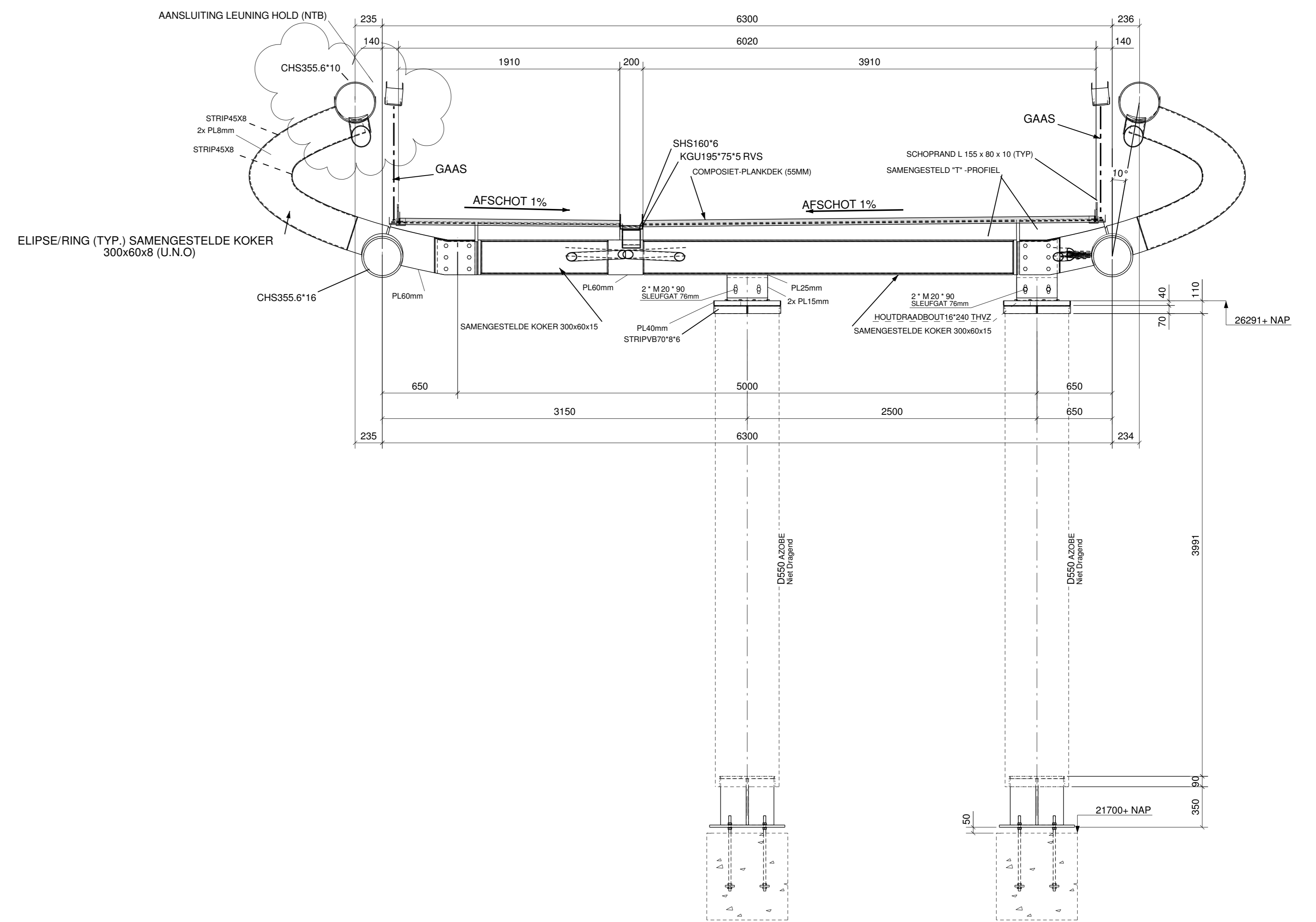
Doorsnede B - B 1:25
