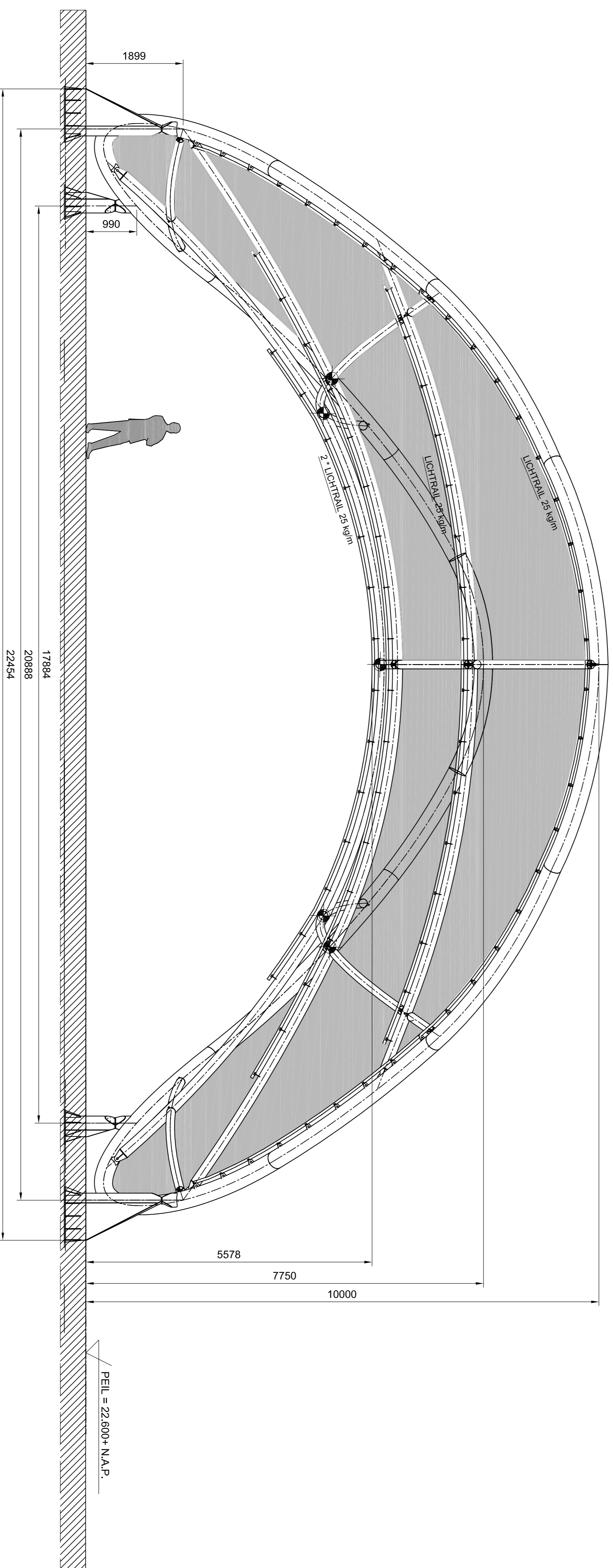
VOORAANZICHT [1:50]
