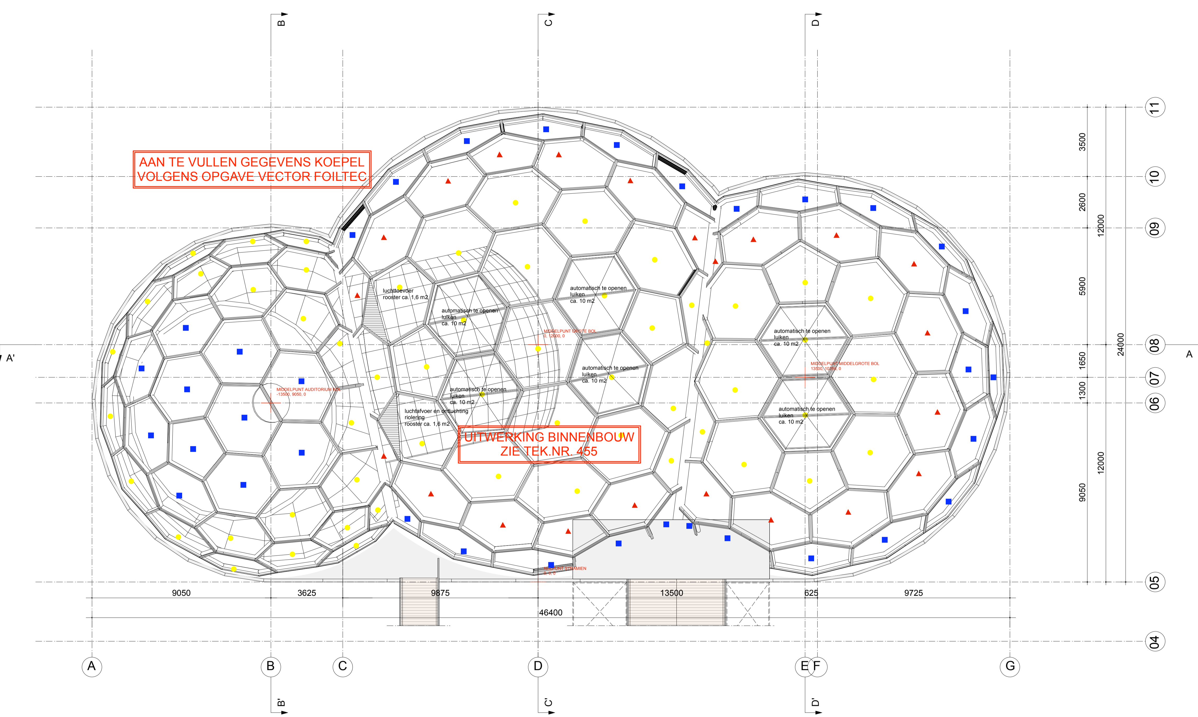
Dakaanzicht drijvend paviljoen schaal 1:100
