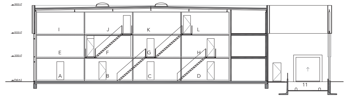
doorsnede A-A
