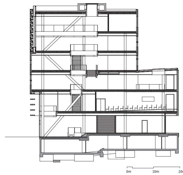
Doorsnede BB
