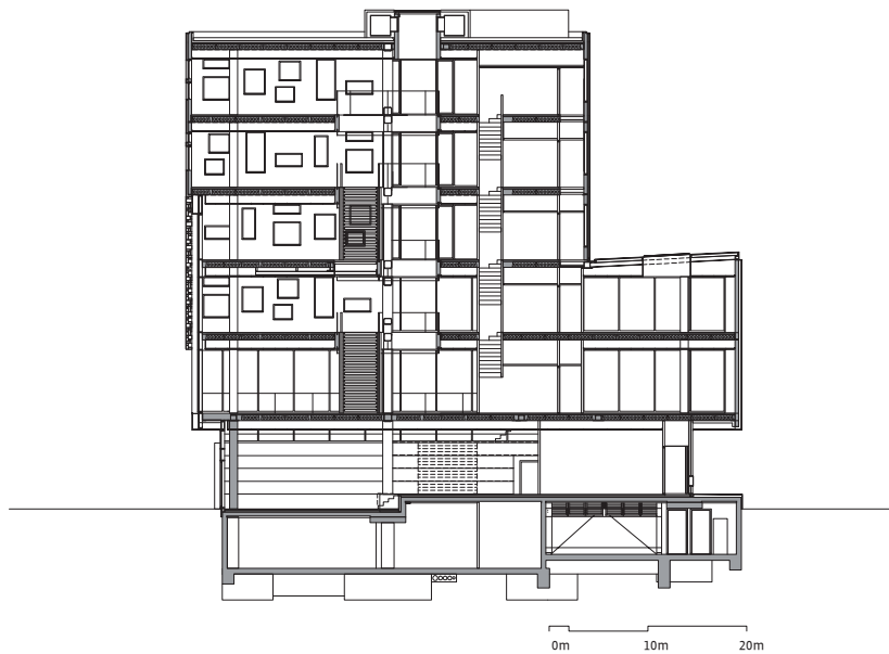
Doorsnede AA
