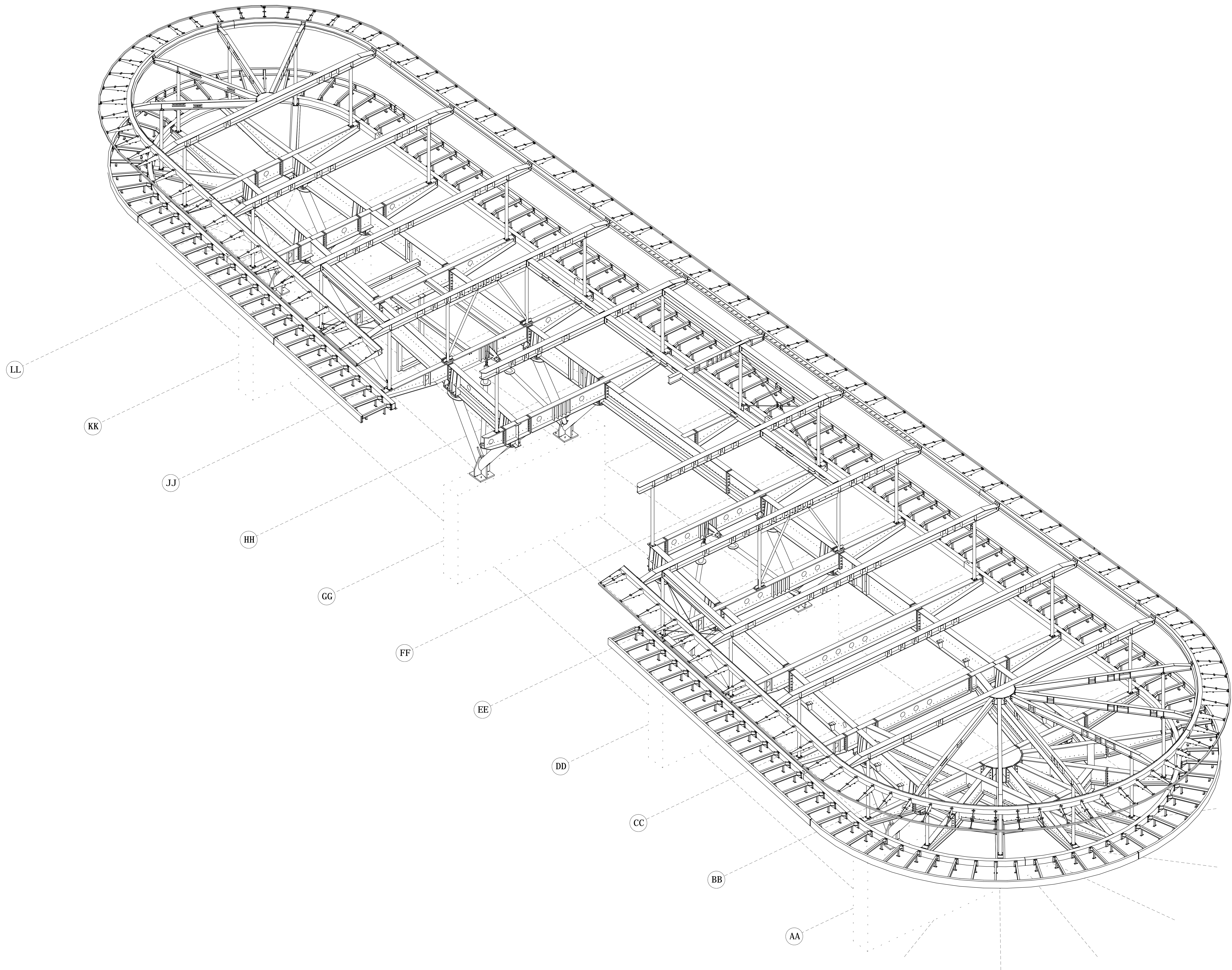
3-D Aanzicht gezien vanuit as 5-5 en AA
