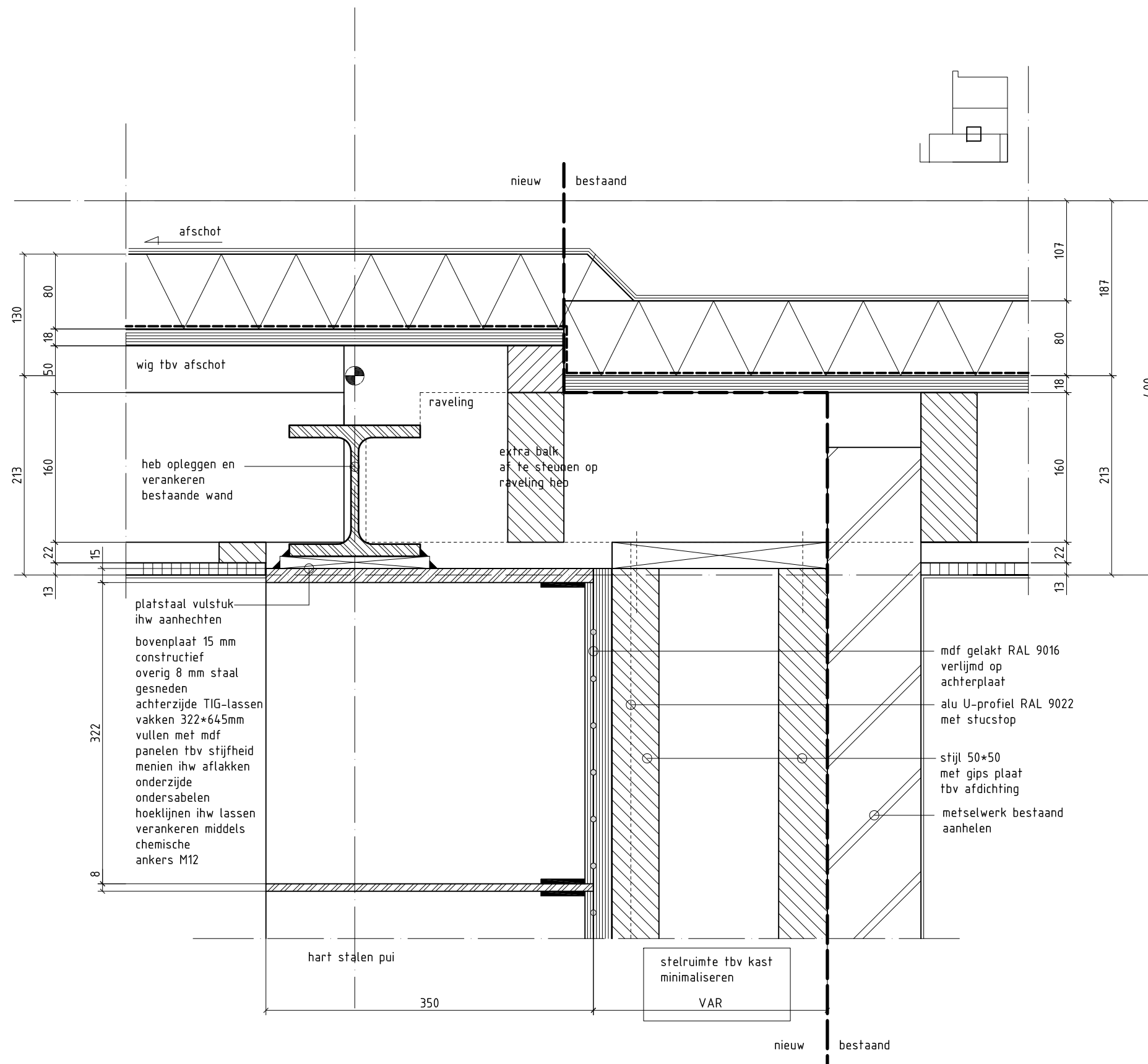
detail 1: principe aansluiting stalen kast
