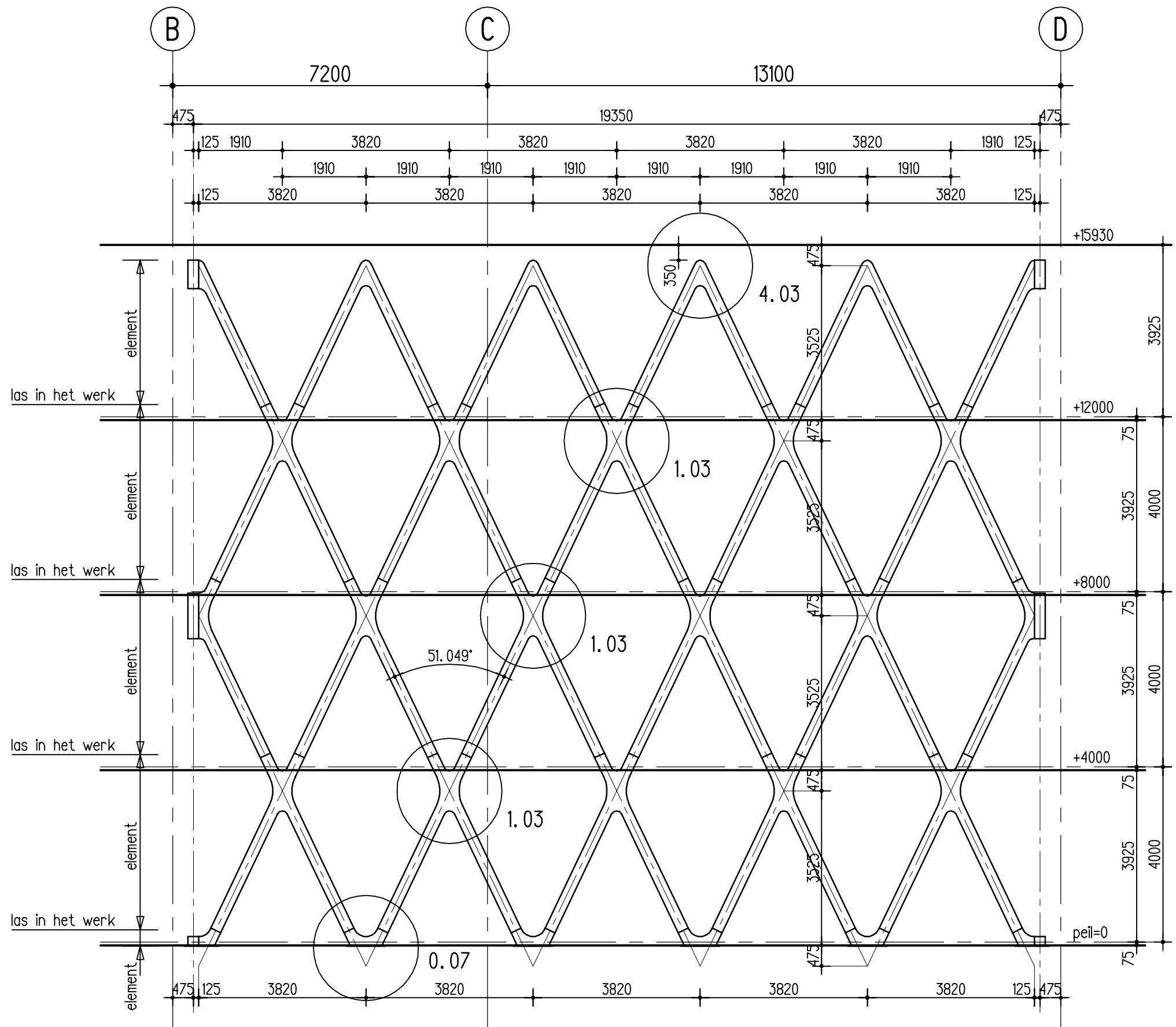
stalen vakwerk gevel evenwijdig aan as 02 en 04
