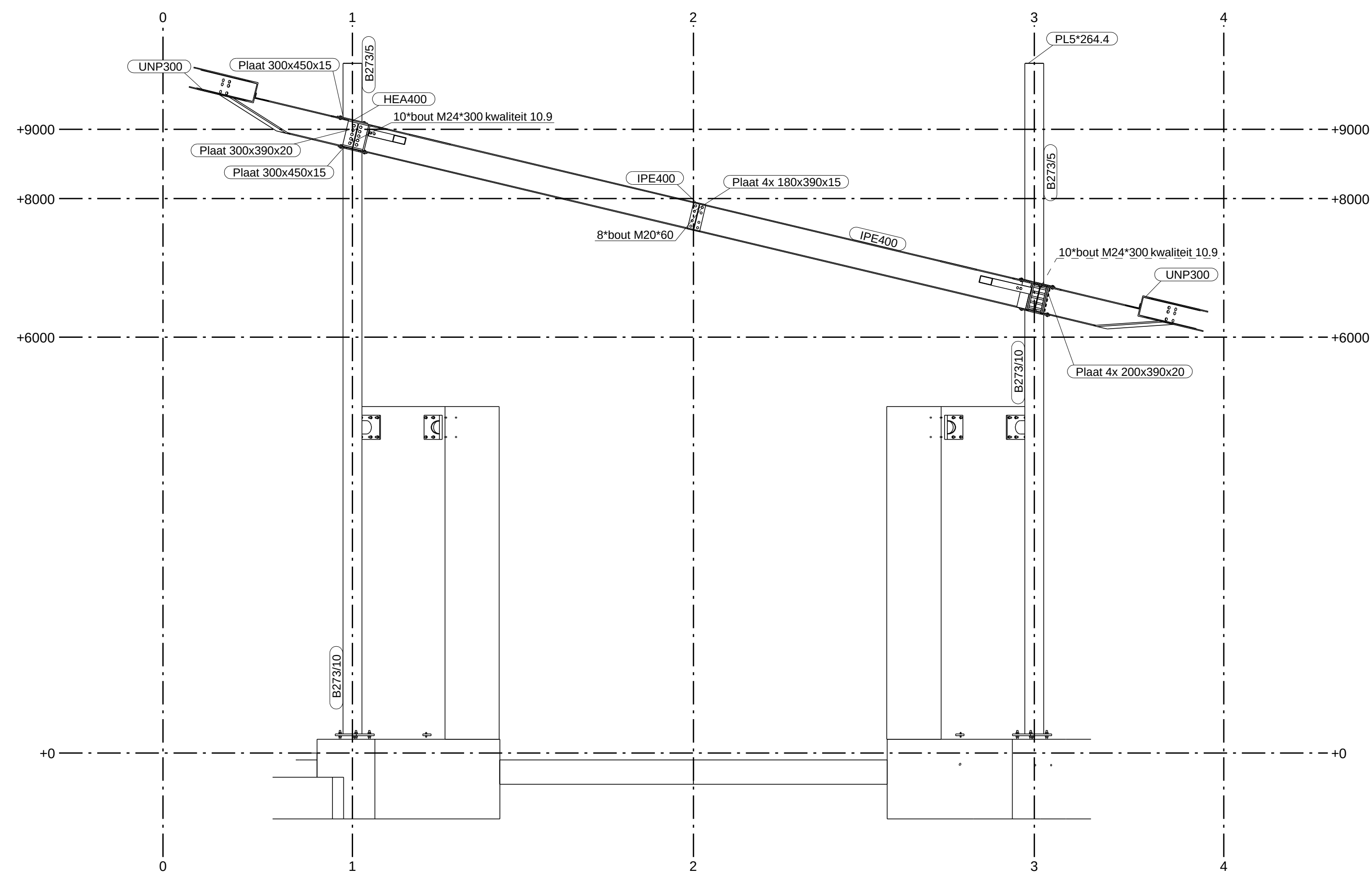
AANZICHT AS D 1:50
