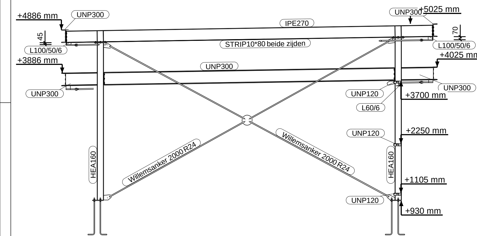
AANZICHT AS Fs 1:50
