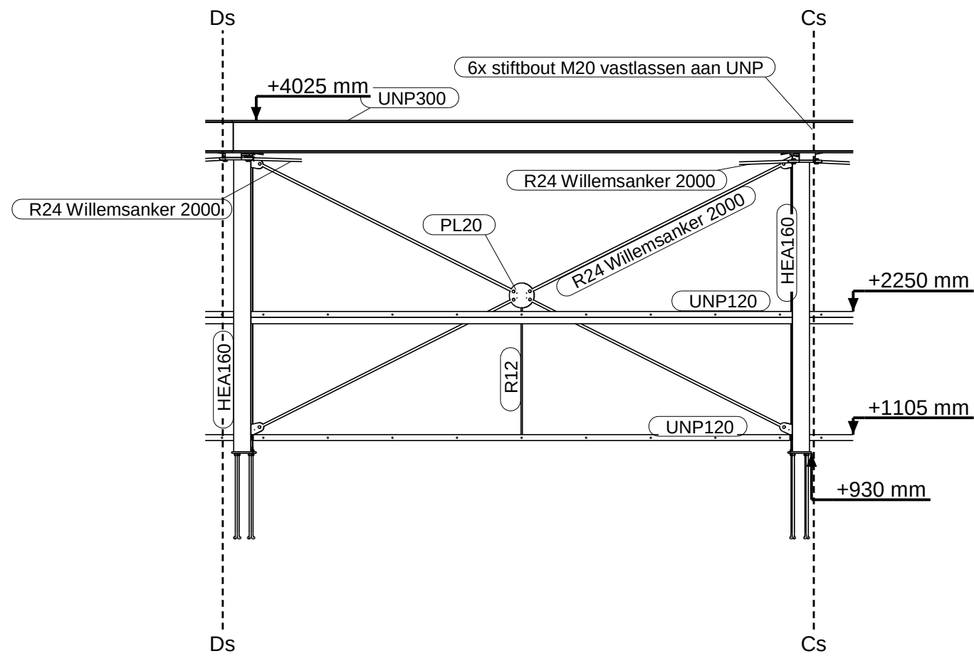
dsn C - C , 1:50 Zie tekening G [2], 4025+
