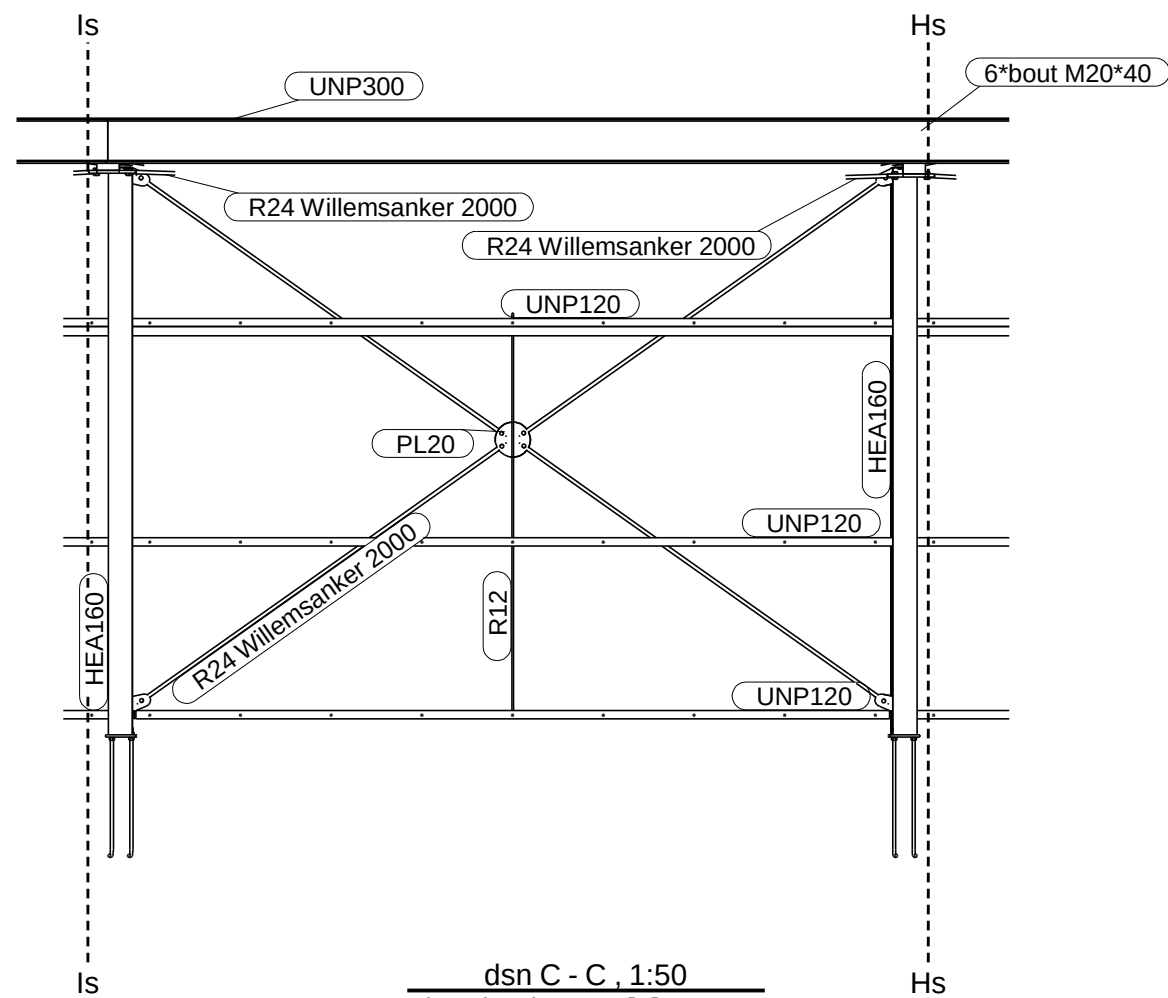
dsn C - C , 1:50 Zie tekening G [2], 4025+
