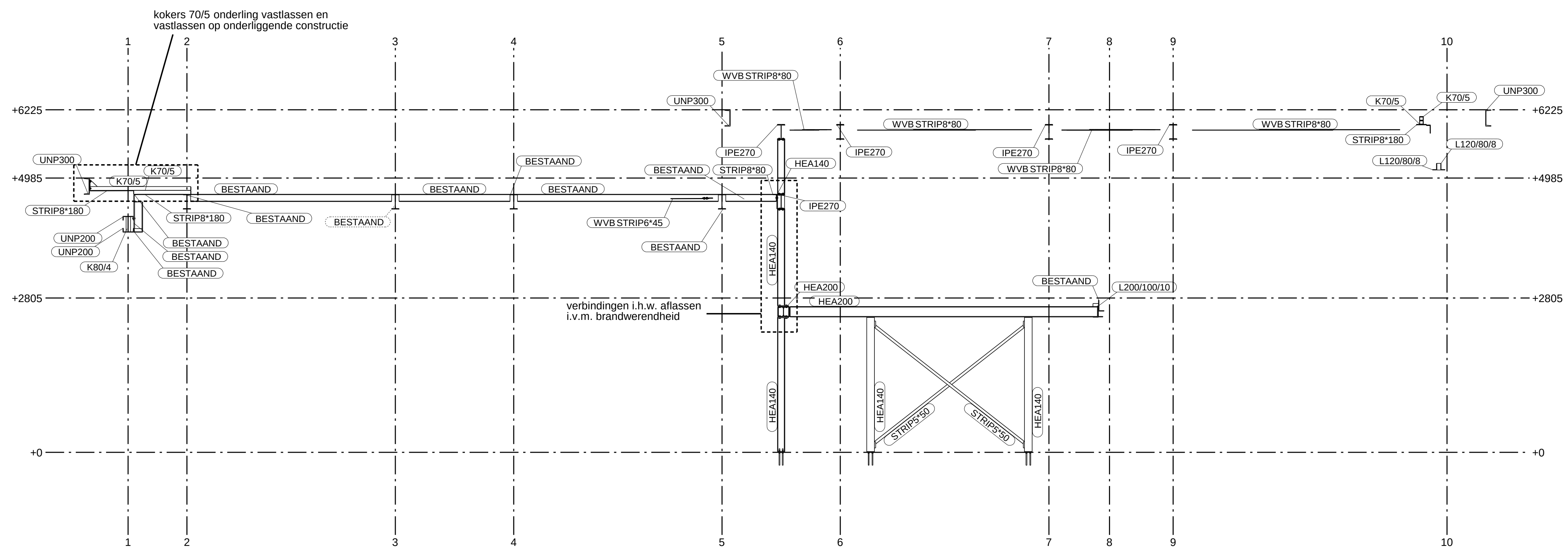
AANZICHT AS B 1:50
