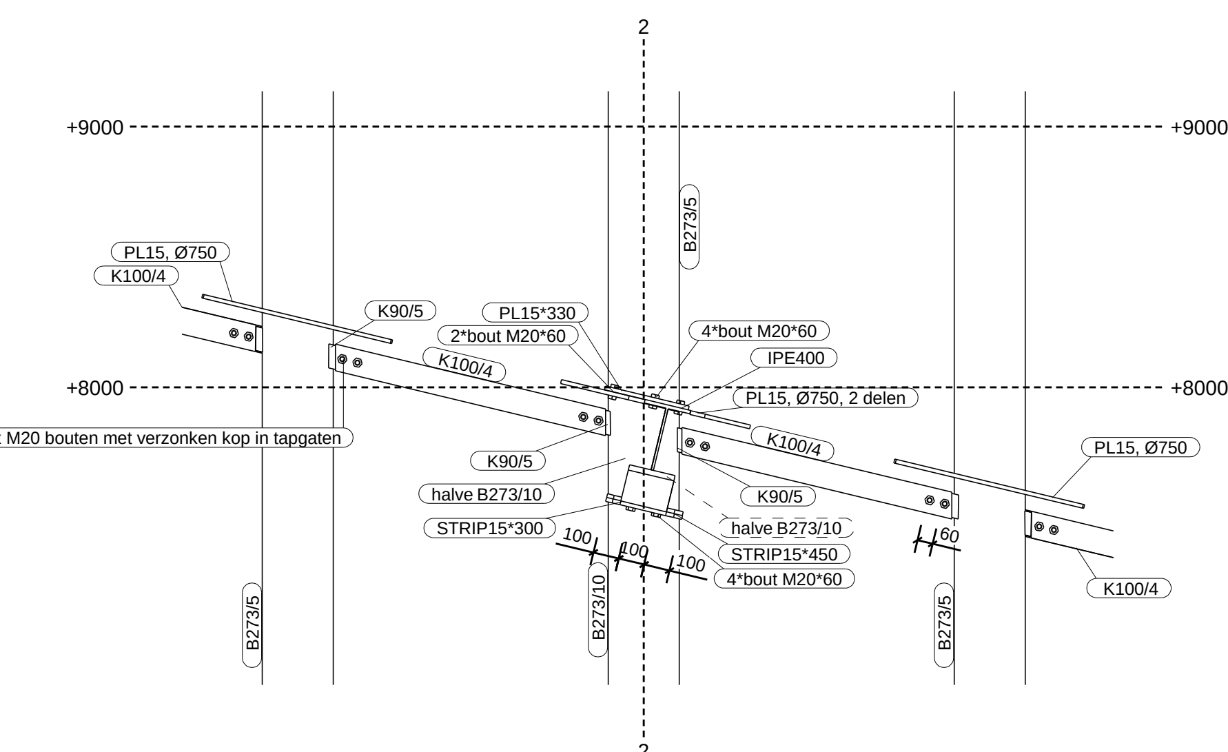
dsn C - C, 1:20 Zie tekening G [3], OVERZICHT
