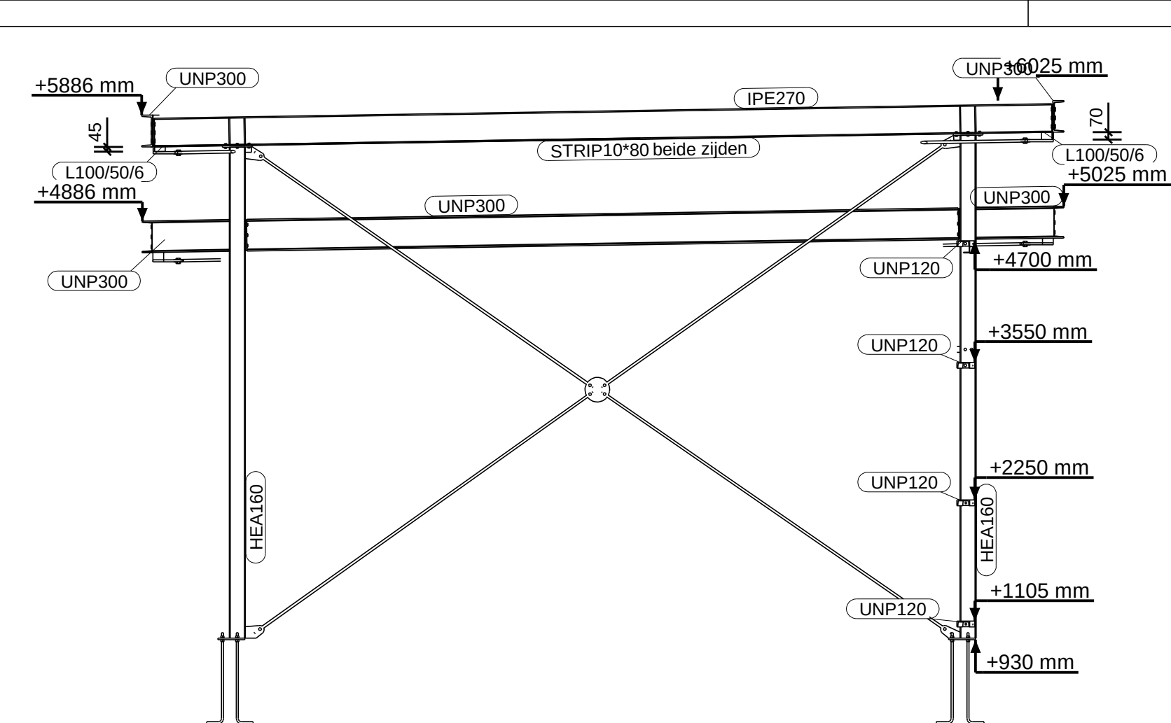
AANZICHT AS Ks 1:50
