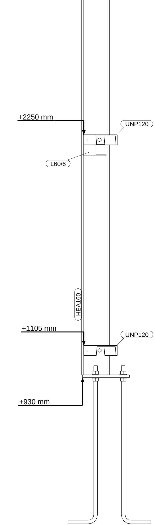
dsn A - A, 1:10
