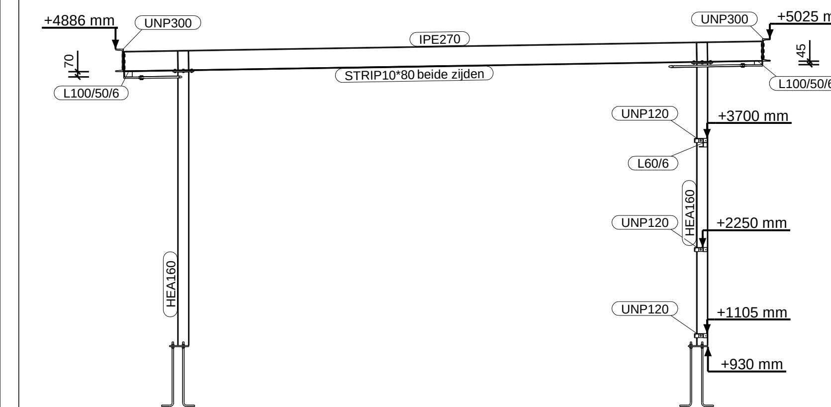
AANZICHT AS Gs t/m Js 1:50
