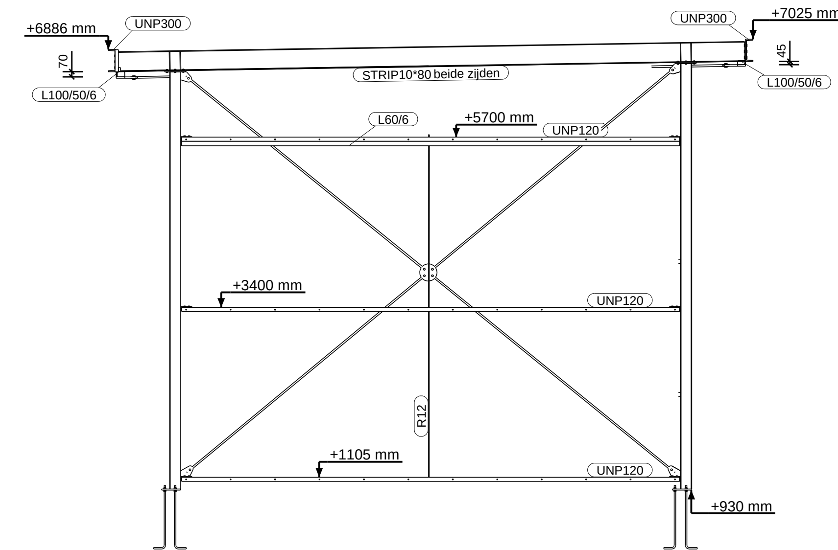
AANZICHT AS Us 1:50
