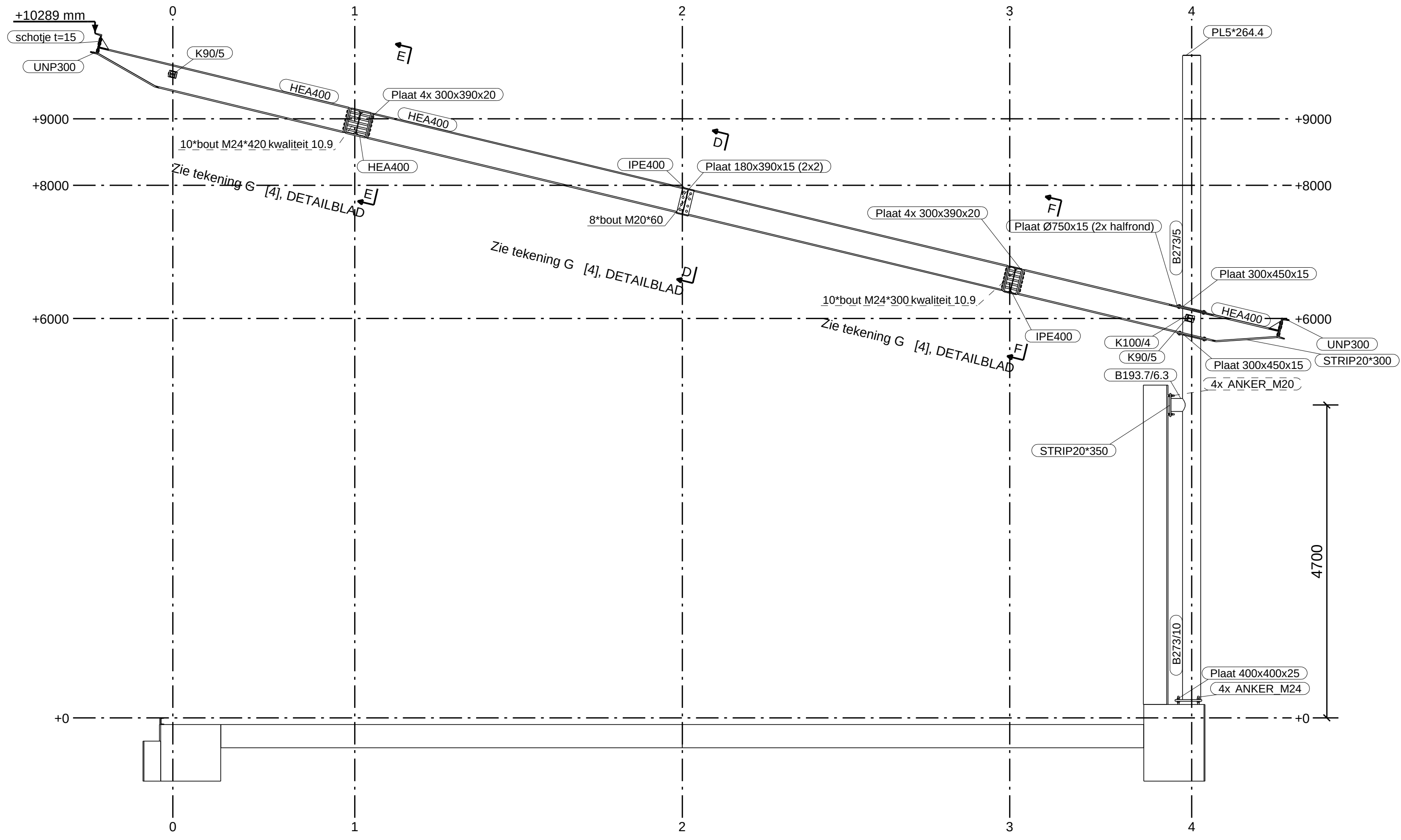
AANZICHT AS C 1:50
