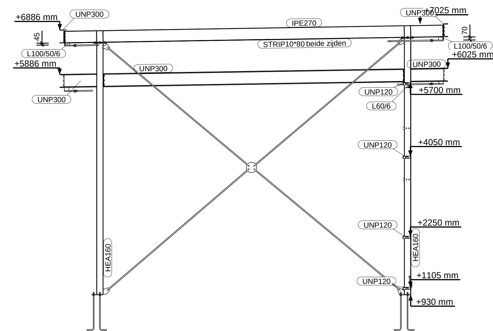
AANZICHT AS Ps 1:50
