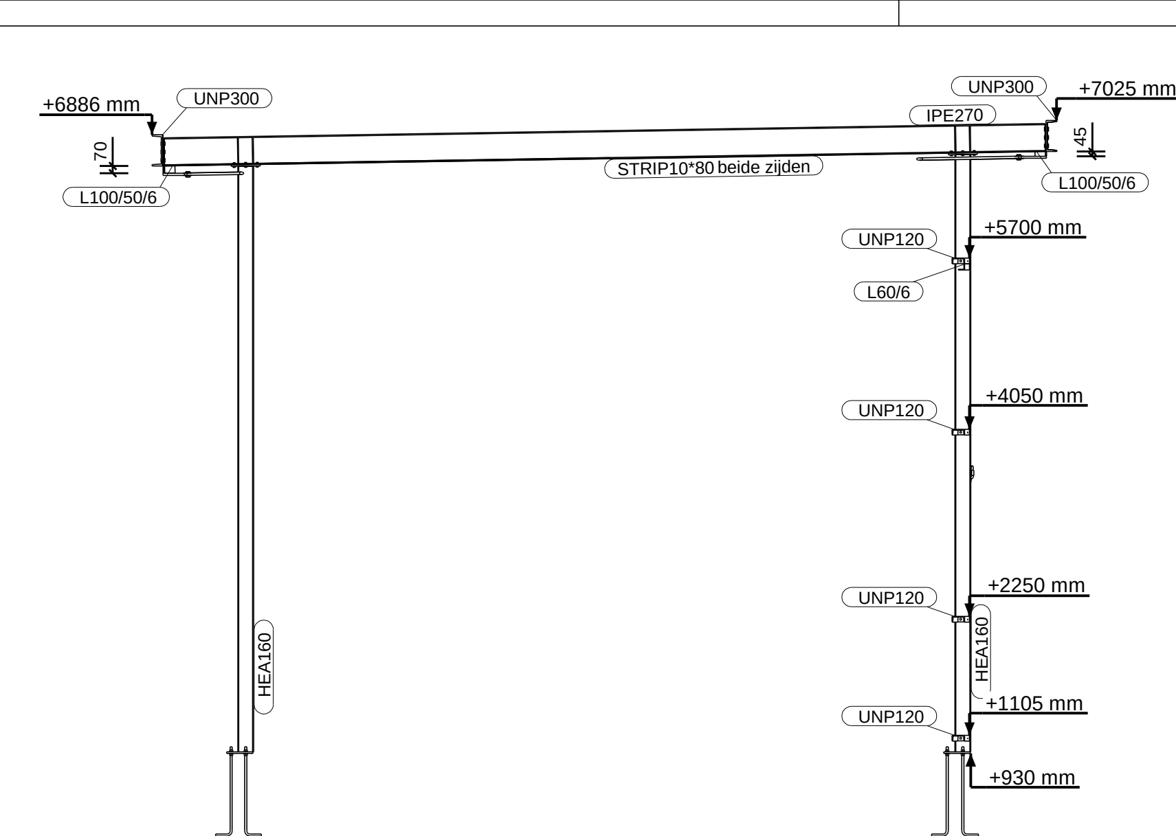
AANZICHT AS Os t/m Ts 1:50
