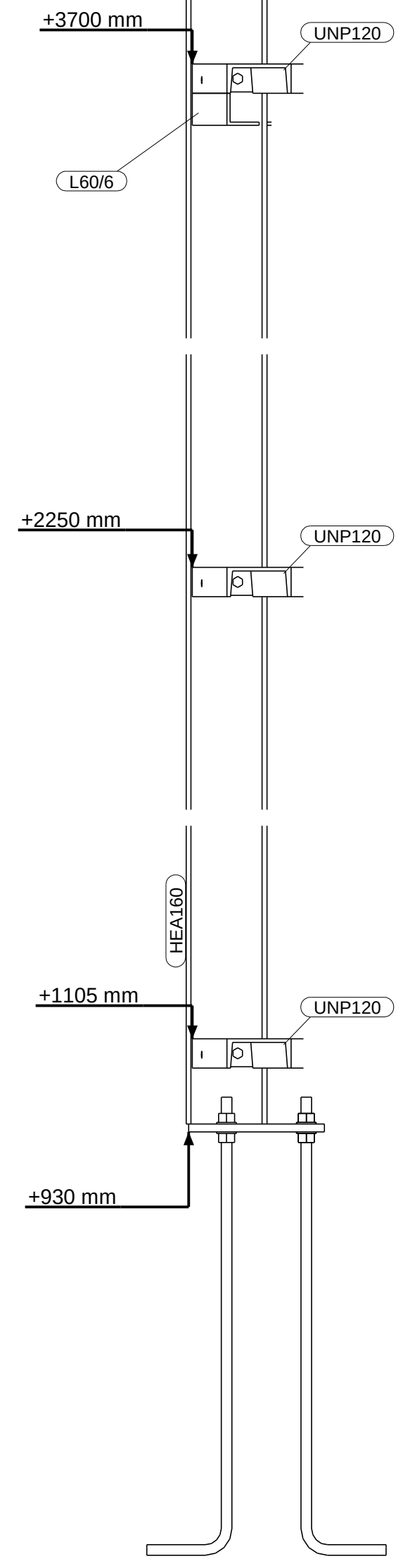
dsn A - A, 1:10
