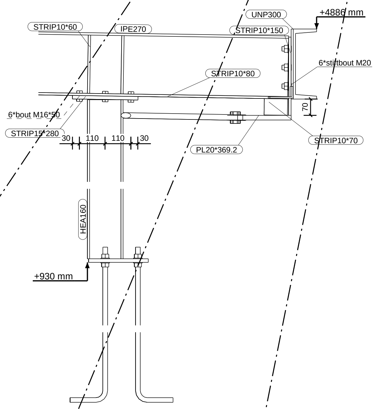
dsn B - B, 1:10
