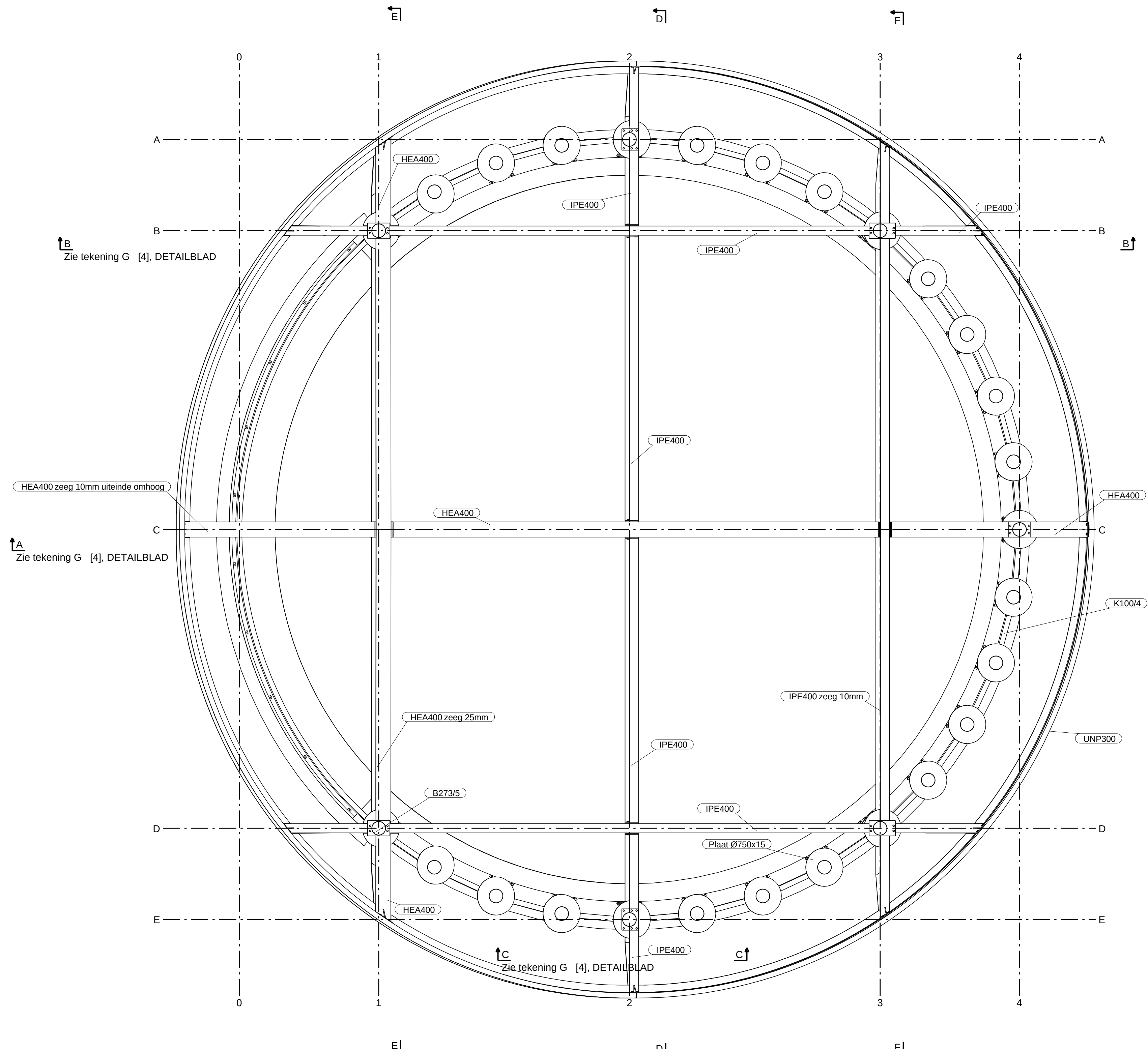
Boven aanzicht 1:50
