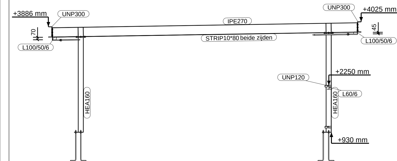
AANZICHT AS Bs t/m Es 1:50
