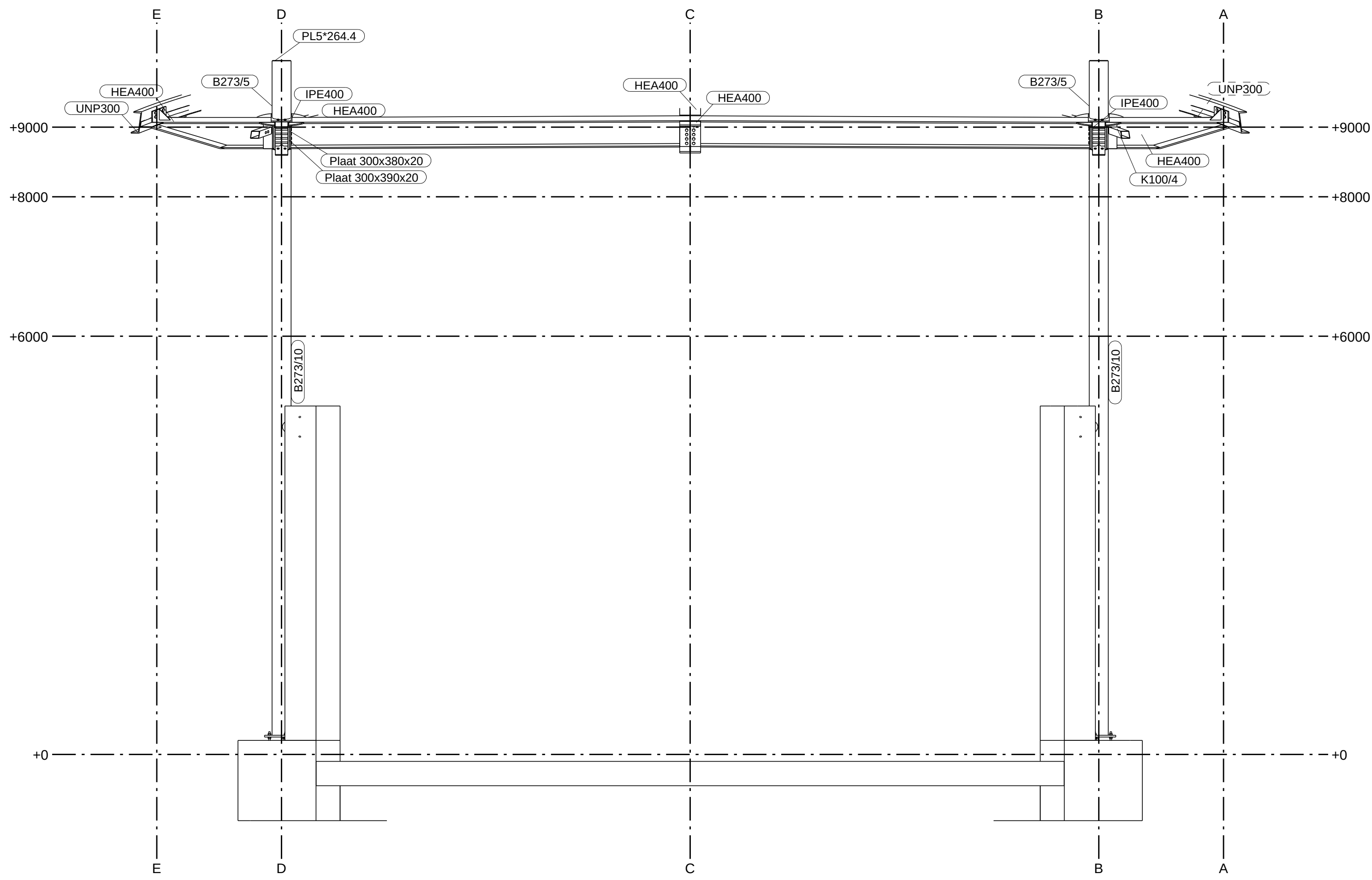
AANZICHT AS 1 1:50
