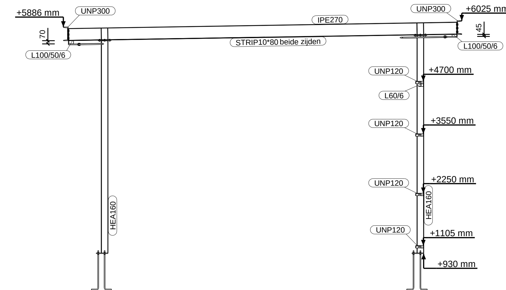
AANZICHT AS Ls t/m Os 1:50
