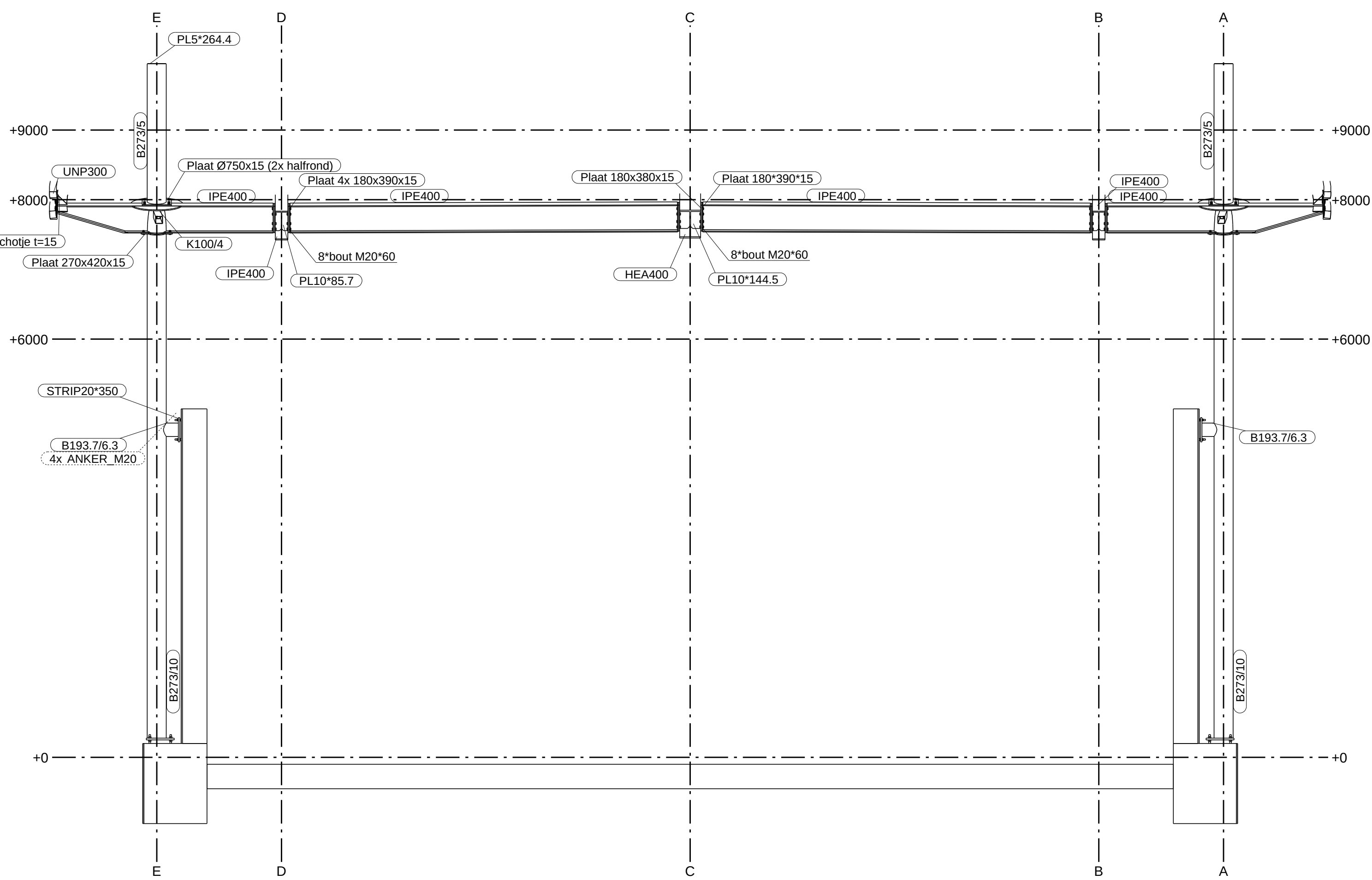
AANZICHT AS 2 1:50
