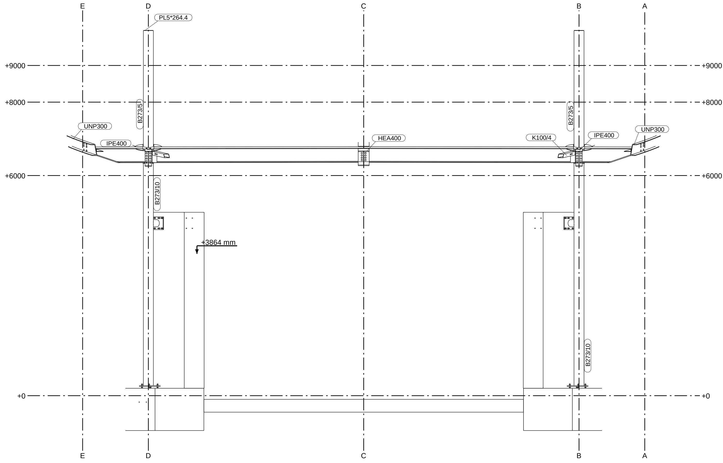
AANZICHT AS 3 1:50
