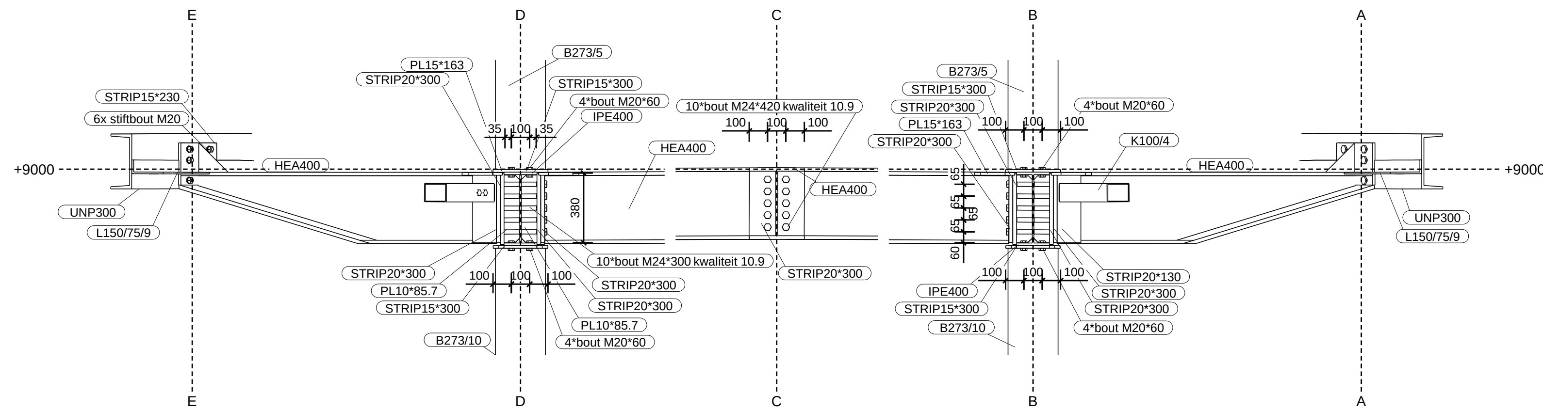
dsn E - E, 1:20 Zie tekening G [3], OVERZICHT
