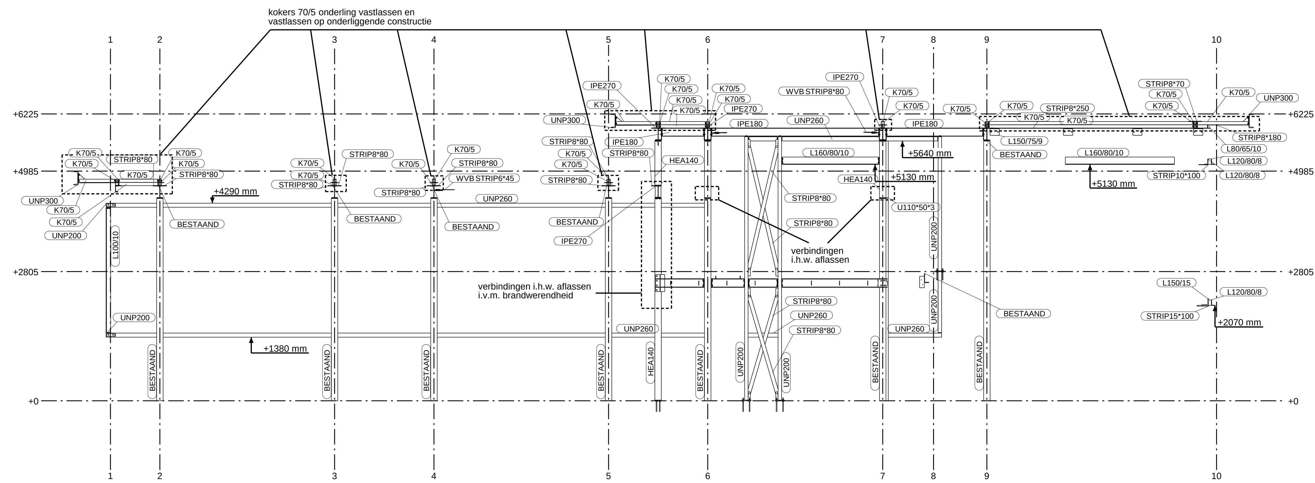
AANZICHT AS A 1:50
