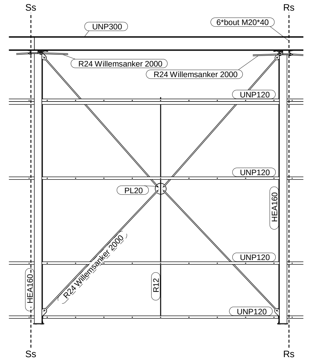
dsn C - C , 1:50 Zie tekening G [5], 7025+
