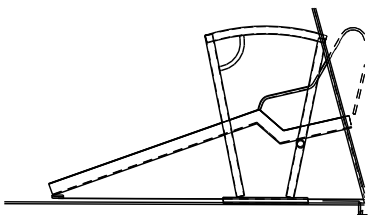
Doorsnede B - B ENKEL REK - HOOG
