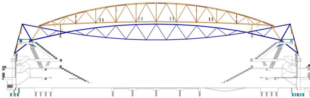
Dwarsdoorsnede bestaand + nieuw
