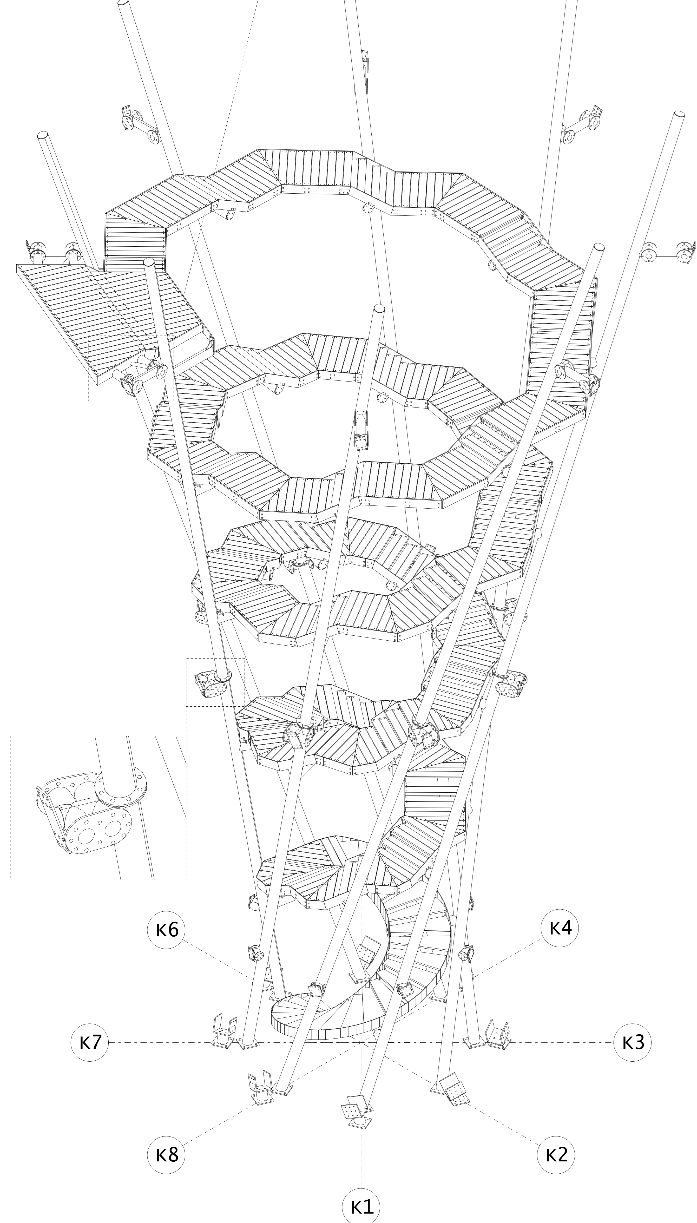
AANZICHT KOLOMMEN+BORDESSEN
