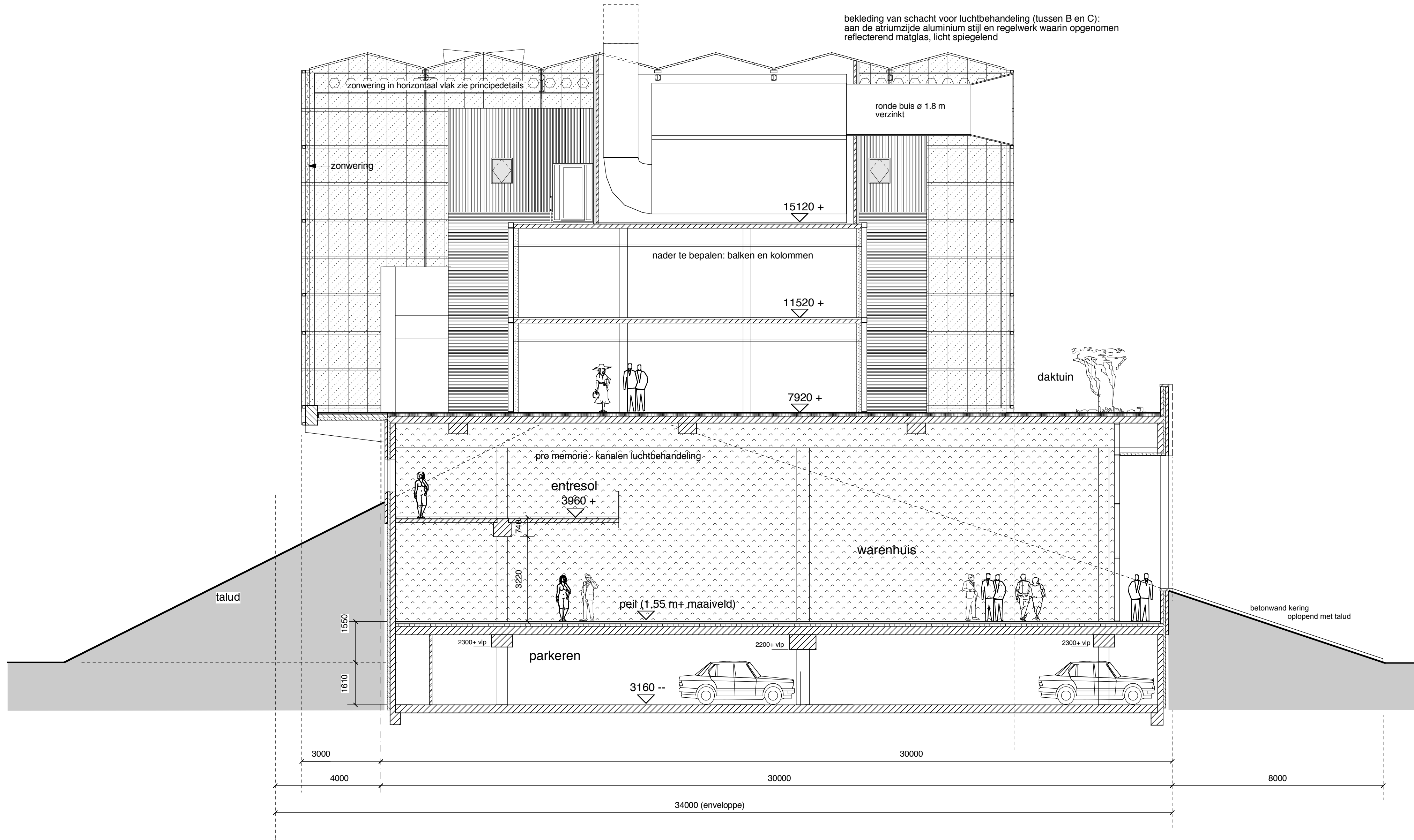
DOORSNEDE II-II
