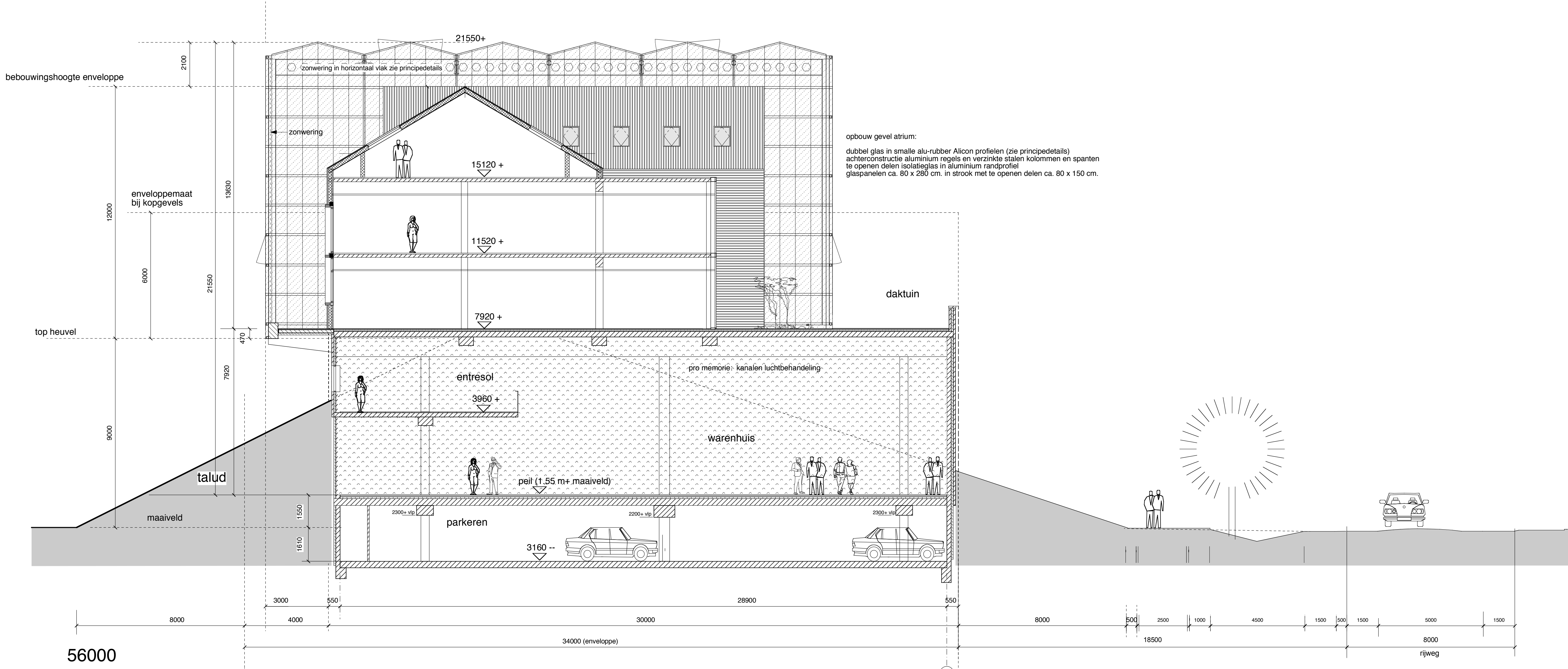
DOORSNEDE I-I
