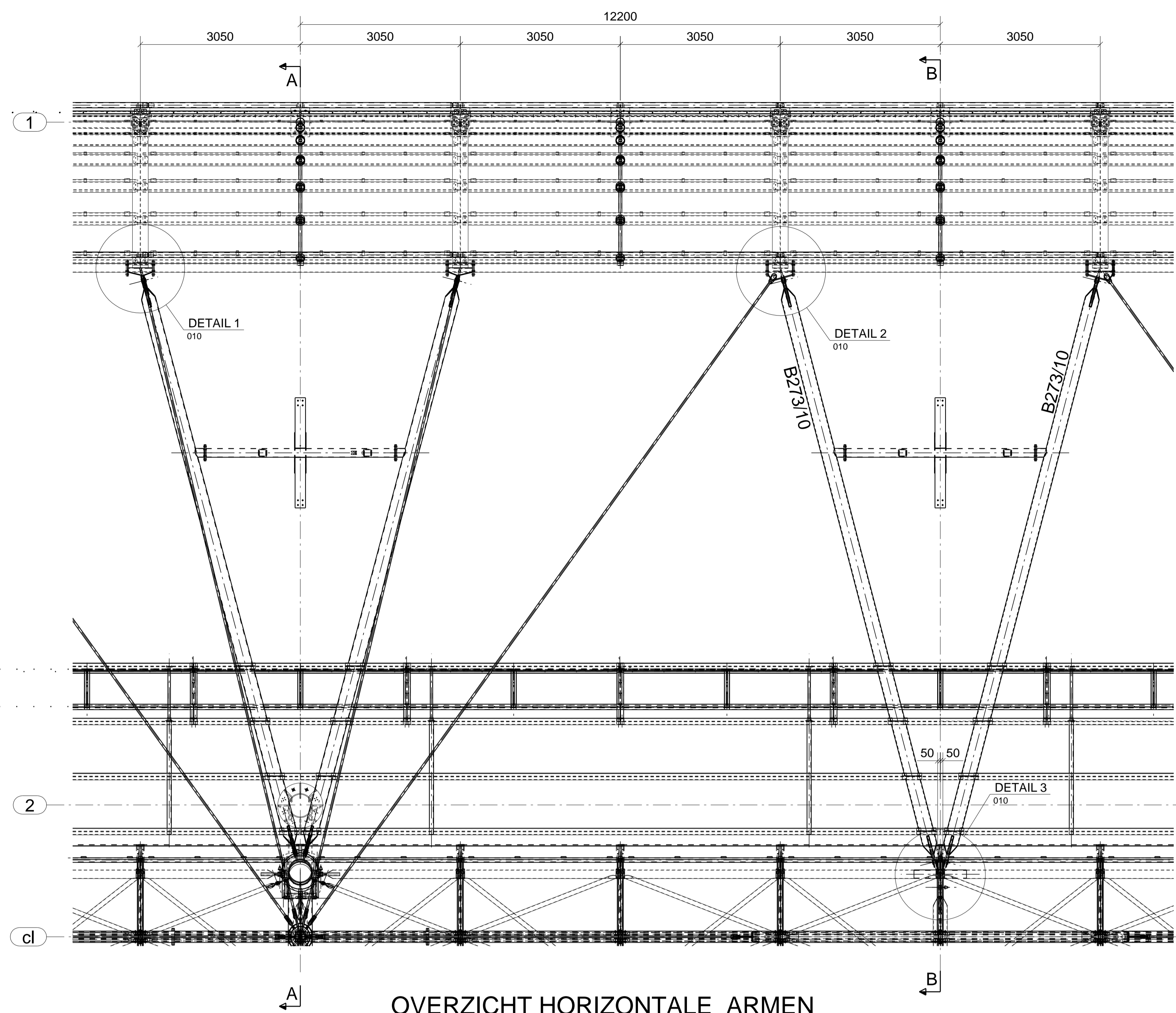
OVERZICHT HORIZONTALE ARMEN Schaal 1:50
