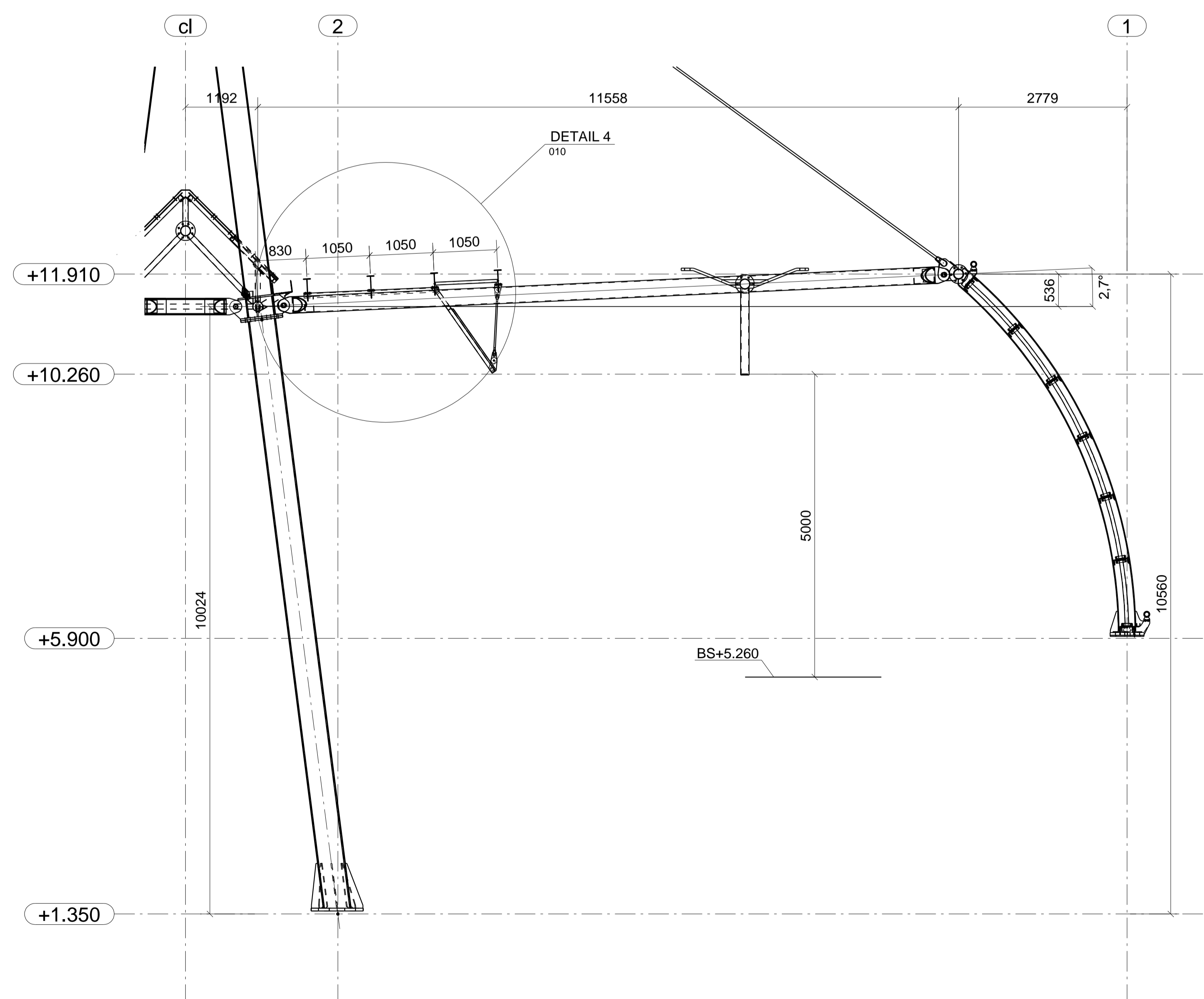
DOORSNEDEN A - A Schaal 1:50
