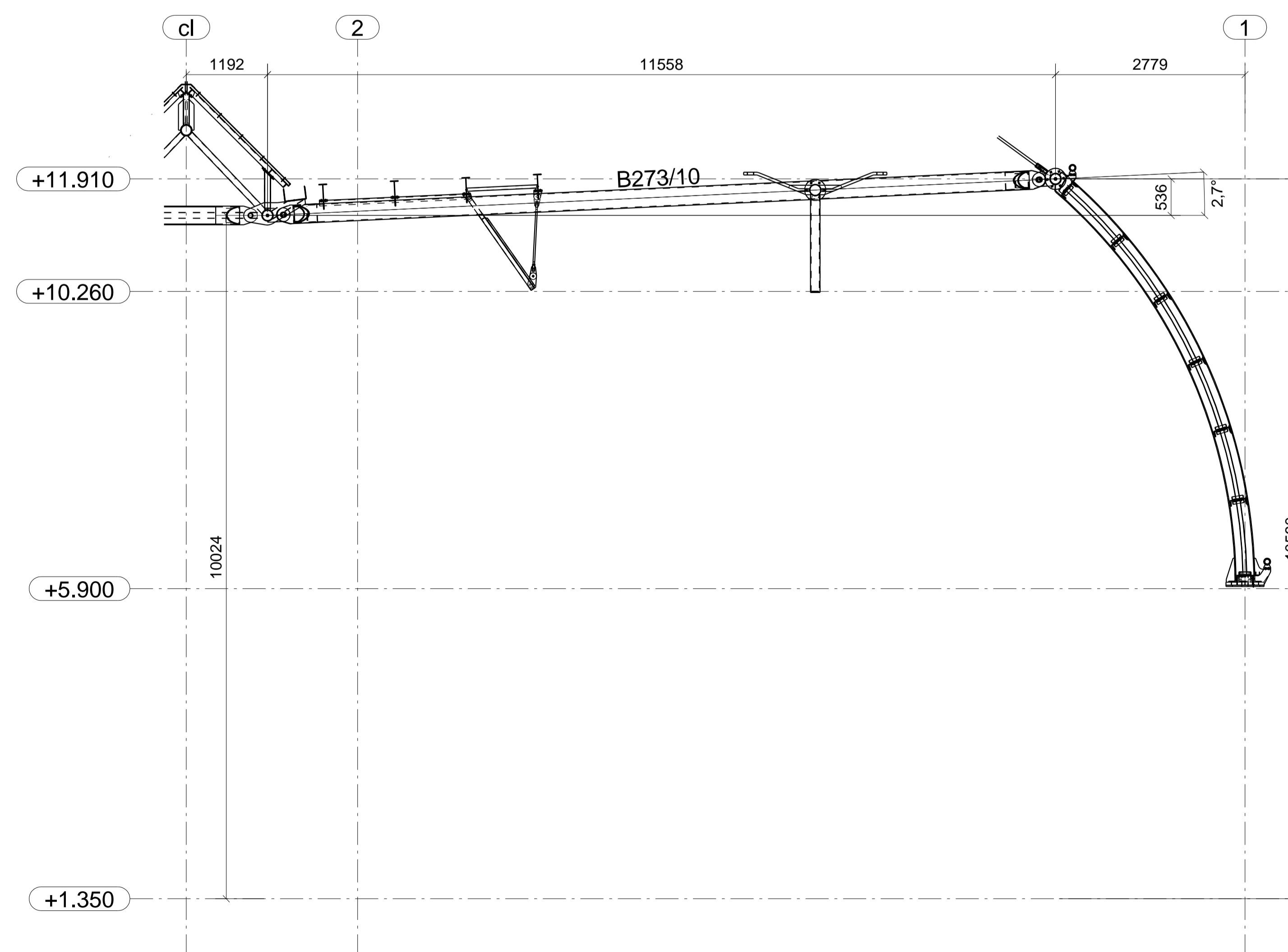
DOORSNEDEN B - B Schaal 1:50
