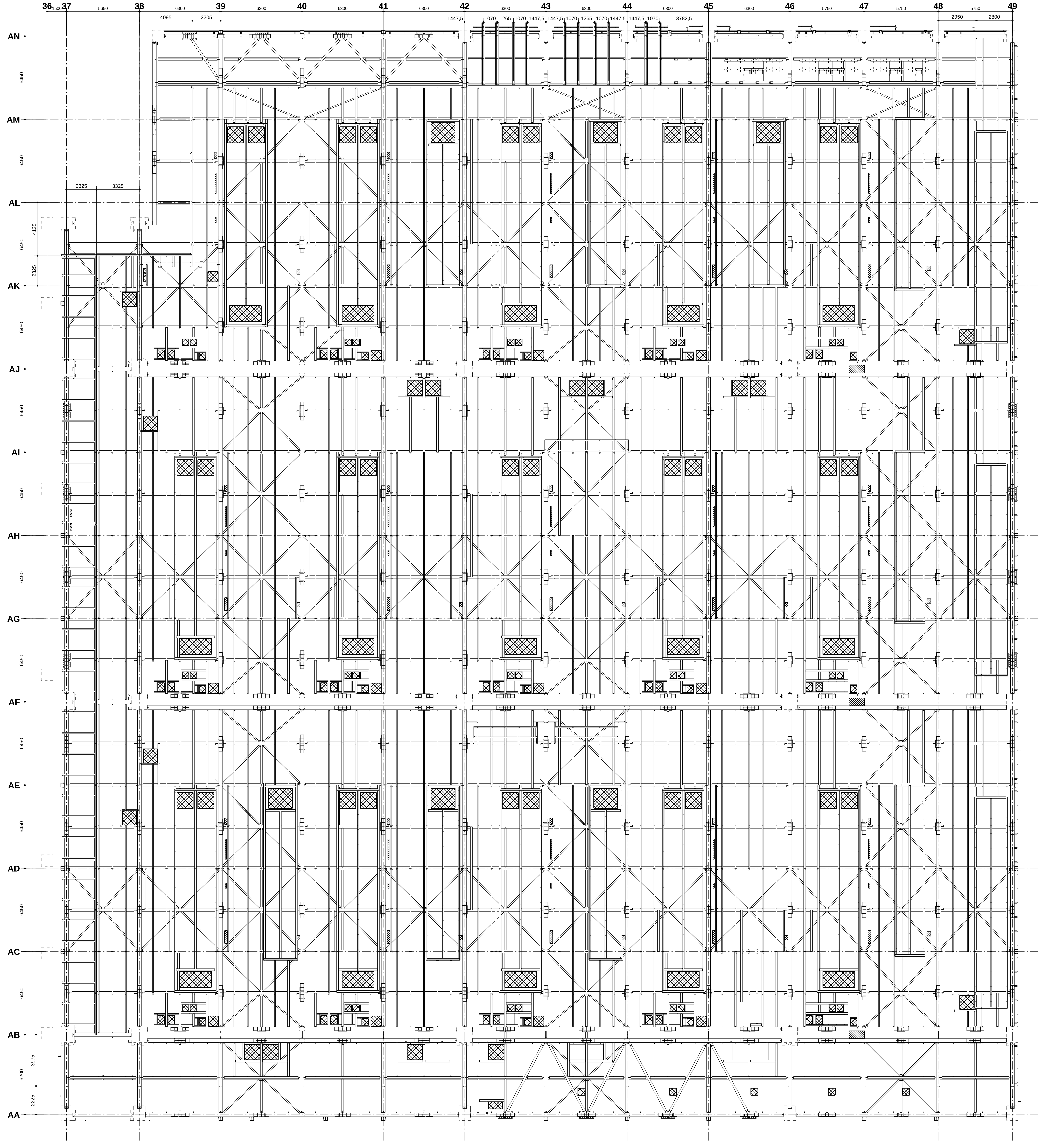
Bovenaanzicht 7800+
