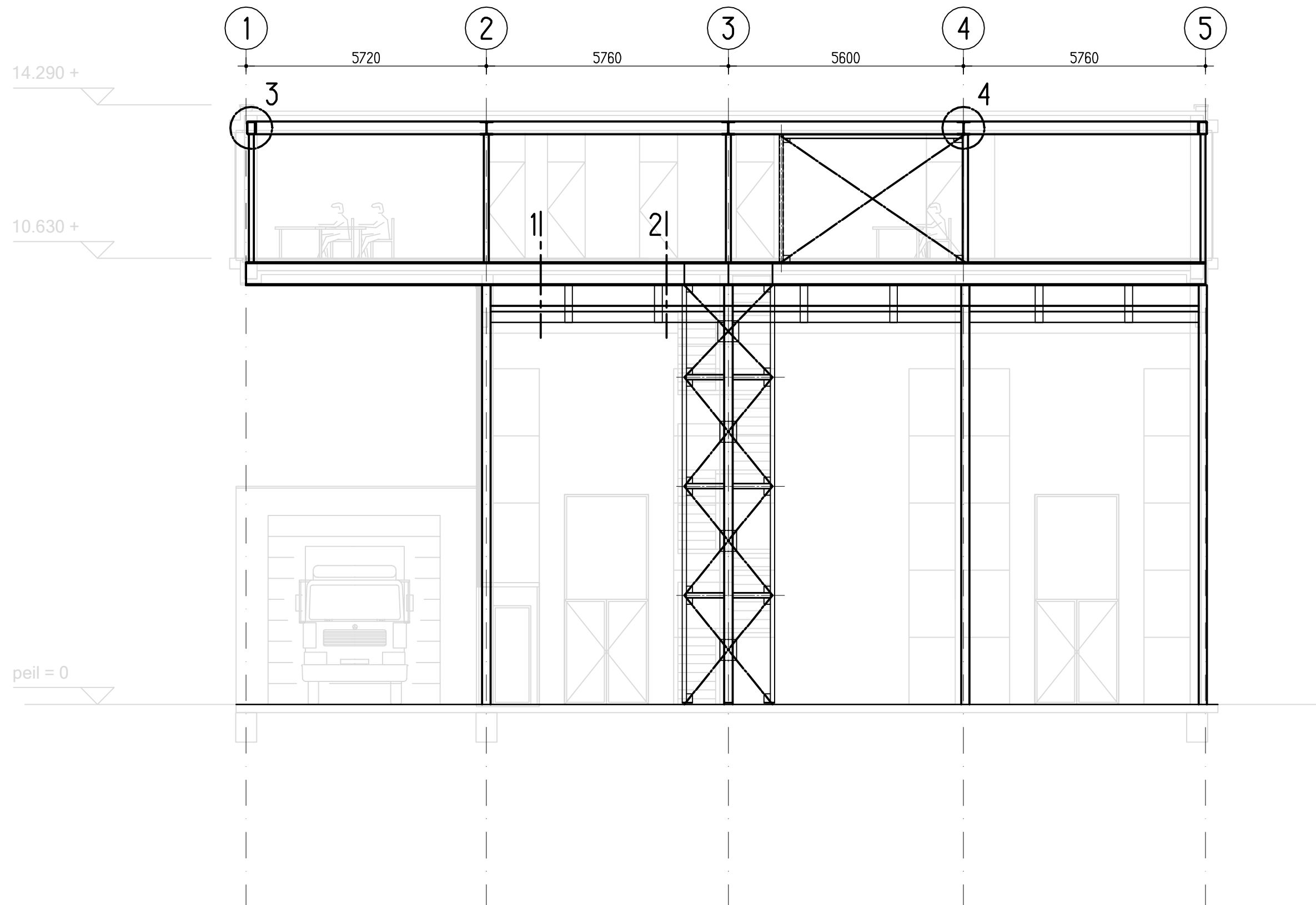
doorsnede bedrijfshal en kantoor
