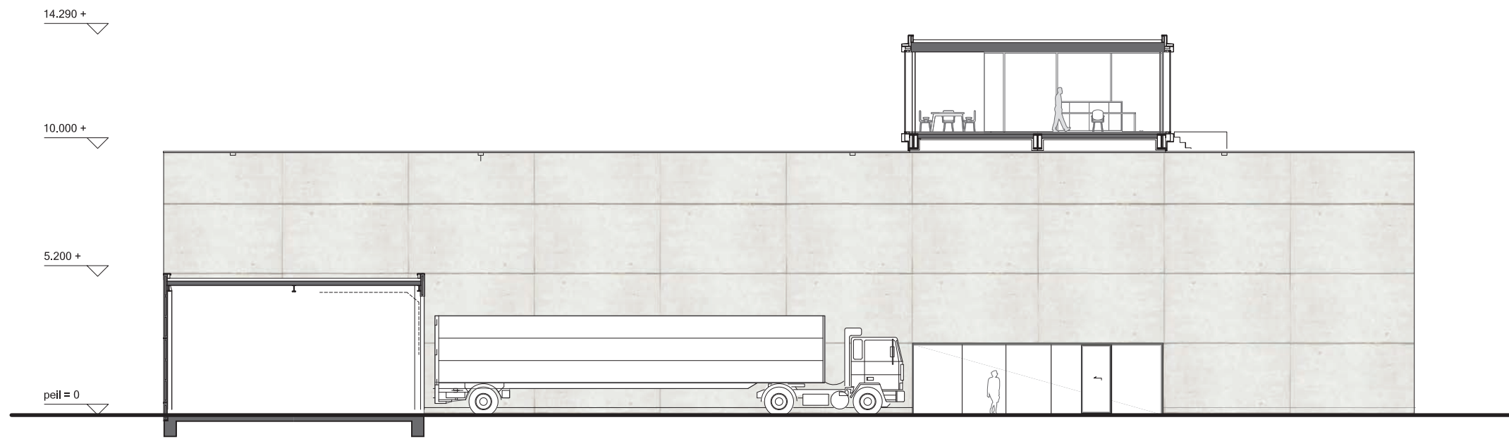
Langsdoorsnede CC
