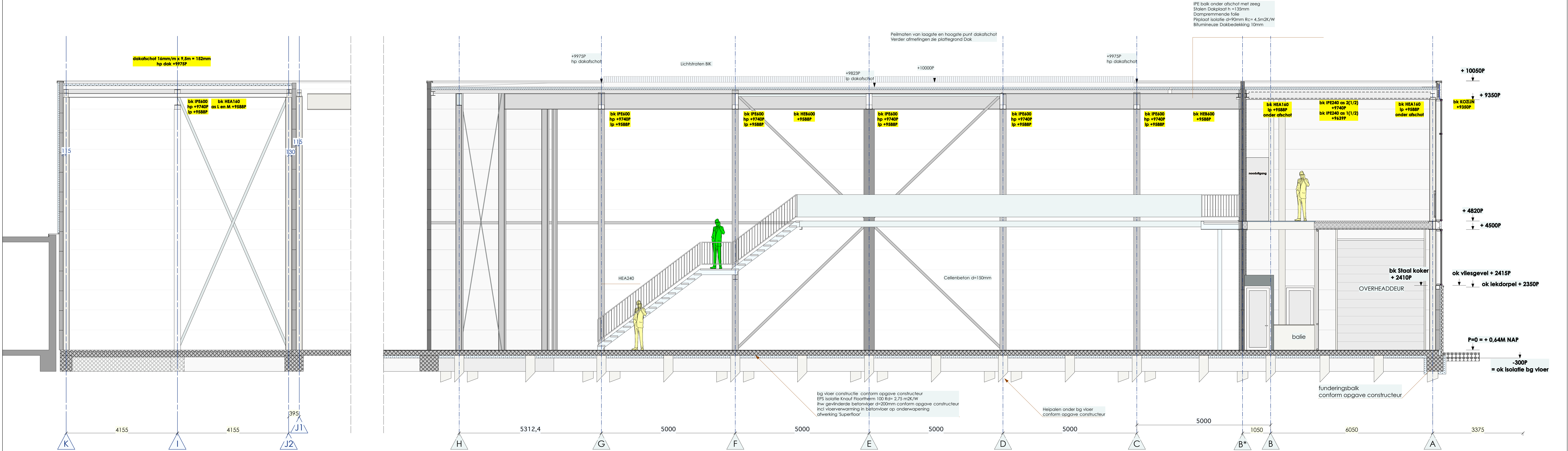
DOORSNEDE c - c
