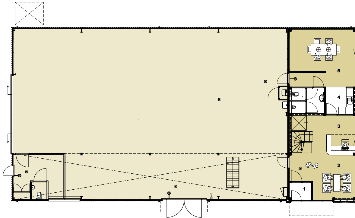
Begane grond
