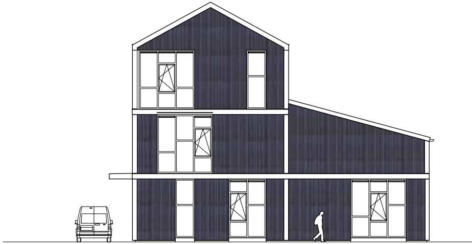
Oostgevel
