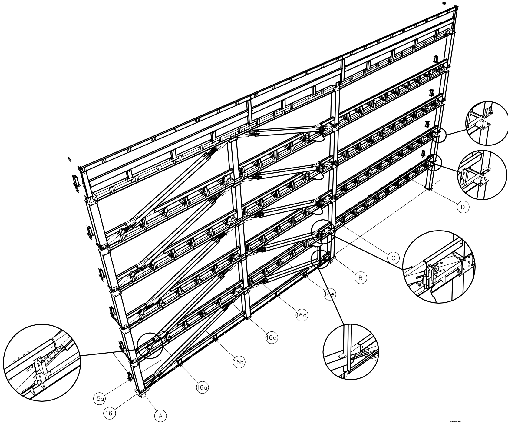
3-D Aanzicht
