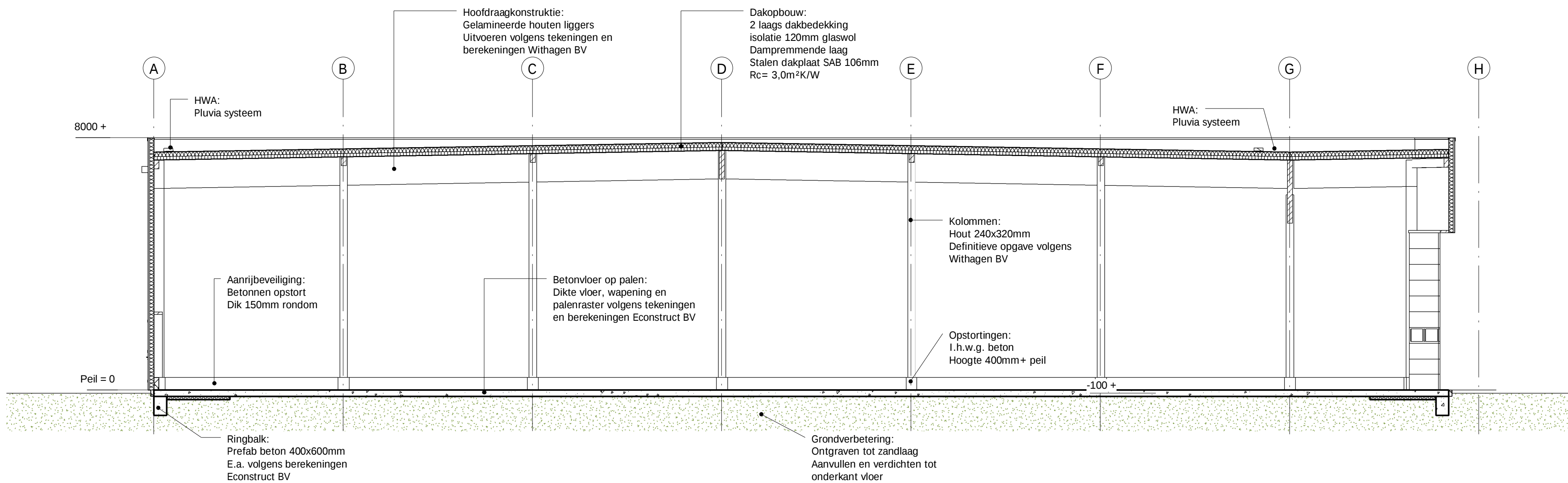
- Doorsnede B - B -
