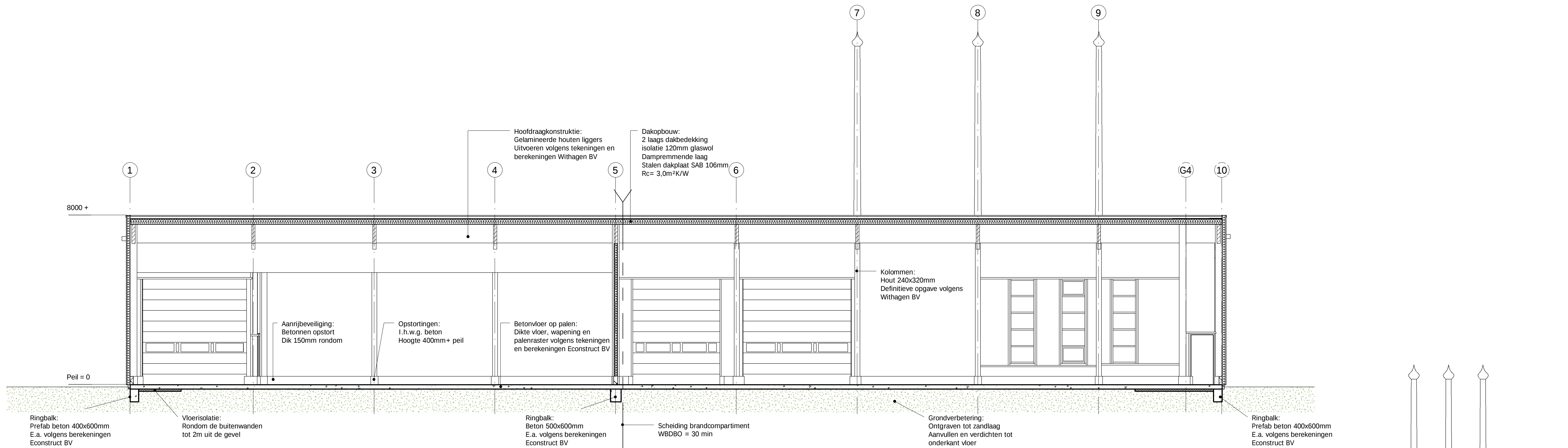
- Doorsnede C - C -
