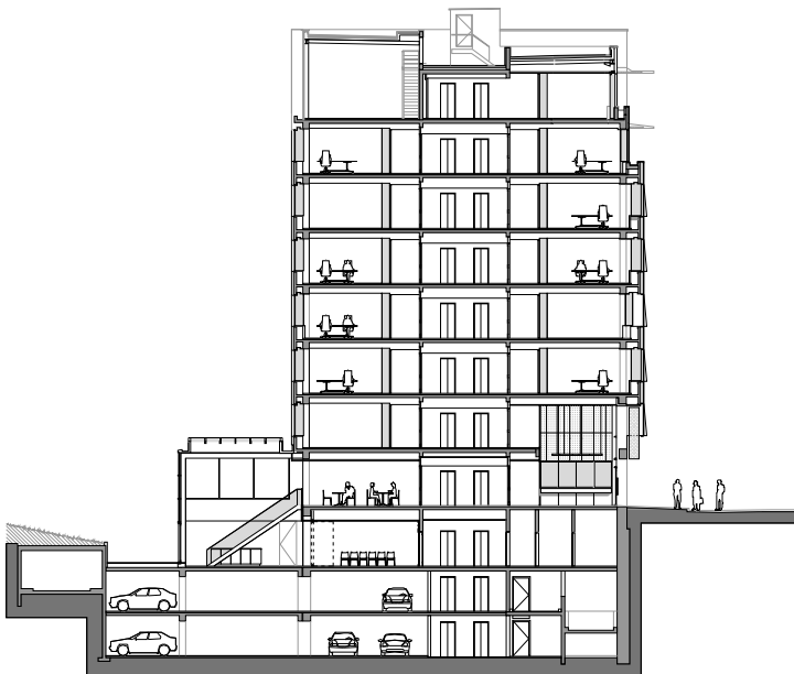
dwarsdoorsnede (nieuw)
