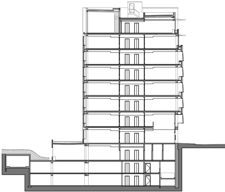
dwarsdoorsnede (bestaand)
