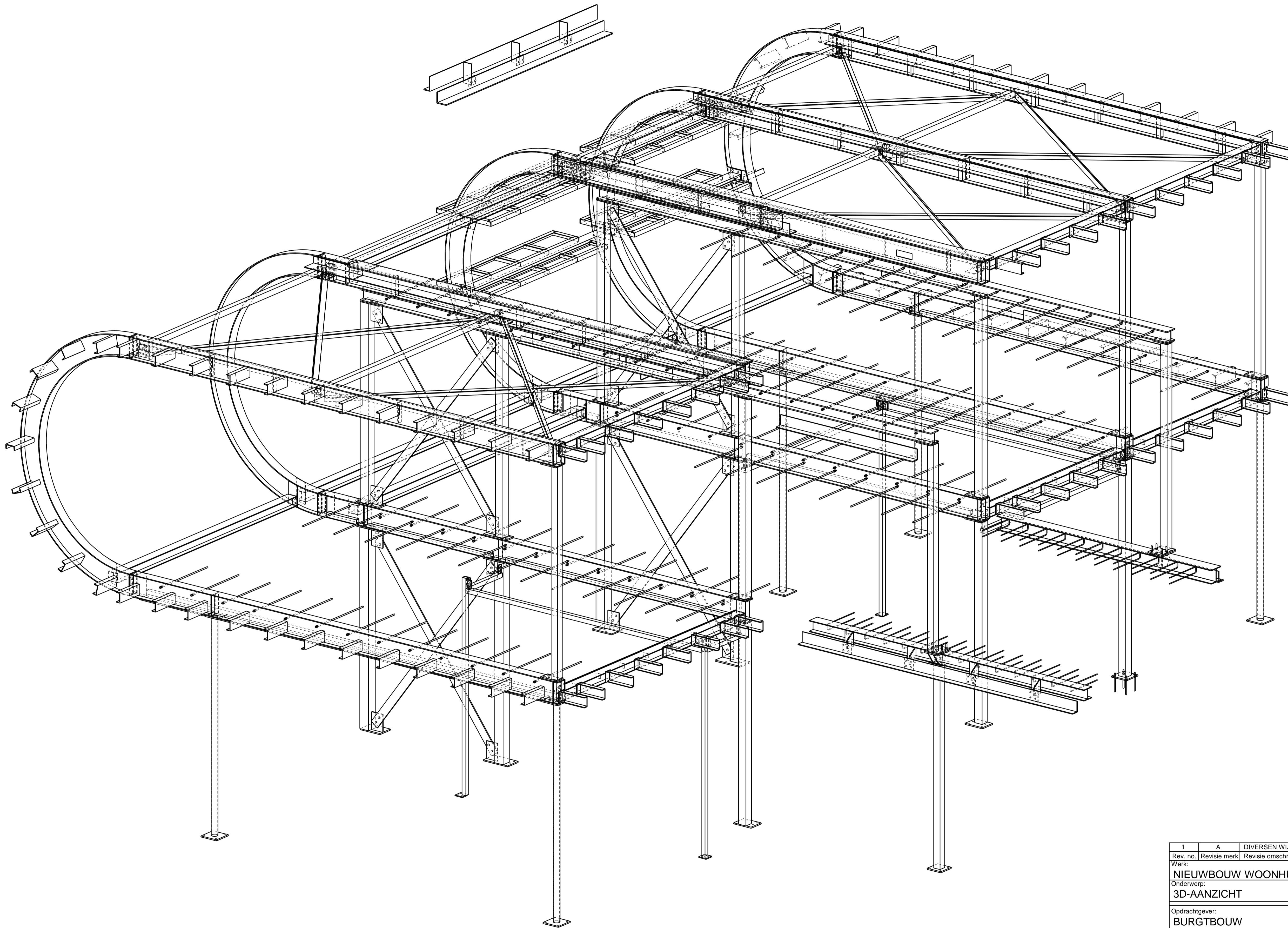
3D-AANZICHT
