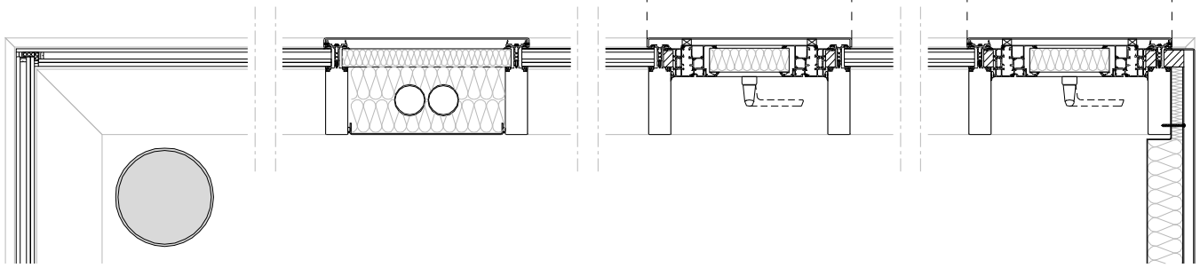
hoek noord-west gevel glas - glas aansluiting
