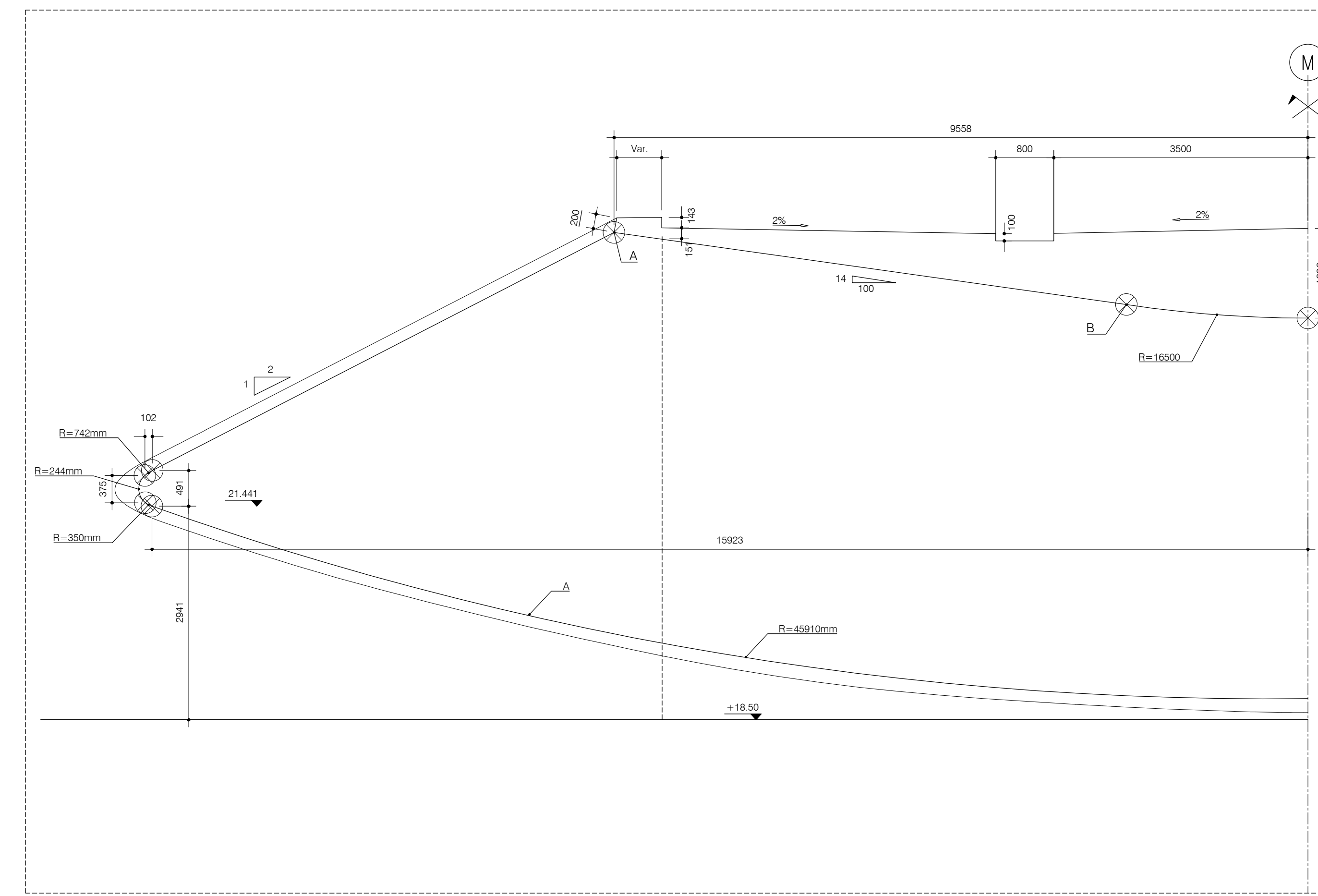
Aanzicht landhoofd Schaal 1:50
