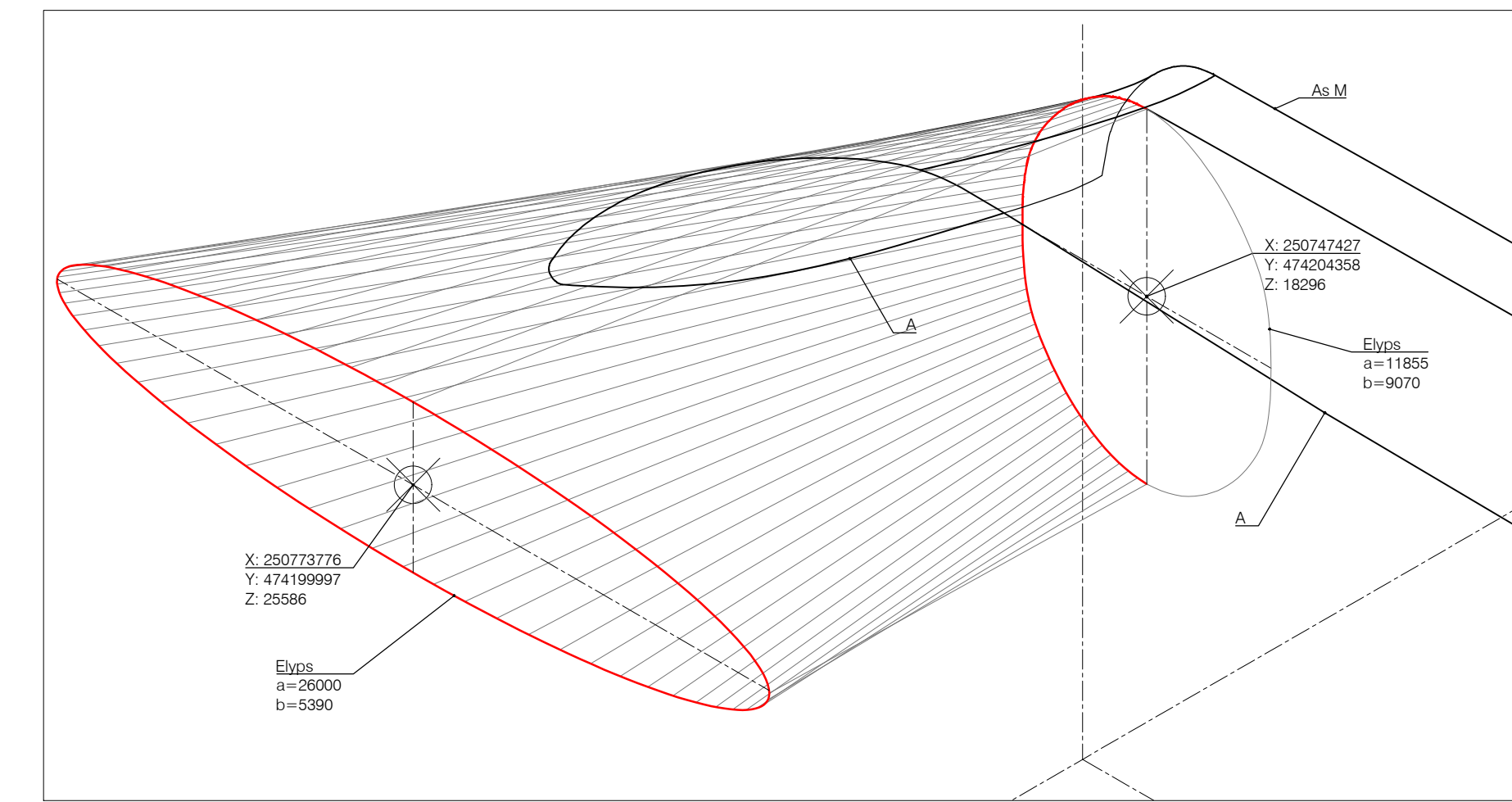
Principe opbouw geometrie landhoofd (LH0)
