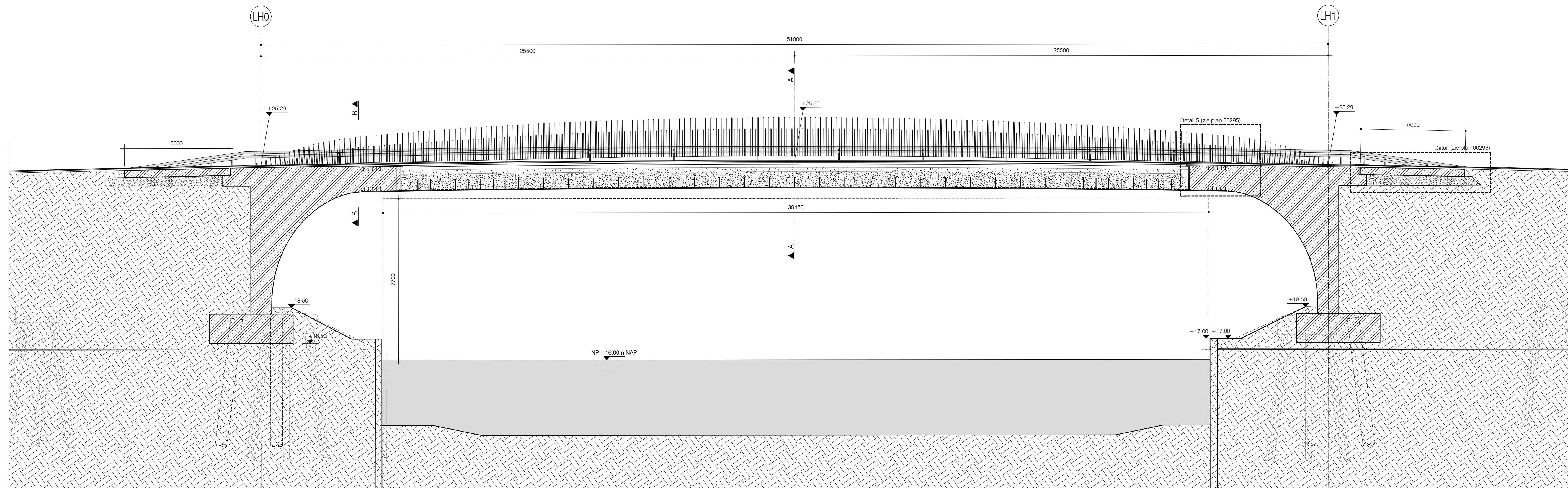
Lengtedoorsnede Schaal 1:100
