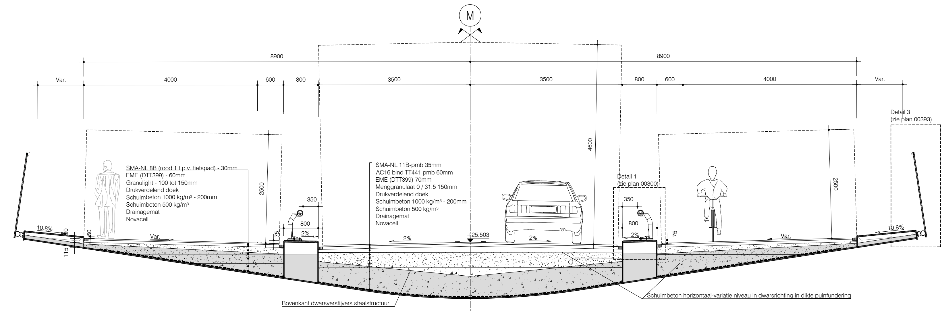
Snedes A-A Schaal 1:20
