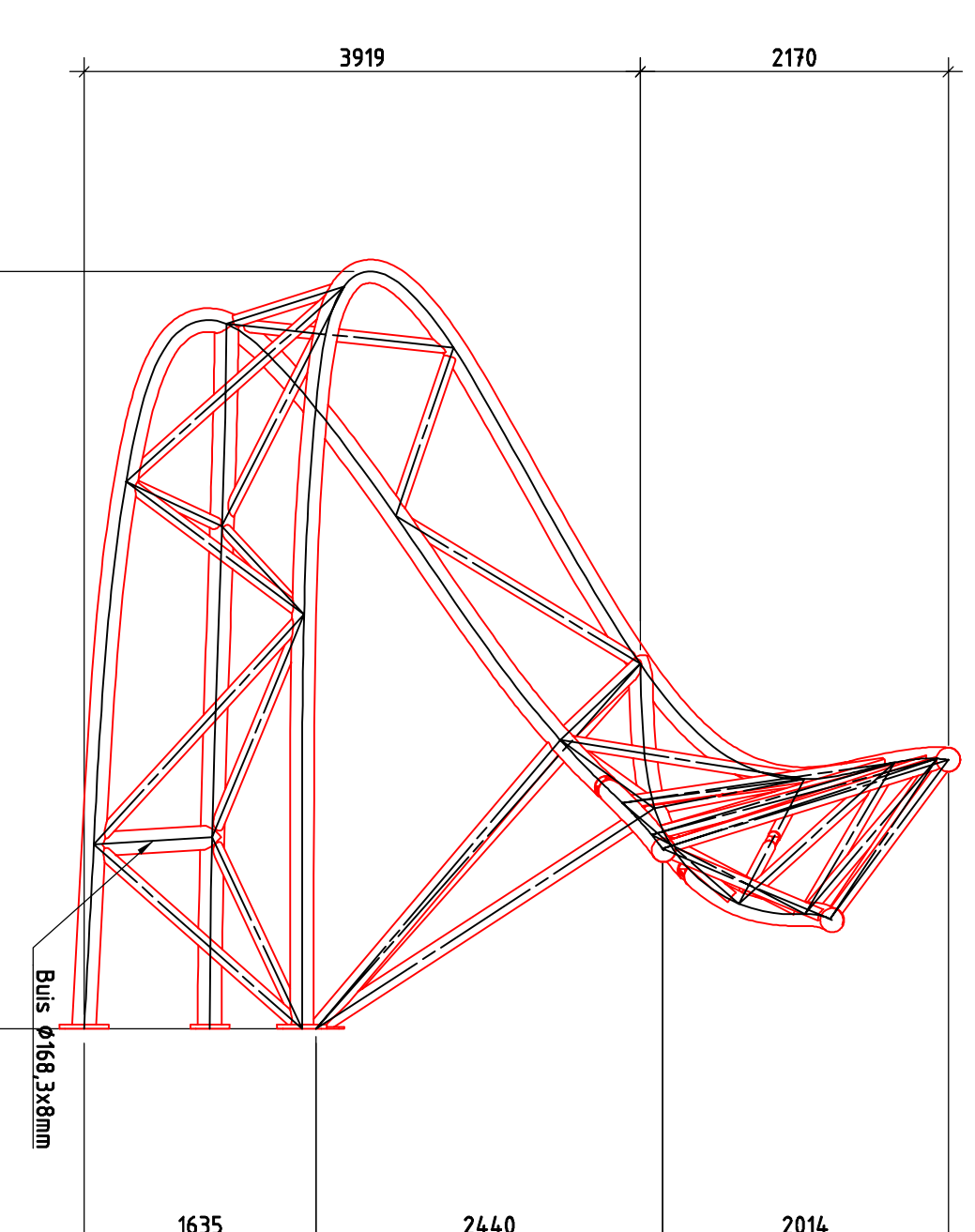
Aanzicht AA Schaal 1:50
