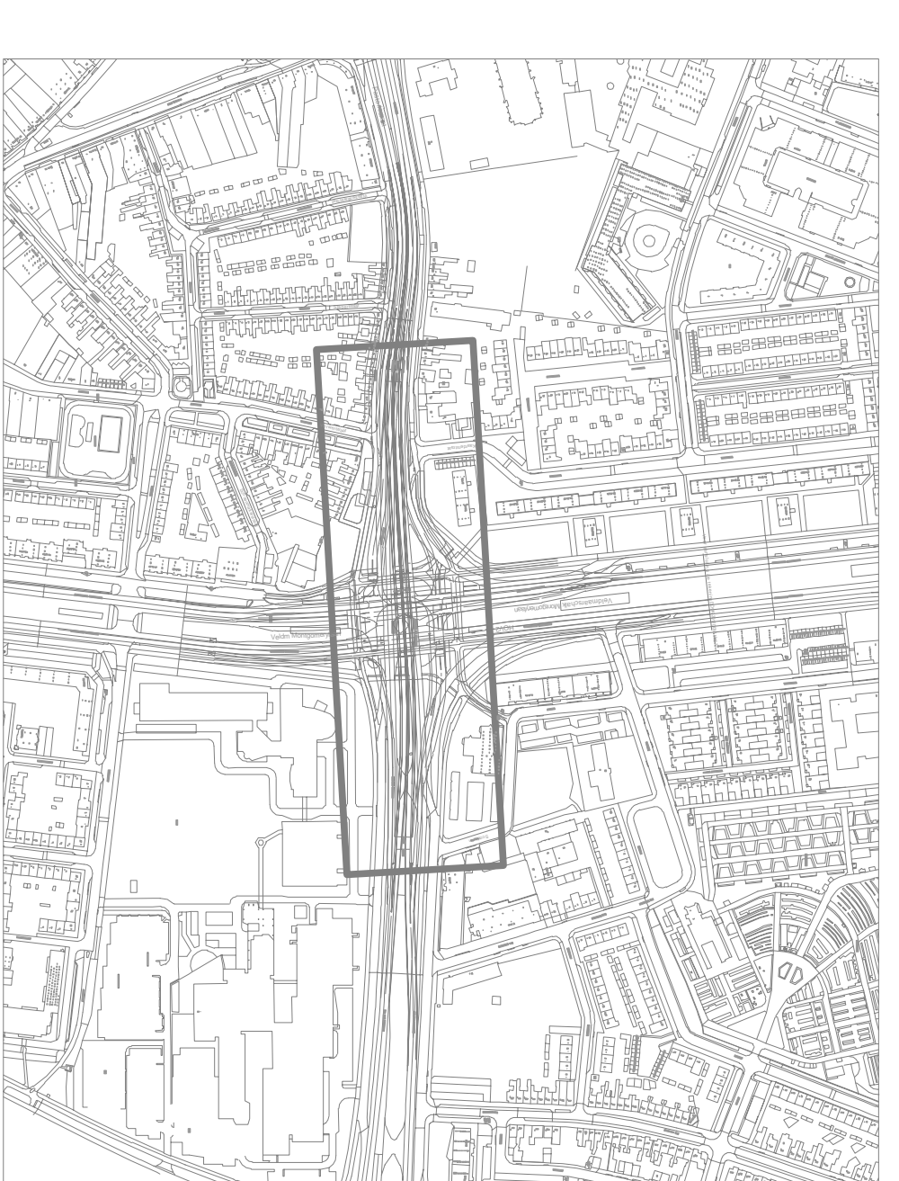
Situatie Schaal 1:1000
