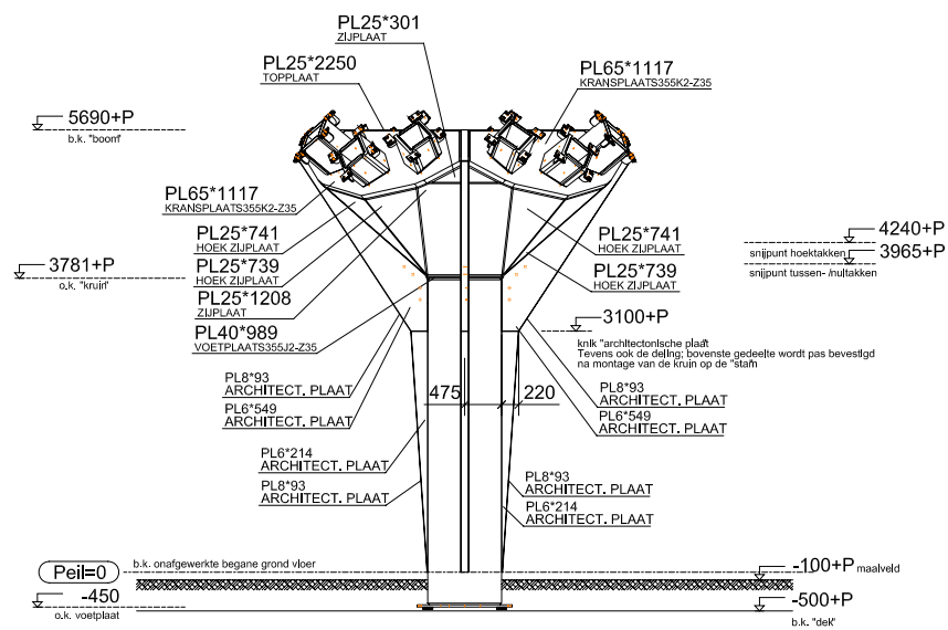
Doorsnede A - A
