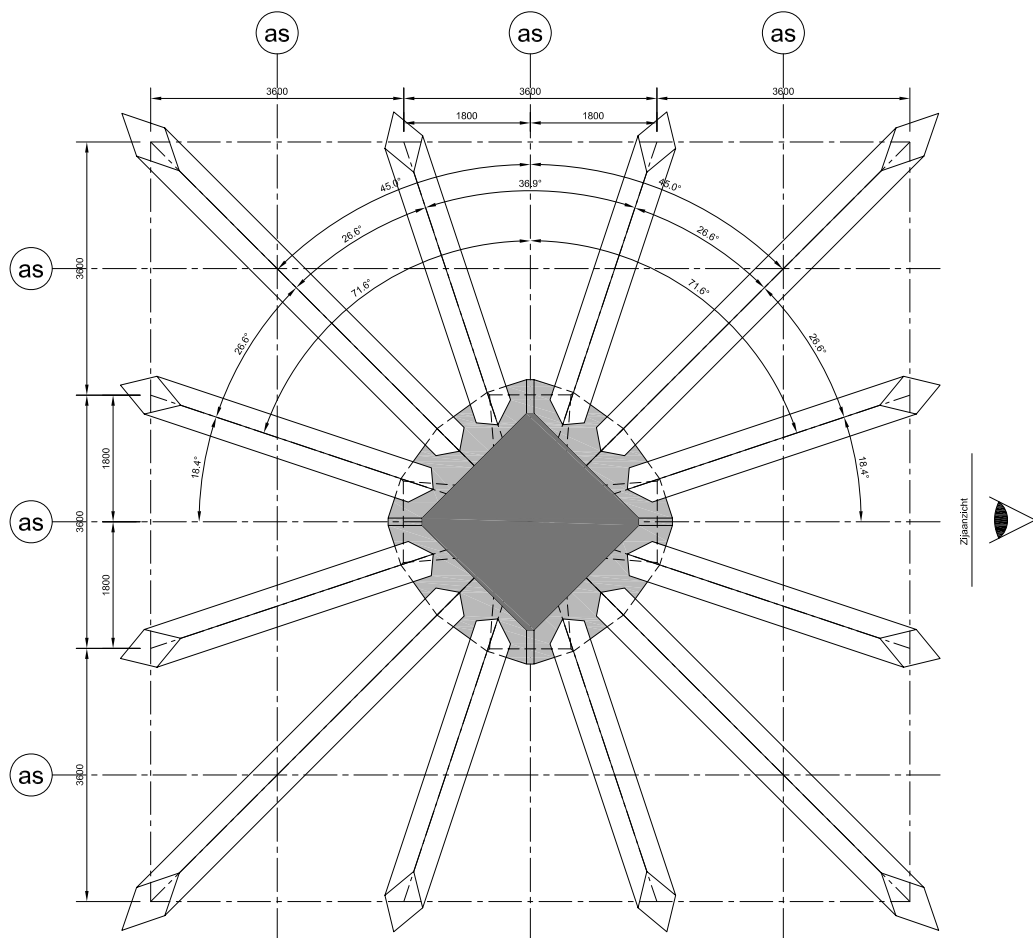
BOVENAANZICHT Maatvoering hoeken
