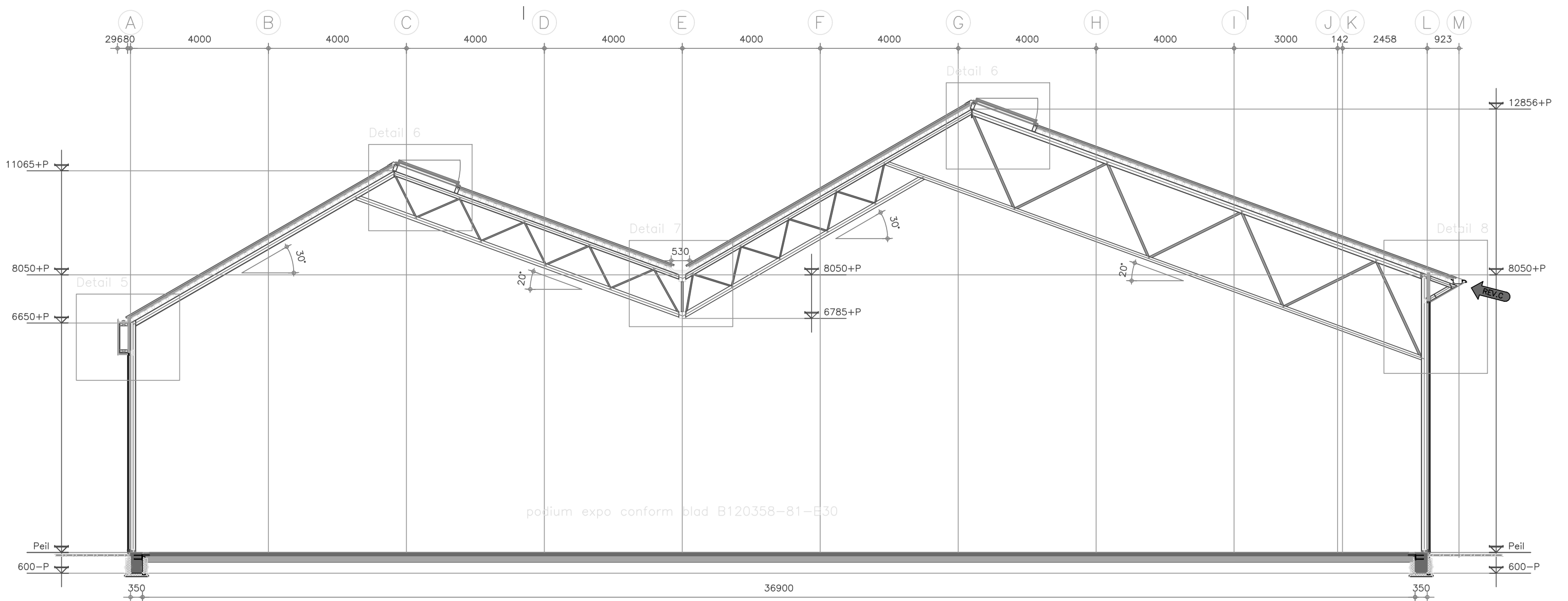
Doorsnede A-A
