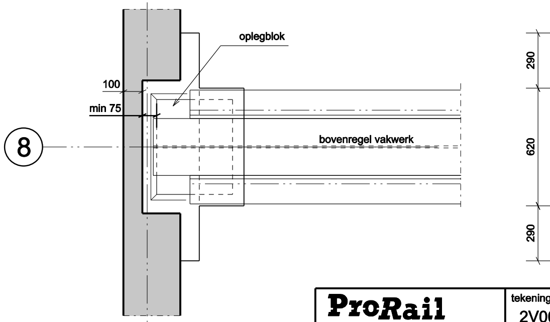
Doorsnede C Oplegging vakwerklijger op woningen tpv as 8, 10,26,30
