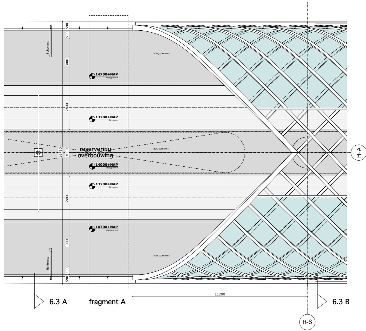
plattegrond
