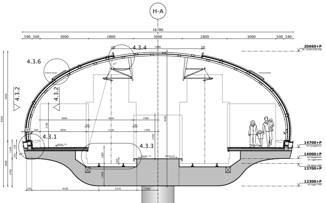
dwarsdoorsnede 6.3 B
