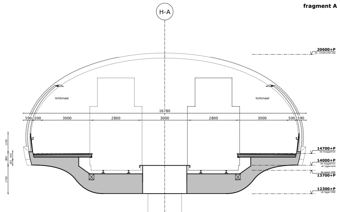
dwarsdoorsnede 6.3 A
