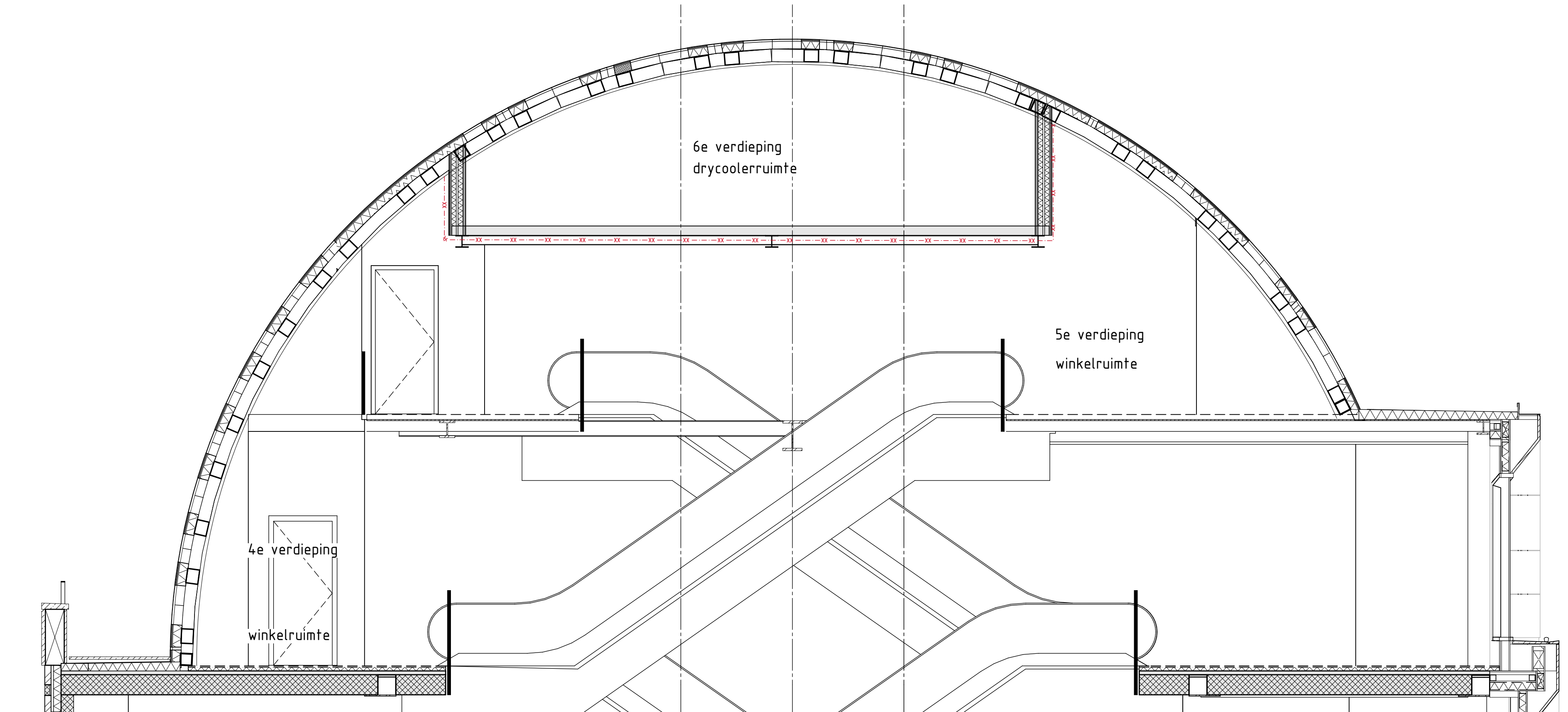
Doorsnede E-E
