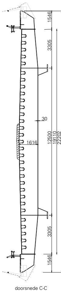
doorsnede C-C
