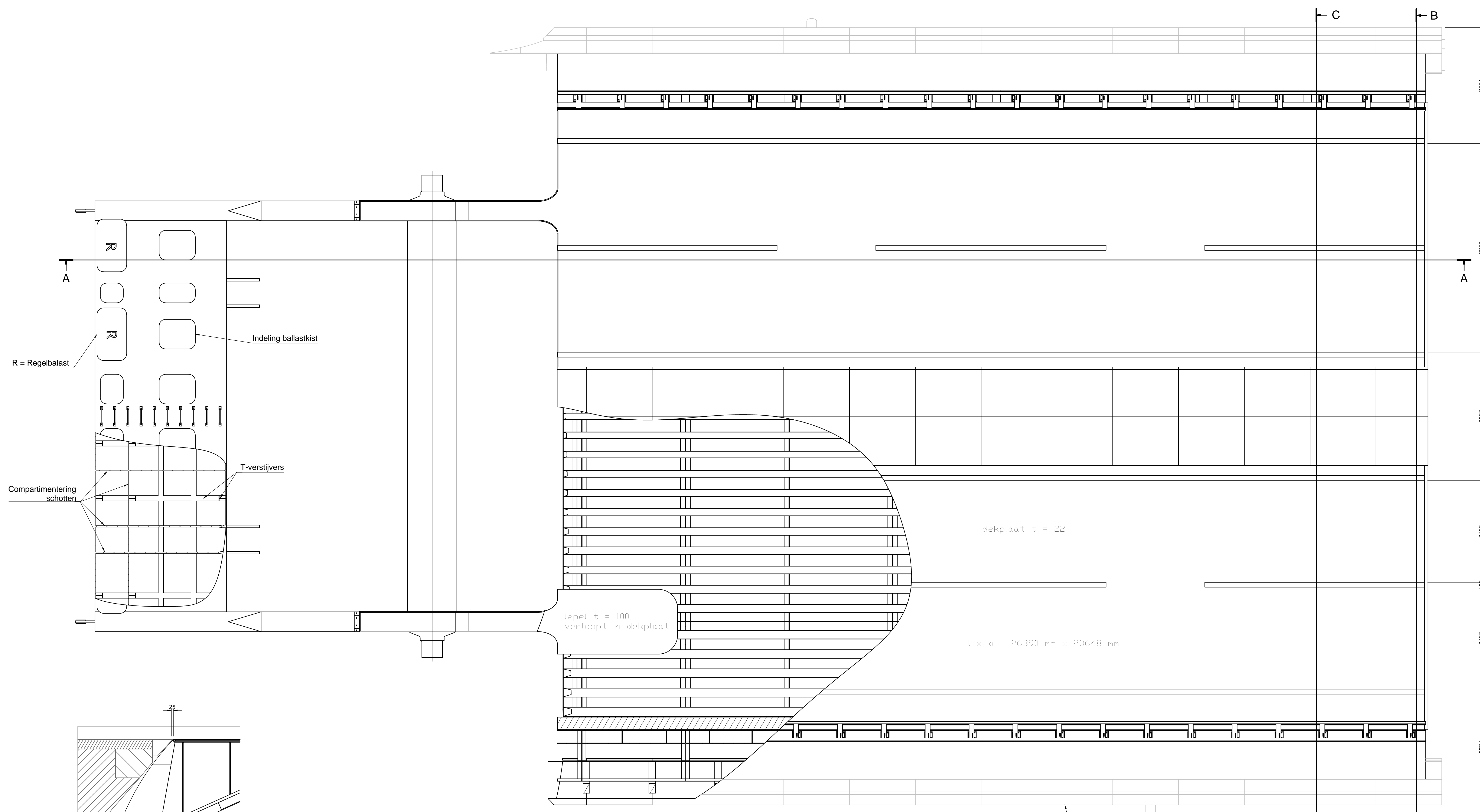
Bovenaanzicht brugval
