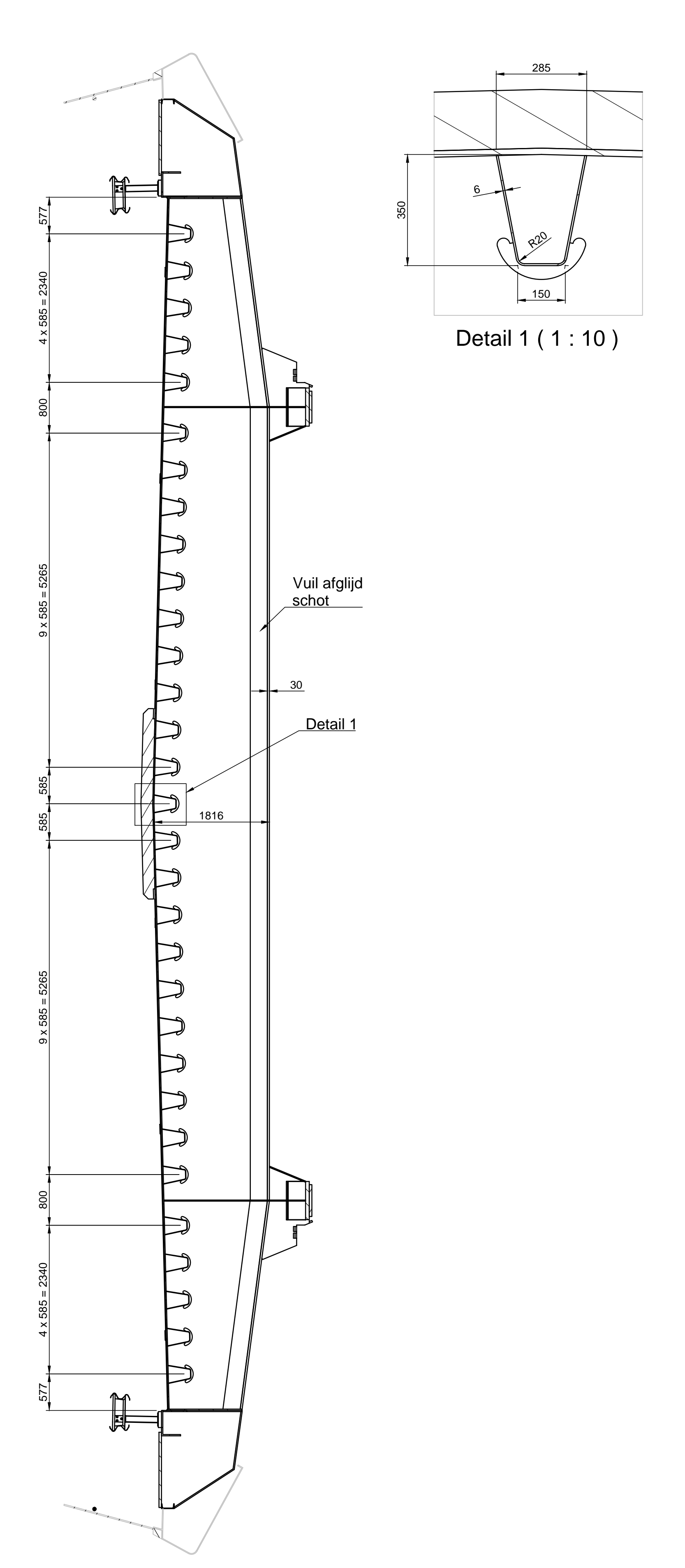
Doorsnede B-B (1:50)
