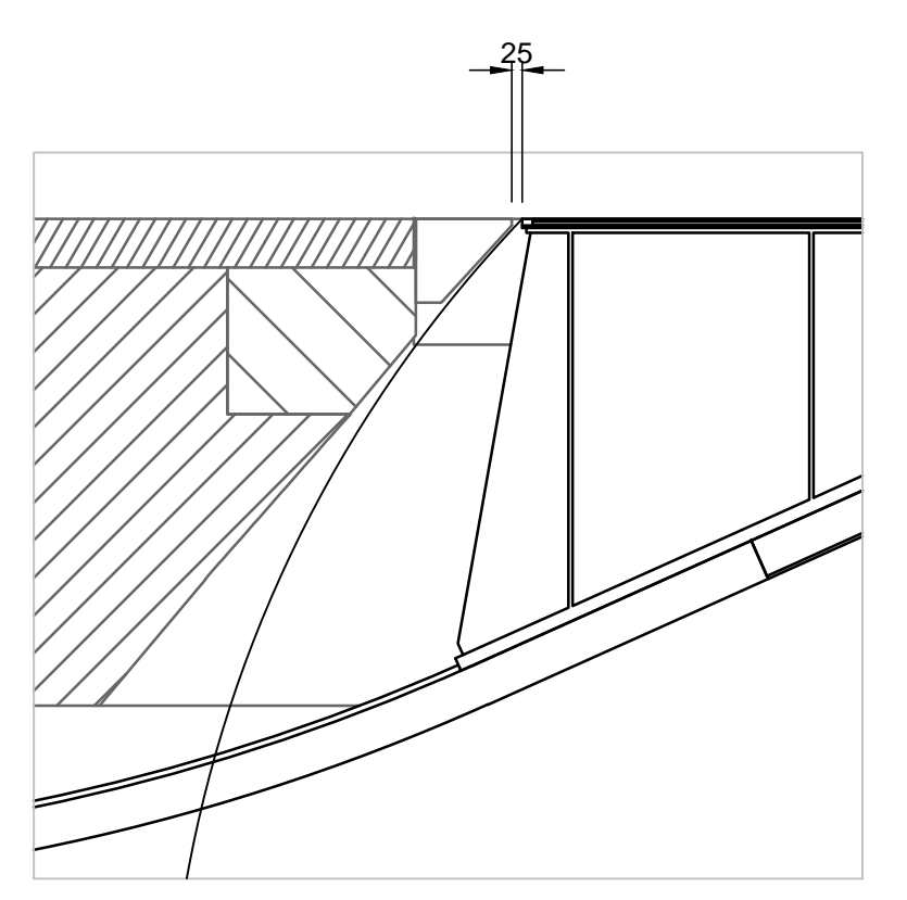
Detail Voeg Sleufopbouw
