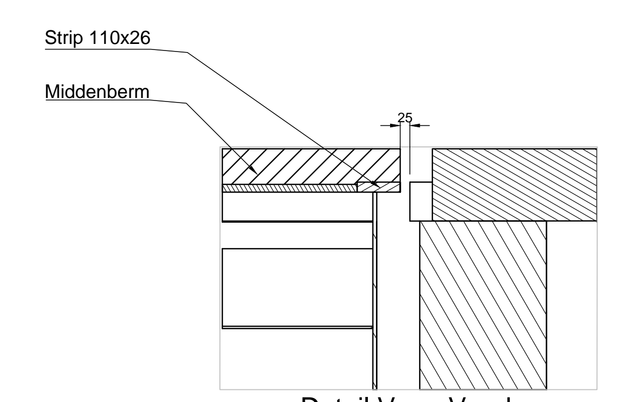
Detail Voeg Voorhar
